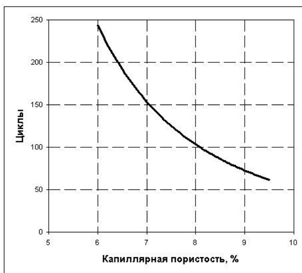
Рис. 5.6. Зависимость морозостойкости бетона от капиллярной пористости
