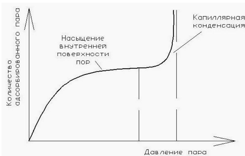
Рис. 5.5. Изотерма адсорбции (относительная влажность воздуха при постоянной температуре)
