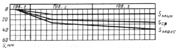
График развития перемещений
