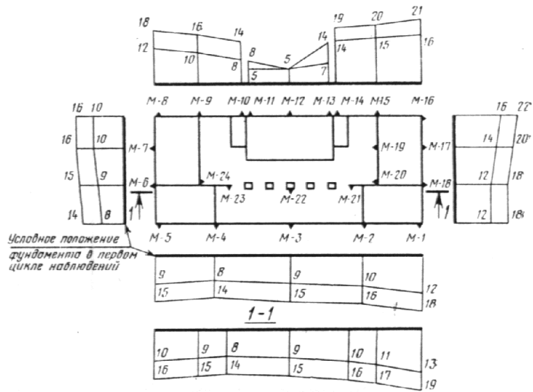
График давления на основание фундамента
