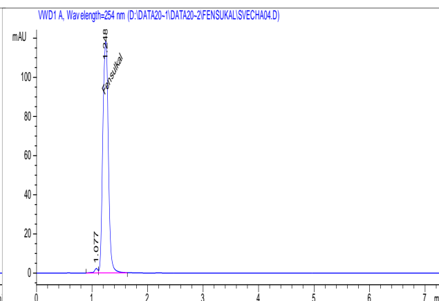
Расм 6. Фенсулкалининг текширилаётган намунаси хроматограммаси
