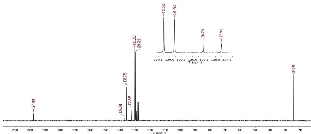
Рисунок 4. ^{13}\text{C} ЯМР спектр бензкетозона
