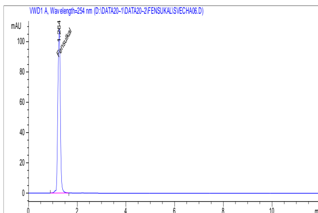
Расм 5. Фенсулкали ишчи стандарт намунасининг хроматограммаси
