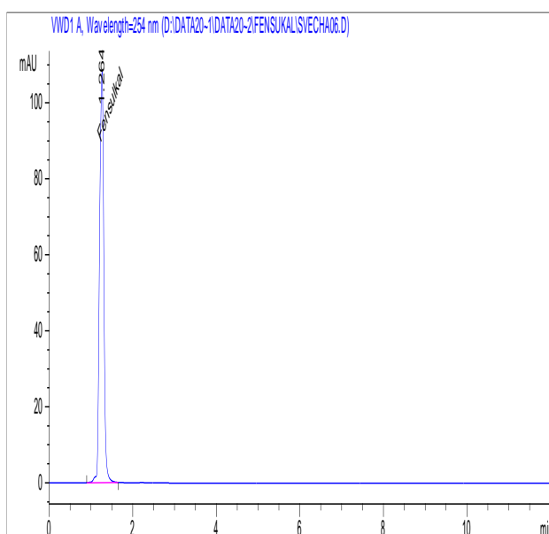
Рисунок 5. Хроматограмма рабочего стандартного образца (PCO) фенсулкала
