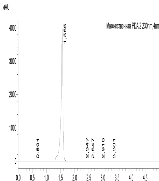
Рисунок 8. Хроматограмма испытуемого образца бензкетозона
