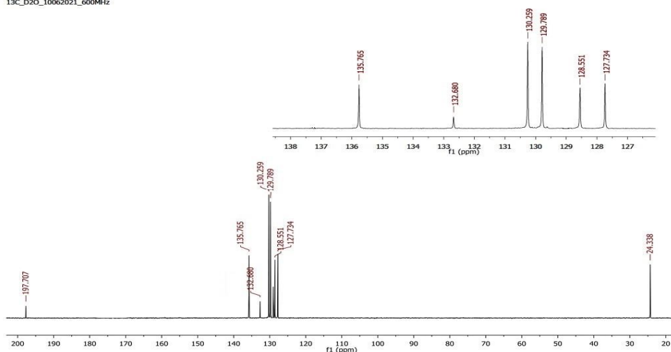
Рисунок 3. ^{13}\text{C} ЯМР спектр фенсулкала
