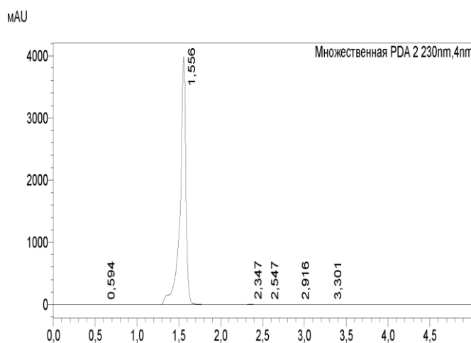
Расм 8. Бензкетозоннинг текширилаётган намунаси хроматограммаси
