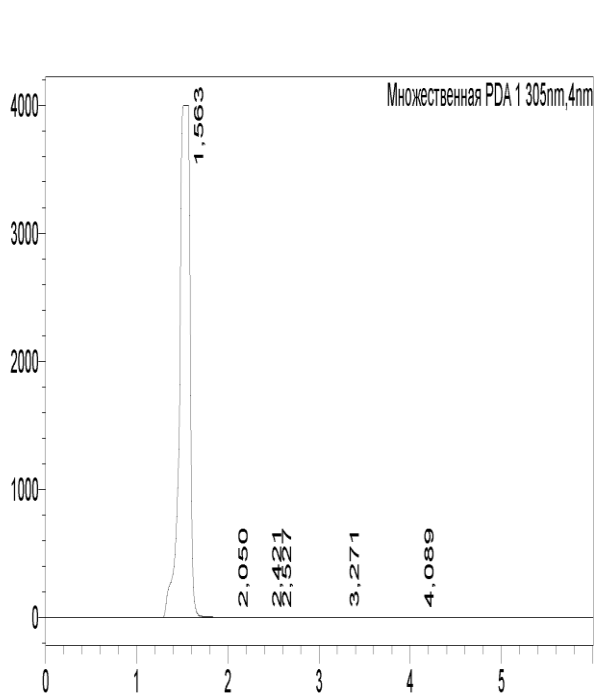
Рисунок 7. Хроматограмма РСО бензкетозона
