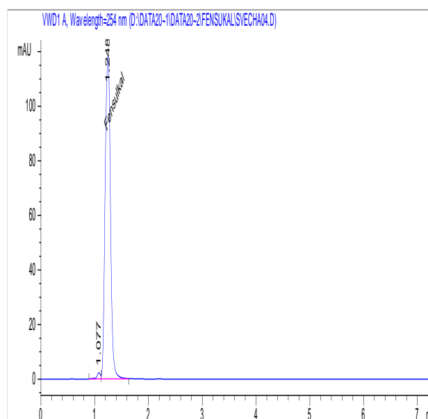
Рисунок 6. Хроматограмма испытуемого образца фенсулкала
