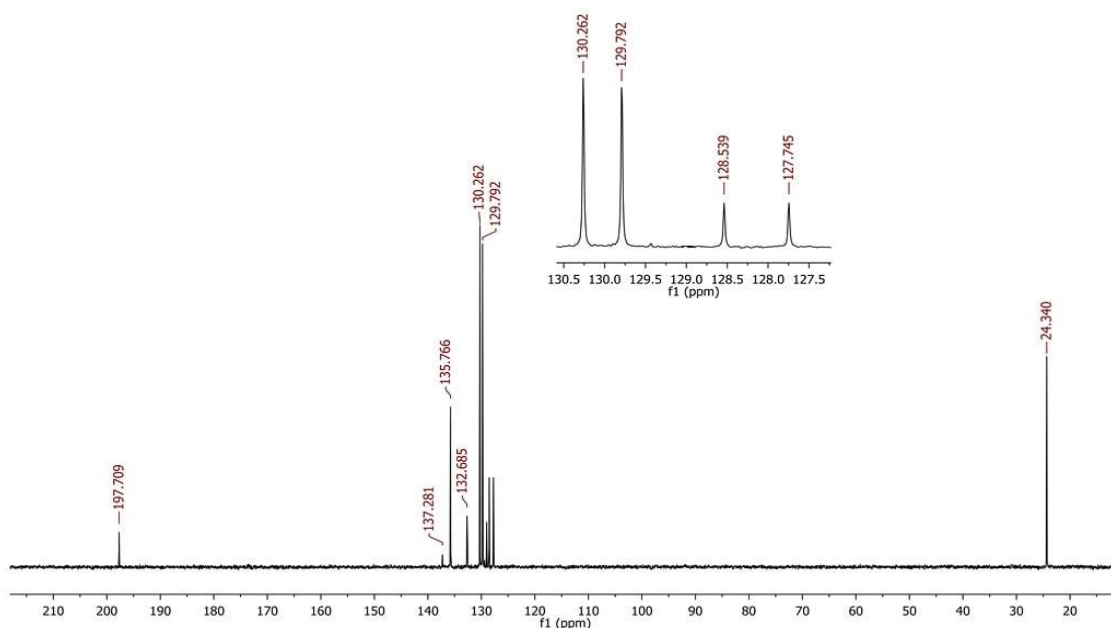
Расм 4. Бензкетозоннинг ЯМР ^{13}\text{C} спектрлари
