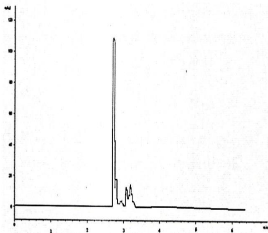
Рисунок 8. Хроматограмма испытуемого образца облепихового масла.
