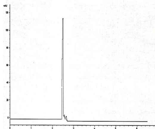
Рисунок 9. Хроматограмма стандартного образца \beta -каротина.
