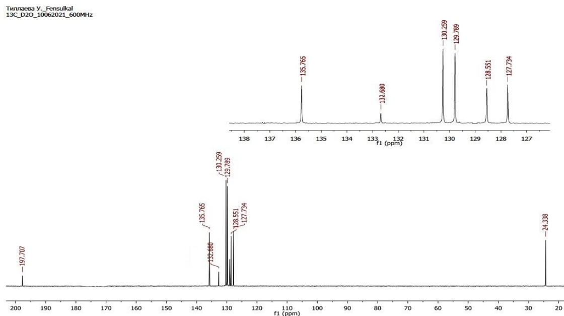
Расм 3. Фенсулгалнинг ЯМР ^{13}\text{C} спектрлари
