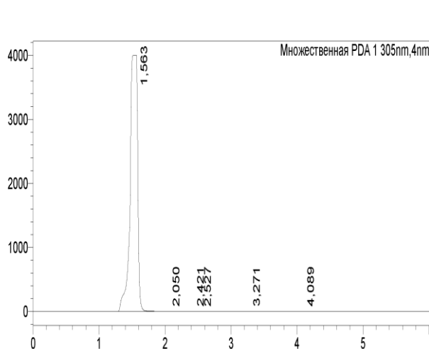
Расм 7. Бензкетозон ишчи стандарт намунасининг хроматограммаси
