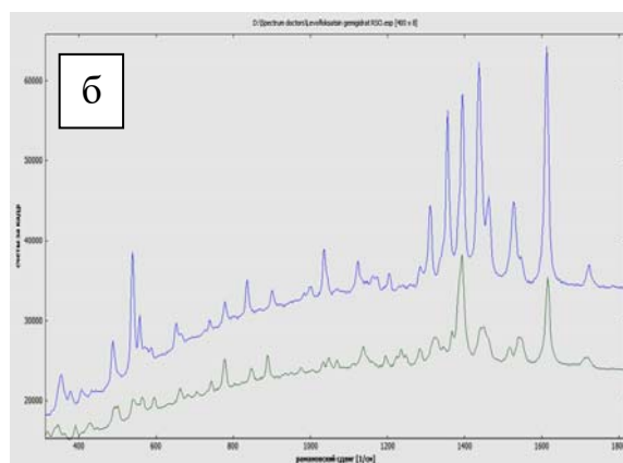
б - 90 ° С ҳароратда қуритилган левофлоксацин гемигидрат Раман спектри
