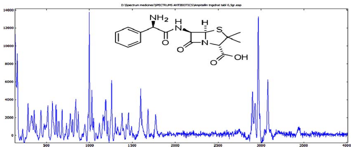
3 -расм. Ампициллин тригидрат таблеткасининг Раман спектри
