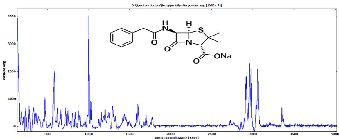
Рис.2. Рамановский спектр порошки бензилпенициллина натрия
