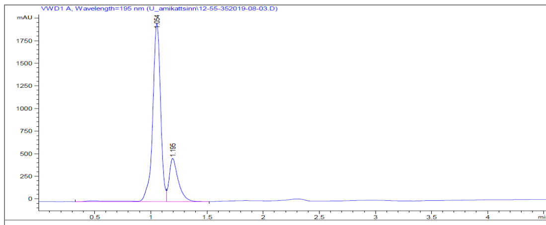
Рис.9. Хроматограмма стандартного образца амикацина сульфата
