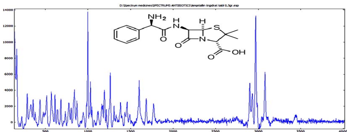
Рис.3. Рамановский спектр таблеток ампициллина тригидрата
