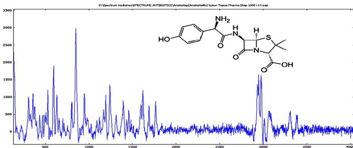
4-расм. Амоксициллин кукунининг Раман спектри
