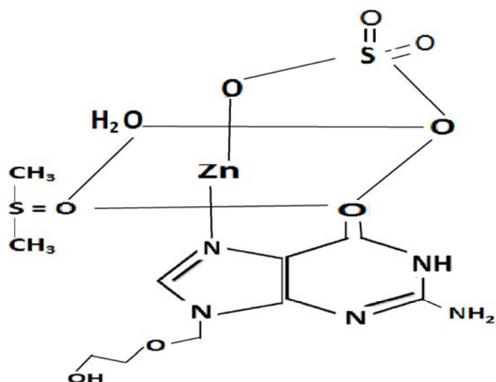
Рис.1. Схематическое строение комплекса Zn(Asuc)(DMSO)SO_4 \cdot H_2O
