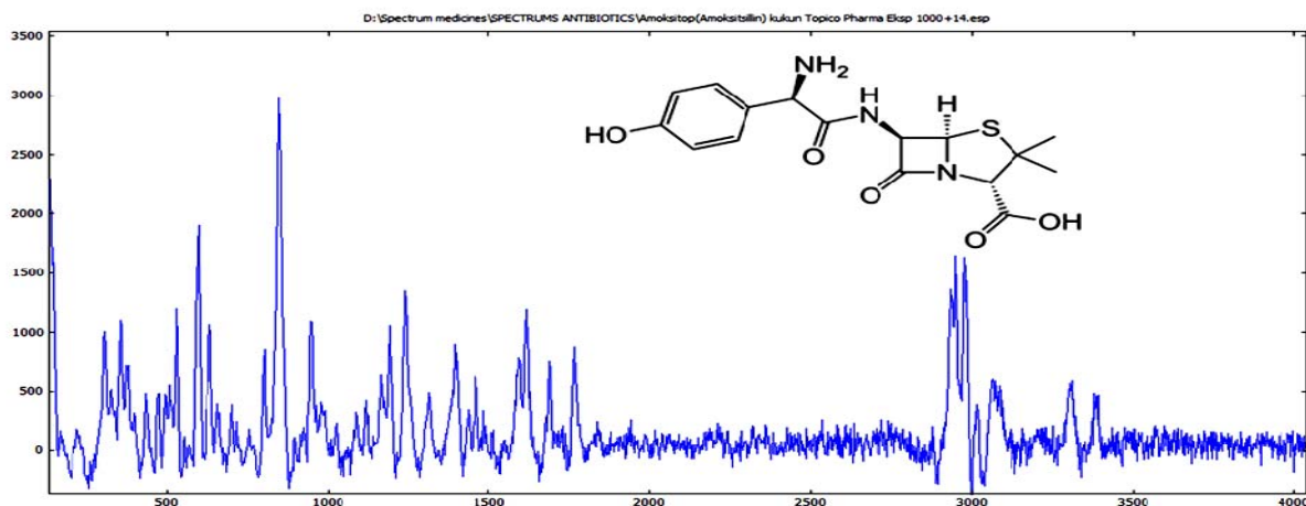
Рис.4. Рамановский спектр порошки амоксициллина
