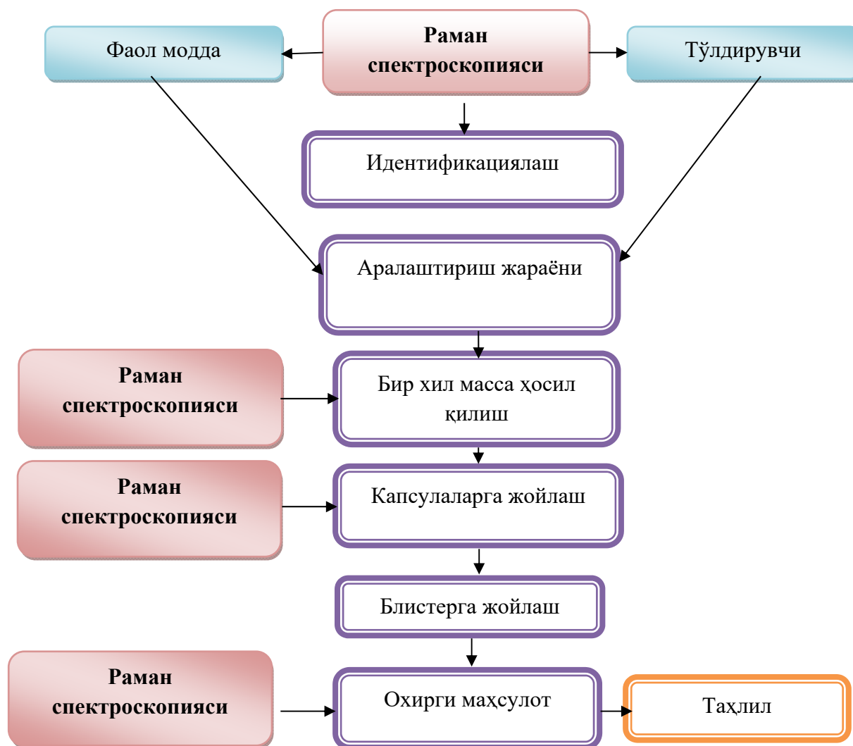
8-расм. Раман спектроскопия усули имкониятлари асосида назорат қилиш босқичлари
