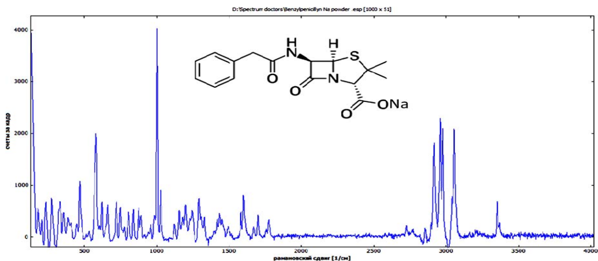
2-расм. Бензилпенициллин натрий кукунининг Раман спектри
