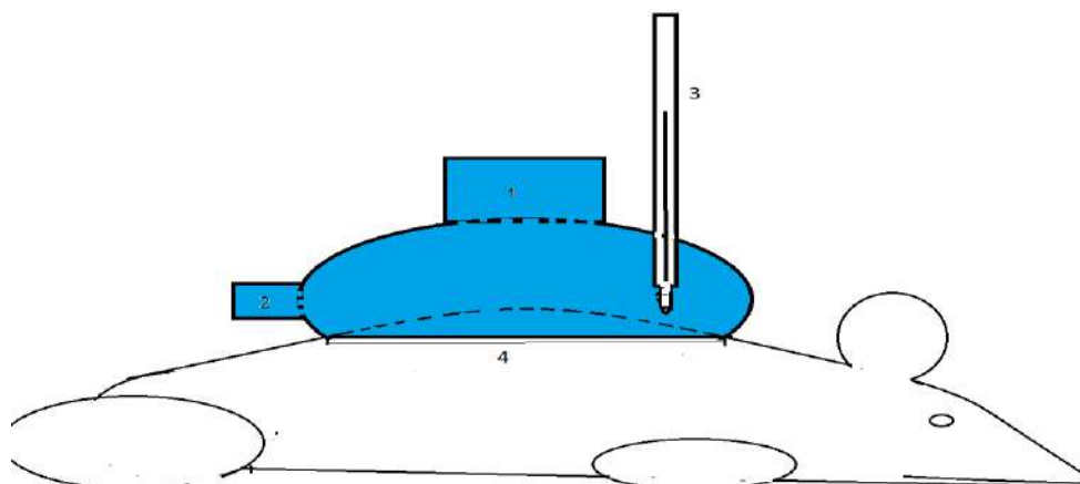
Рис. 3. Устройство для моделирования ожоговой раны у лабораторного животного. Камера устройства: 1 - отверстие для введения горячей жидкости; 2 – сливное отверстие с трубкой; 3 – термометр; 4 – отверстие для контакта с кожей, покрытое тонкой резиновой пленкой.
