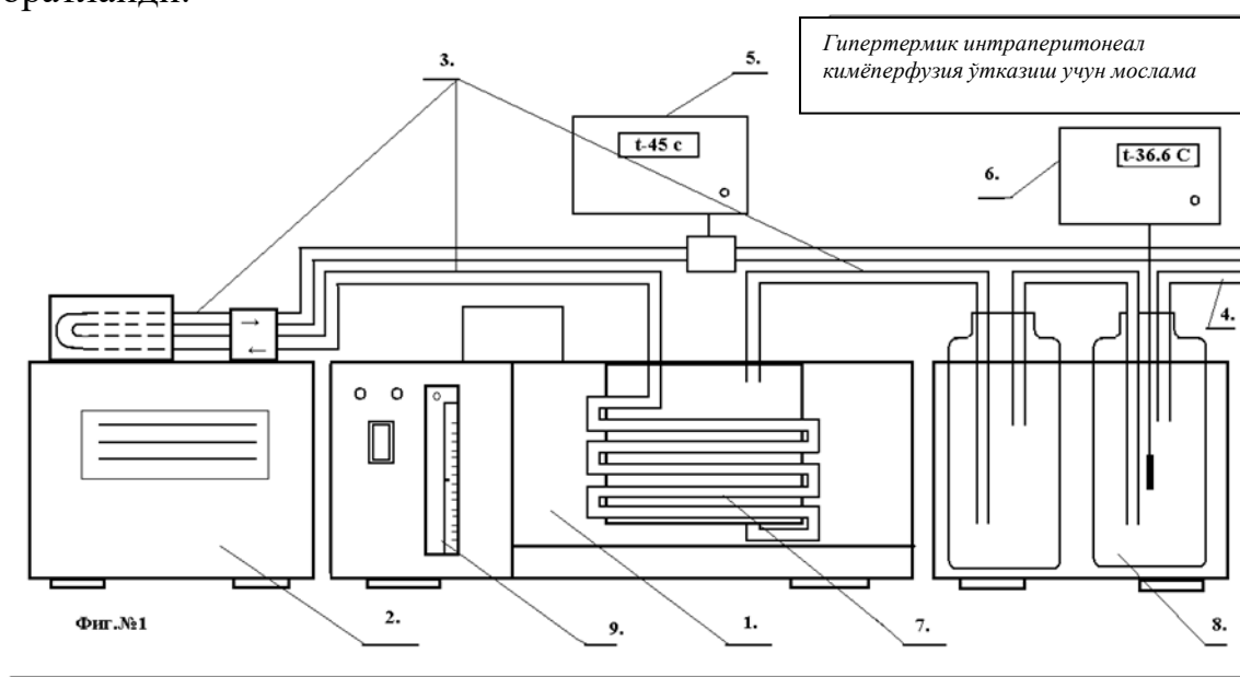
2-расм. Гипертермик интраперитонеал кимё перфузия ўтказиш учун қурилманинг схематик кўриниши
