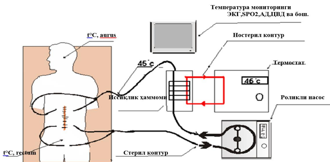
1-расм. Гипертермик интраперитонеал кимё перфузия ўтказилиш тизими
