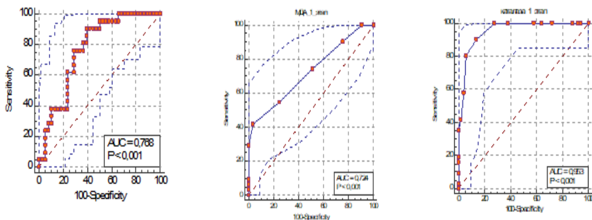
Рис. 3. ROC-кривая для креатинина, МДА, каталазы на 1-м этапе (AUC).
