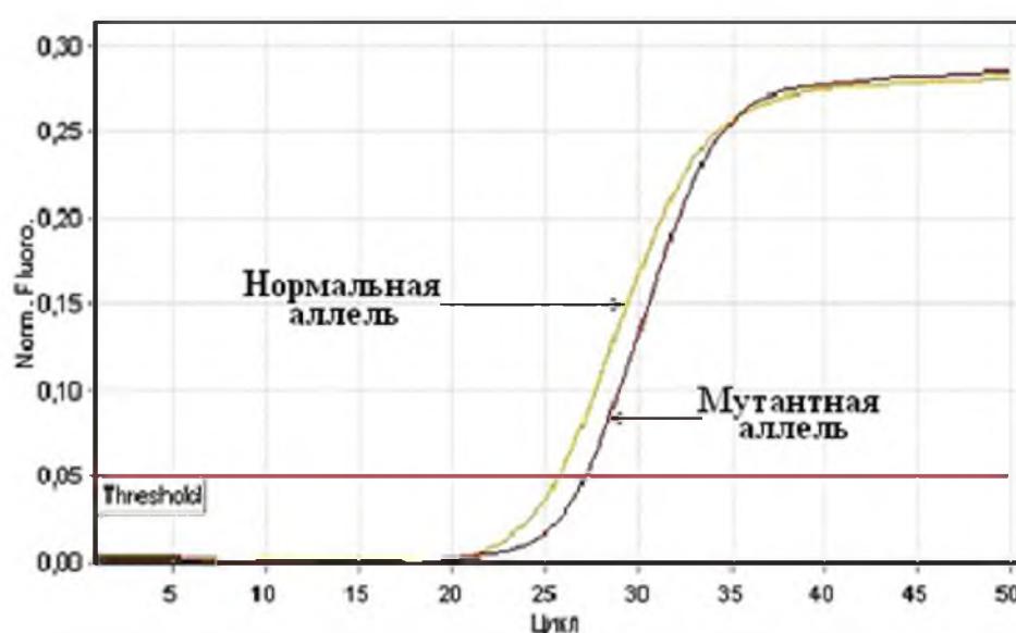
Рис. 11. Гетерозиготная форма мутации гена MDR1 3435 T/C
