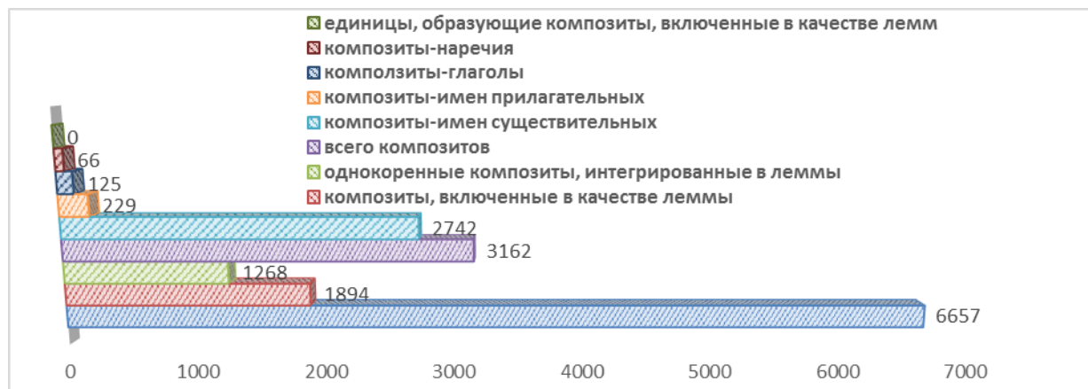
Рис. 2. Статистический анализ лемм, включенных в словарь Я.Беньяминова, С.Саидова (1991)
