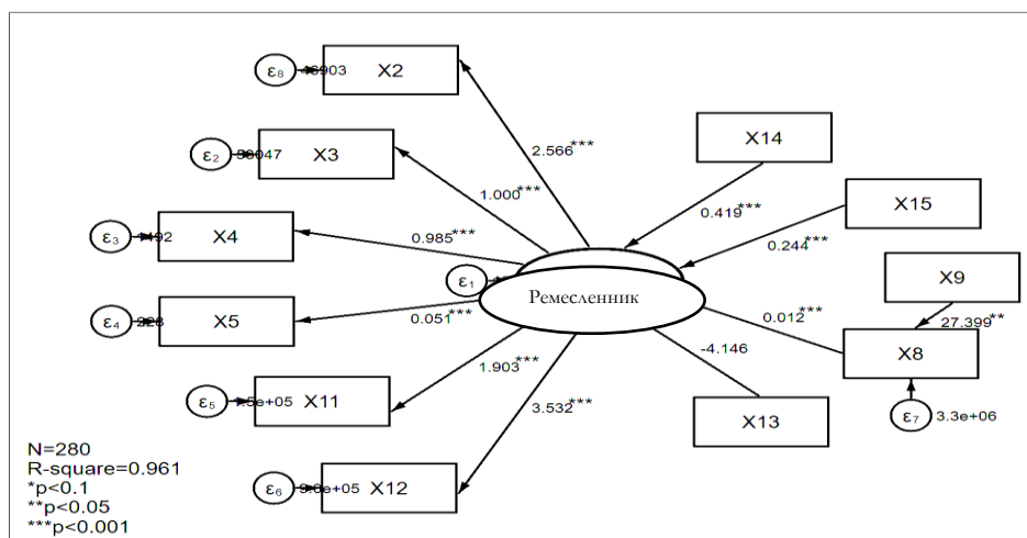
Рис.8. Иллюстрированный вид модели SEM+SEM-Path+LCA 37
