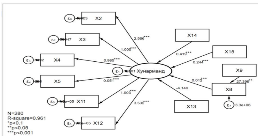
8-расм. SEM+SEM-Path+LCA моделининг тасвирий кўриниши 37
