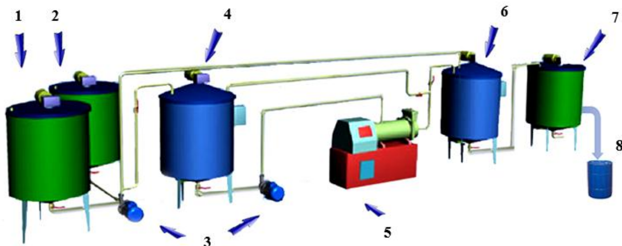
Рис.6 Схема технологии получения новых составов эффективных жаропрочных лакокрасочных материалов:
