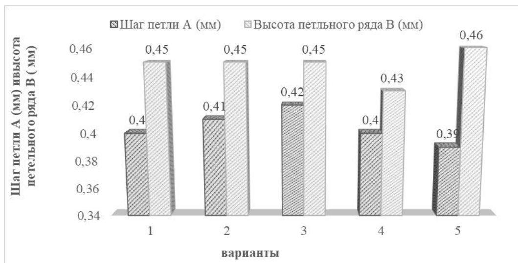
2-рисунок. Диаграмма изменения шага петли А (мм) и высоты петельного ряда В (мм).
