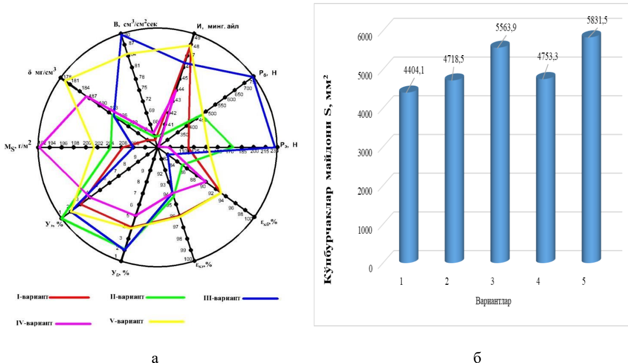
12-рasm. Трикотаж тўқимасининг сифат кўрсаткичларини комплекс баҳолаш диаграммаси ва гистограммаси
