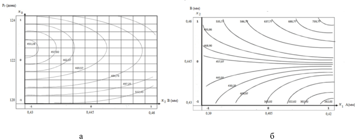
9-расм. Трикотаж тўқимасининг узиш кучи (бўйи бўйича) кўрсаткичларининг қийматлари
