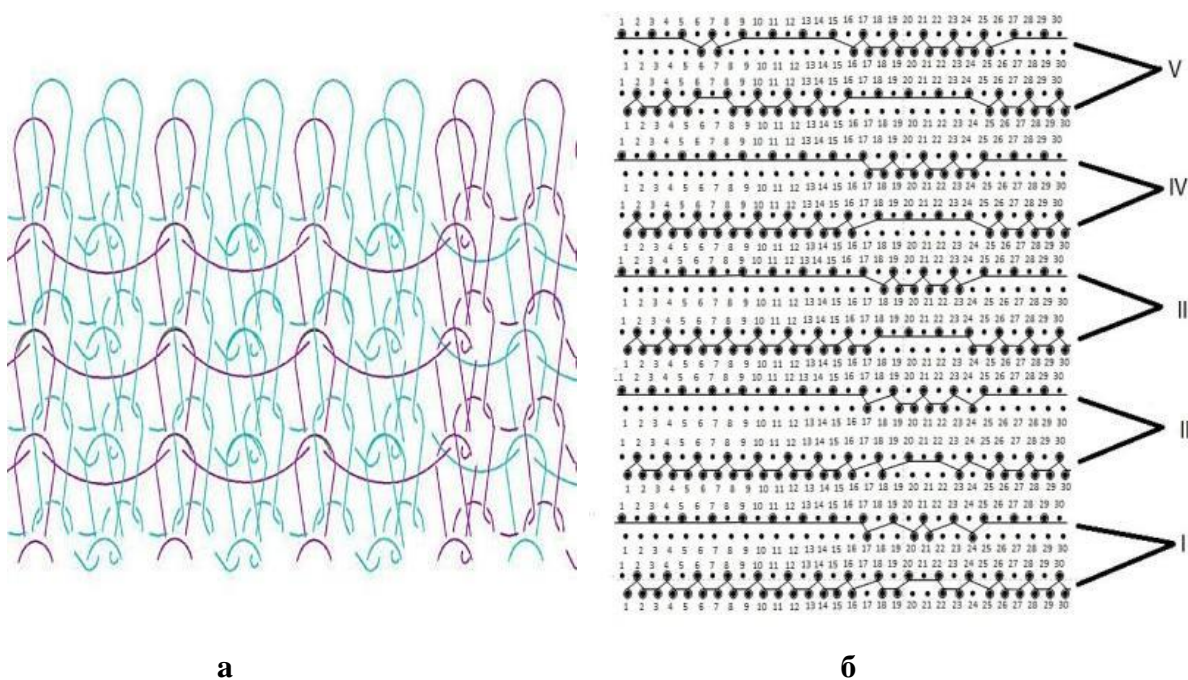
1-рasm. Турли хомашёлардан олинган трикотаж тўқималарининг тузилиши (а) ва график ёзуви (б).
