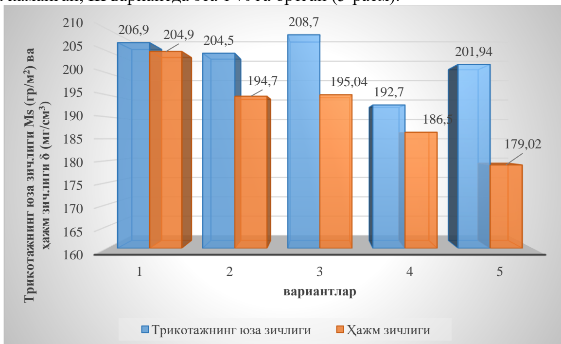
5-расм. Трикотаж тўқимасининг юза зичлиги ва ҳажм зичлигини ўзгариши гистограммаси.
