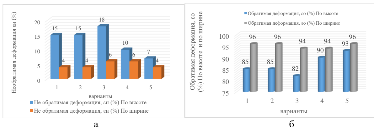
Рисунок 8. Гистограмма необратимой и обратимой деформации трикотажных полотен, полученных из разного сырья.
