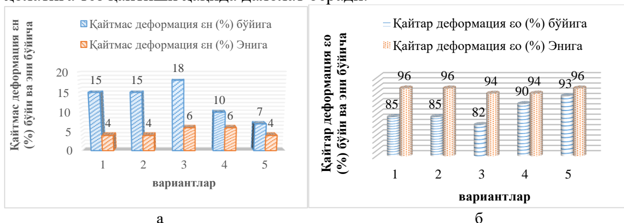
8-расм. Турли хомашёлардан олинган трикотаж тўқималарининг қайтмас ва қайтар деформациясини ўзгариши гистограммаси
