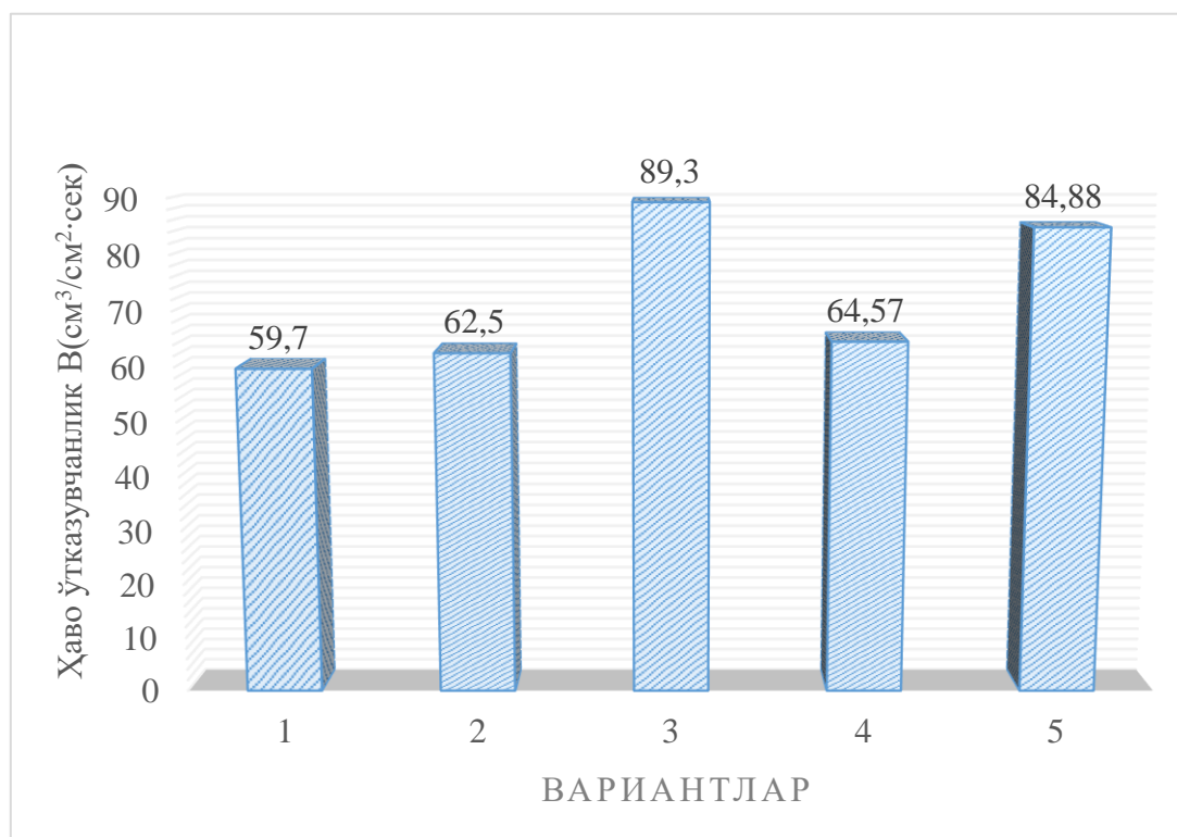
6-расм. Турли хомашёлардан олинган трикотаж тўқимасининг хаво ўтказувчанлик ўзгариши гистограммаси.
