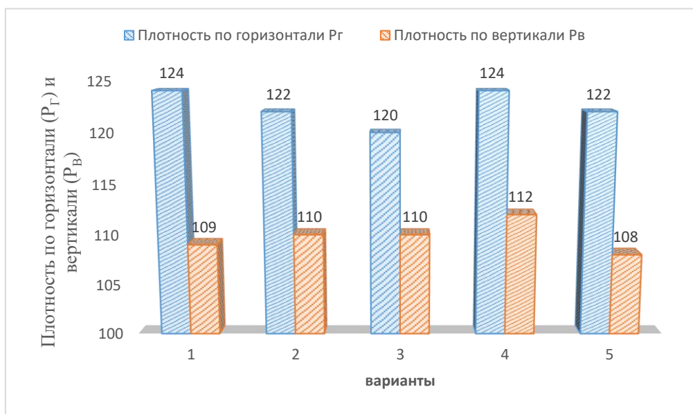
4-рисунок. Диаграмма изменения плотности по горизонтали (P г ) вертикали (P в )
