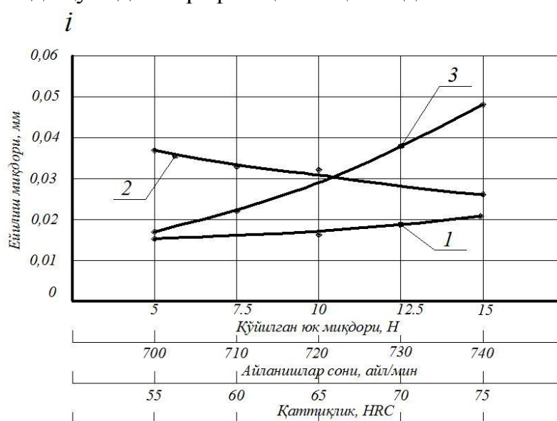
2-расм. Колосникларни унга таъсир этадиган босим кучи(1), материалнинг қаттиқлиги(2) ва арранинг айланиш тезлиги(3)га боғлиқ равишда ейилиш графиги.
