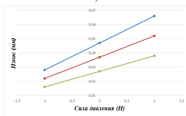
Рис.4. а) средняя скорость износа образцов; б) график изменения показателя износа ( y ) в зависимости от твердости наплавленного покрытия ( HRA ); в) график изменения показателя износа ( y ) в зависимости от числа оборотов ( n ) пыльного полотна; г) график изменения показателя износа ( y ) в зависимости от силы давления ( P )
