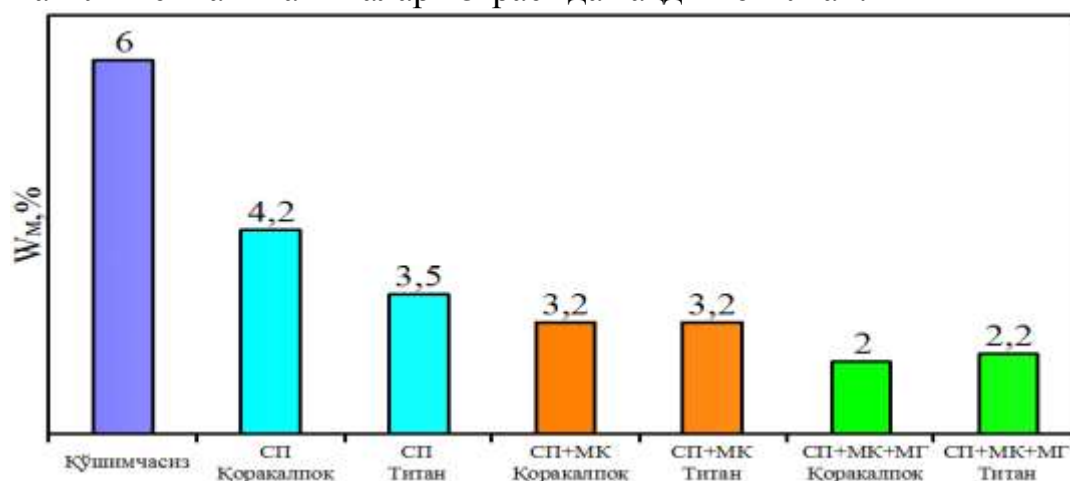
5-расм. 28 кунлик модификацияланган бетонларнинг сув шимувчанлиги хусусиятига оид синовлар натижалари.
