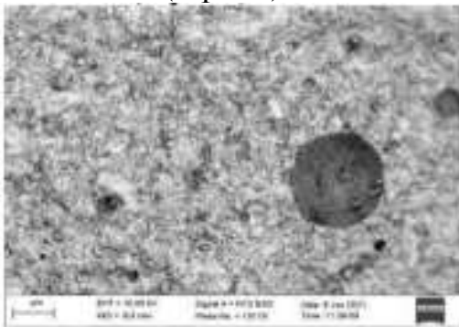
Қўшимчасиз цемент тошининг микротузилиши ва таркиби.
