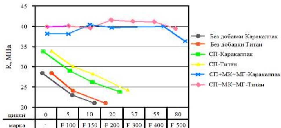
Рис. 6. Результаты испытания образцов модифицированных бетонов на морозостойкость
