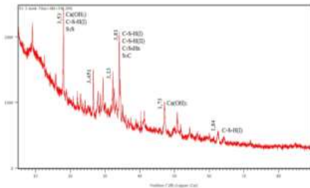
Цемент тоши СП+ МК+МГ рентгенфазавий таҳлили маълумоти
