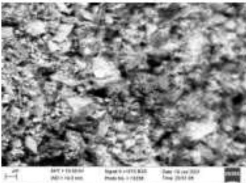
СП+МК+МГ цемент тошининг микротузилиши ва таркиби.
