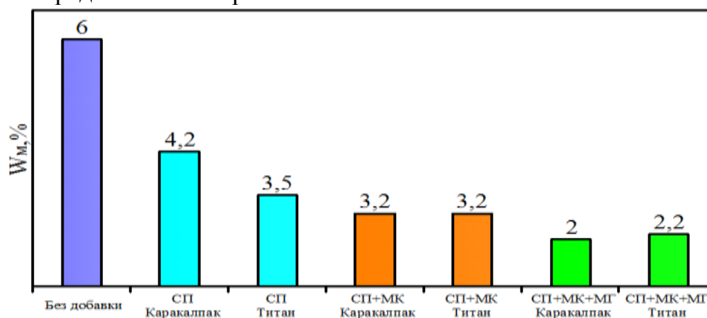
Рис. 5. Результаты испытания водопоглощения модифицированных бетонов в возрасте 28 суток.
