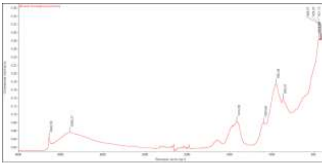
Қўшимчасиз 28 кунлик цемент тоши ИҚ таҳлили маълумоти
