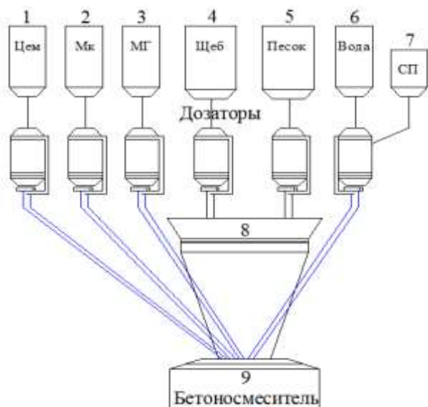
7-расм. Модификацияловчи қўшимчалар мажмуига эга бўлган бетон олишнинг технологик схемаси
