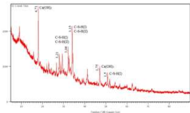
Кўшимчасиз цемент тошининг рентген-фазавий таҳлили маълумоти
