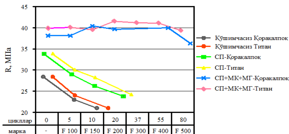
6 -расм. Модификацияланган бетонлар намуналарининг совуққа чидамлилиққа синаш натижалари
