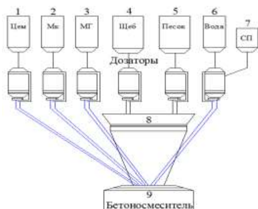
Рис. 7. Технологическая схема получения бетона с комплексом модифицирующих добавок 1-7 - бункер составляющих композиционную бетонную смесь; 8 - распределитель песка и щебня; 9 - бетоносмеситель.
