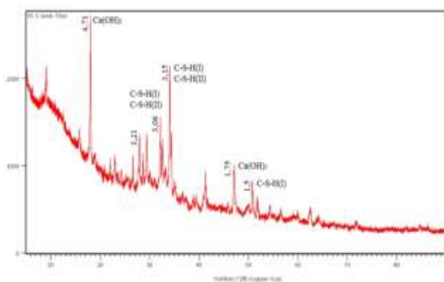
Данные рентгенофазового анализа цементного камня без добавки
