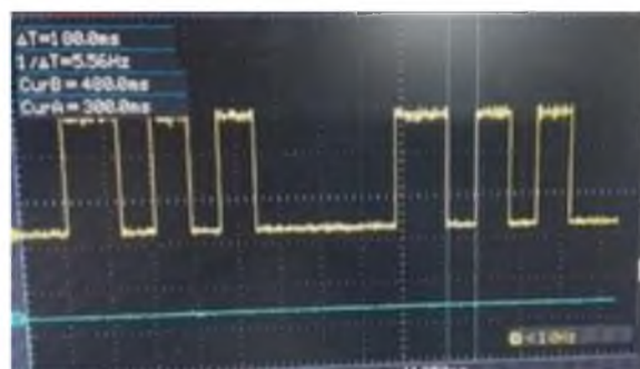
8-расм. Бирлаштирилган микроэлектрон импульс шакллантиргични осциллографлар ёрдамида текширишларини ўтказиш
