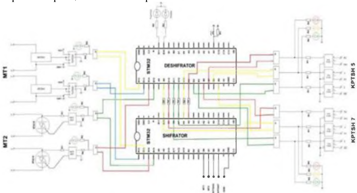
Рис. 5. Принципиальная схема интегрированного микроэлектронного формирователя импульсов
