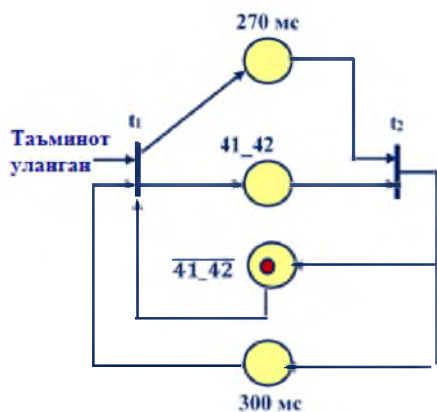
2-расм. Петри тармоғи графда МТ-1 транзиттерининг бирлаштирилган модели
