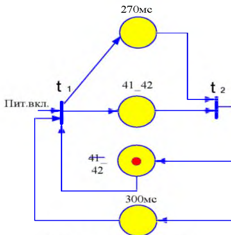
Рис. 2. Граф сети Петри обобщенной модели маятникового транзиттера МТ-1
