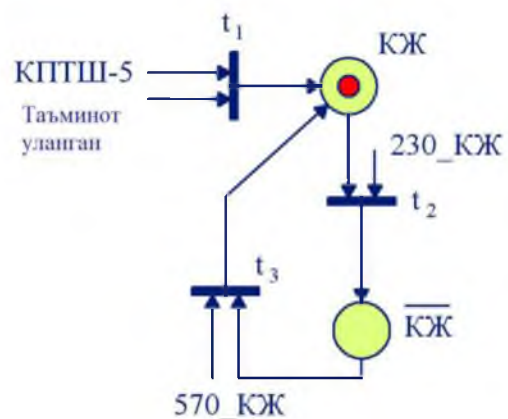
3-расм. КЖ кодини шакллантиришда Петри графи
