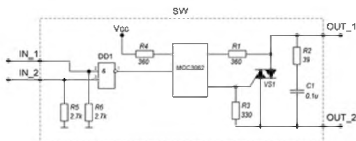
9-расм. Бирлаштирилган микроэлектрон импульс шакллантиргични ўзгарувчи токли юклага мувофиқлаштириш схемаси
