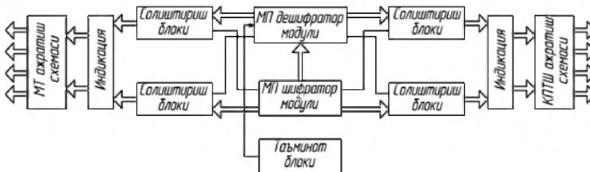
4-расм. Бирлаштирилган микроэлектрон импульс шакллантиргичнинг тузилмавий схемаси
