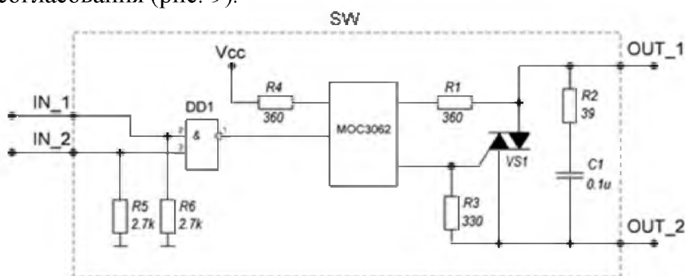
Рис. 9. Схема увязки для переменного тока
