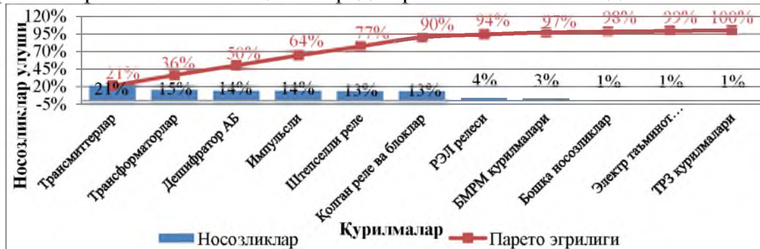
1-расм. Носозликларнинг қурилмалар бўйича тақсимланиши
