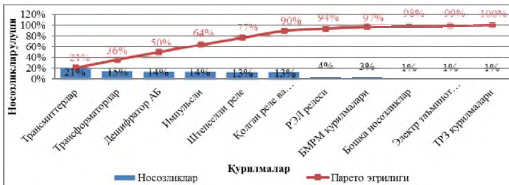
Рис.1. Распределение отказов по устройством
