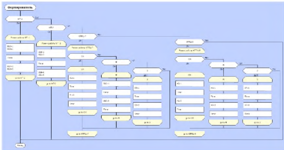
Рис. 6. Алгоритм работы шифратора интегрированного микроэлектронного формирователя импульсов.
