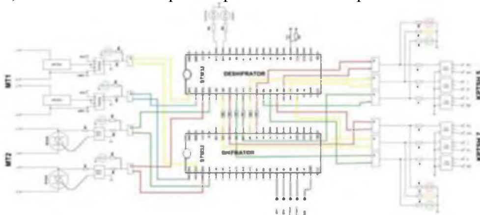
5-расм. Бирлаштирилган микроэлектрон импульс шакллантиргичнинг принцинал схемаси
