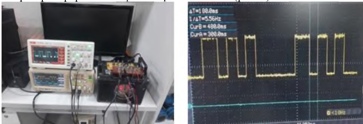
Рис. 8. Проведение испытаний интегрированного микроэлектронного формирователя импульсов с помощью осциллографов.
