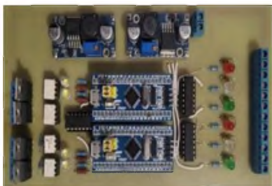
11-расм. Бирлатирилган микроэлектрон импульс шаклантиригич платаси
