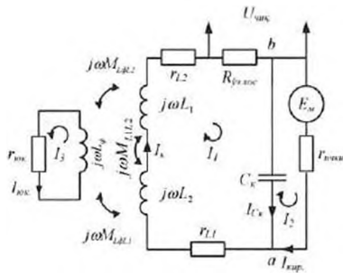
8-расм. ҒЖИД ғалтаклари ва ғилдирак гардишини ўзаро таъсирининг ўрин алмашиш эквивалент схемаси
