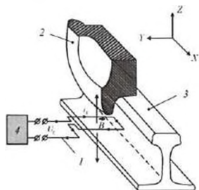
Рис.2. Конструктивное расположение чувствительного ДИКП к элементам относительно колес и рельсов
