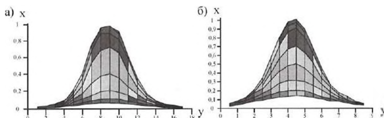
10-расм. Индуктивлик ғалтакларининг ЭММ кучланишининг марказидан (симметрия ўқи) масофа билан ўзгариши: а) ҒЖИД юзасидан 20 мм масофада; б) 6 мм масофада
