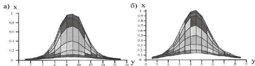
Рис.10. Изменение катушек индуктивности на расстоянии от центра напряжения ЭМП (оси симметрии): а) на расстоянии 20 мм от поверхности ДИКП; в) на расстоянии 6 мм от поверхности ДИКП
