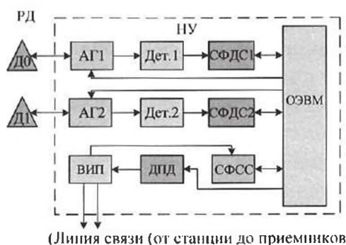
Рис.4. Функциональная схема ЭССО в счетном пункте
