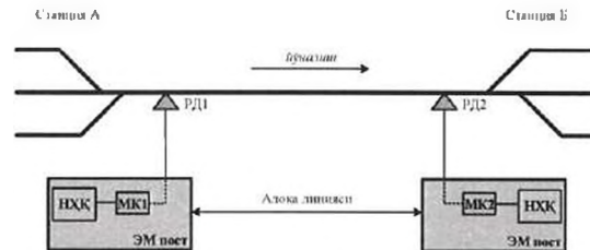
12-расм. Ярим автоматик блокировкасини умумлаштирилган тузилмавий схемаси
