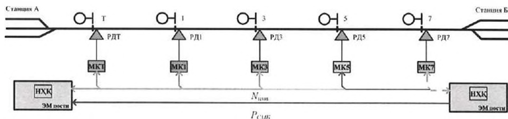
13-расм. Автоблокировка тизими учун ишлаб чиқилган назорат ва ҳисоблаш қурилмасини тузилмавий схемаси ( P_{сиг} – сигнализация, марказлаштириш ва блокировка қурилмаларига светофор кўрсаткичинини очиш учун тегишли рухсат берувчи кўрсаткич, N_{имп} импульслар сони)
