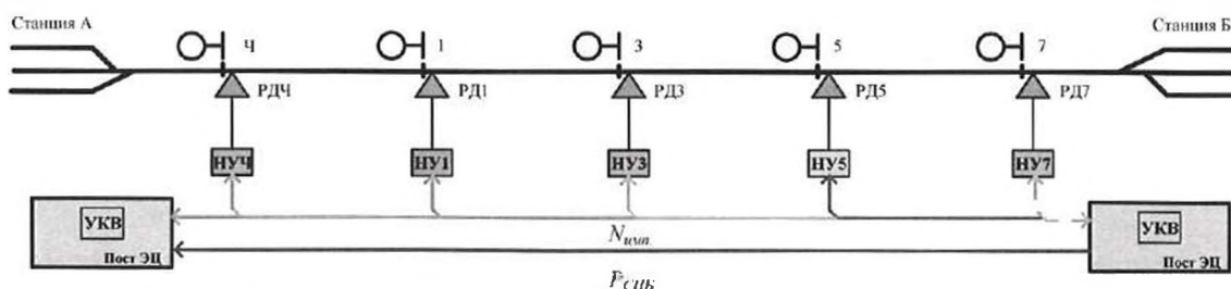
Рис.13. Структурная схема контрольно-вычислительного устройства, разработанного для системы автоблокировки ( R_{сцб} - индикатор, позволяющий устройствам сигнализации, централизации и блокировки открывать сигналы светофора, N_{имп} количество импульсов)
