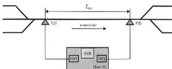
Рис.11. Обобщенная структурная схема управления участком дороги
