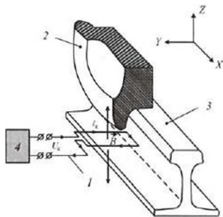
2-расм. ҒЖИД сезгир элементининг ғилдирак ва рельсга нисбатан тузилмавий жойлашини
