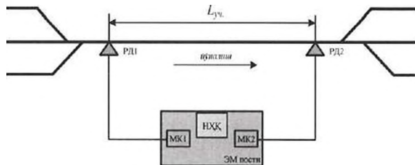
11-расм. Йўл участкаси назоратини умумлаштирилган тузилмавий схемаси
