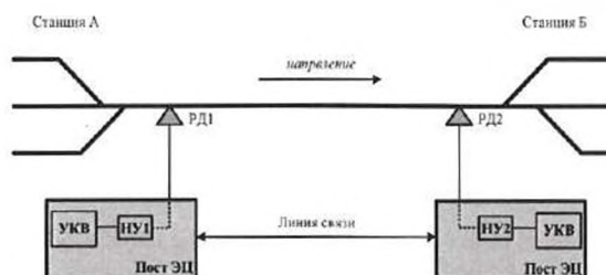
Рис.12. Обобщенная структурная схема полуавтоблокировки
