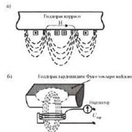
3-расм. ҒЖИД индуктив ғалтакларининг ғилдирак гардиши билан ўзаро таъсири: а) ўзаро индукция бўйича бир-бирига таъсири; б) Фуко тоқларининг пайдо бўлиши
