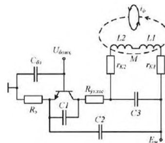
9-расм. Индуктор ғалтакларини уйғотишнинг соддалаштирилган эквивалент схемаси
