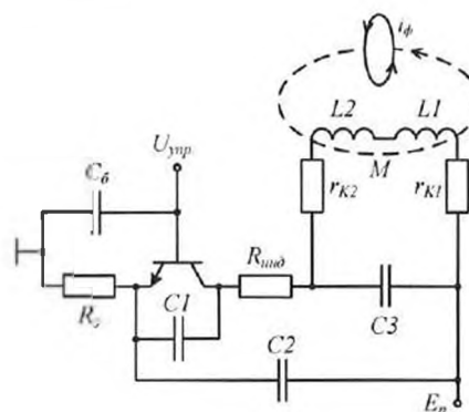
Рис.9. Упрощенная эквивалентная схема возбуждения катушек индуктора
