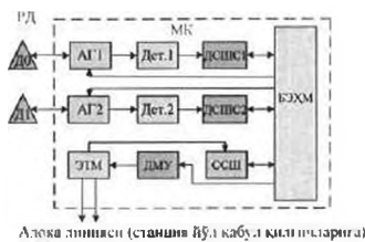
4-расм. ЎСЭТ тизимининг ҳисоблаш пунктидаги тузилавий схемаси
