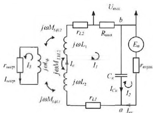
Рис.8. Эквивалентная взаимодействия катушки ДИКП и колесного гребня
