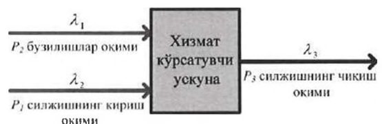
5-расм. Хизмат кўрсатувчи қурилма модели
