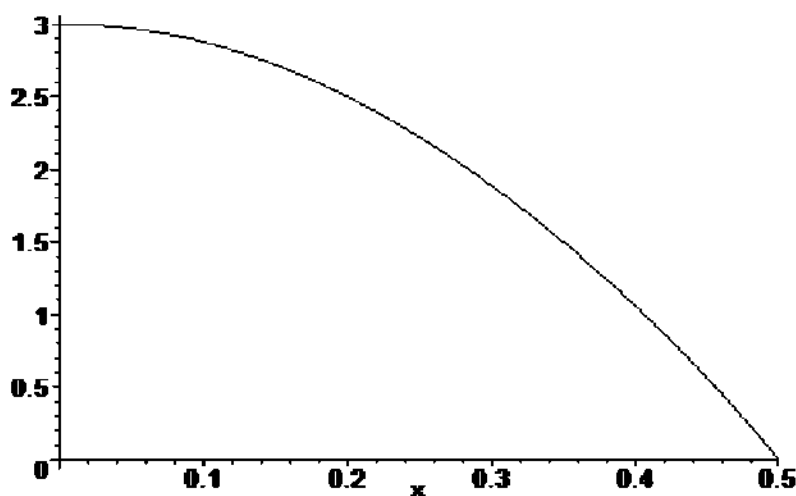
3-расм. Ўлчовсиз Юнг модуль E_0 = E/K нинг Пуассон коэффициенти \mu га нисбатан ўзгариш графика
