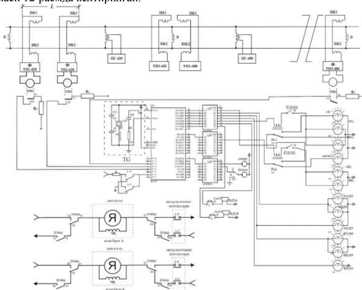
12-расм. Автошлагбаум билан микропроцессорли кесишма сигнализацияси.
