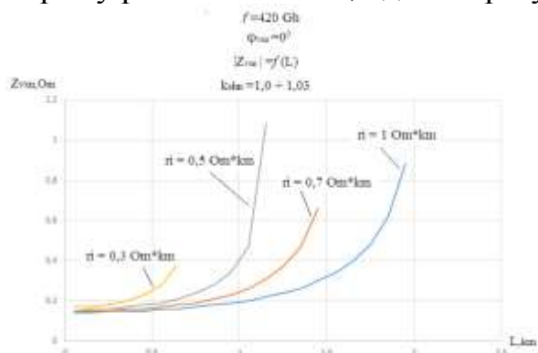
Рис. 9. Графики зависимостей входного сопротивления управляющего датчика при условии, что чувствительность шунта к длине цепи на частоте сигнала \phi_{\text{вхн}} = 0^0 и f = 420\text{Гц} .
