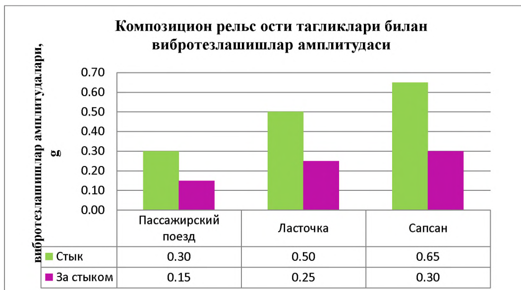
3-расм. Ер полотноси асосий майдонидаги вибротезлашишлар амплитудаси
