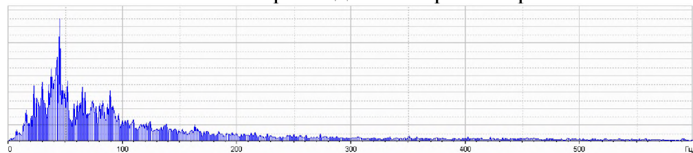
Частоты виброускорений балласта на удалении (3,3 метра от стыка) при штатных прокладках-амортизаторах
