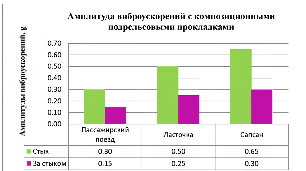
Рис.3. Амплитуда виброускорений на основной площадке земляного полотна
