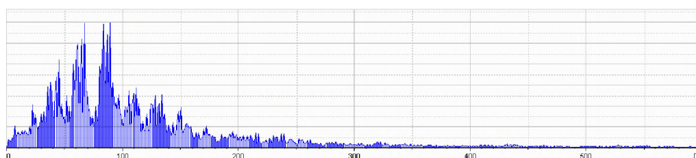
Частоты виброускорений основной площадки земляного полотна в зоне рельсового стыка при штатных прокладках-амортизаторах
