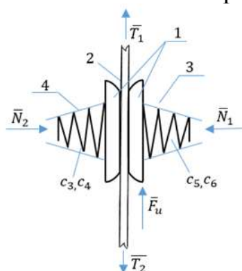
Рис.2. Расчётная схема натяжителя
