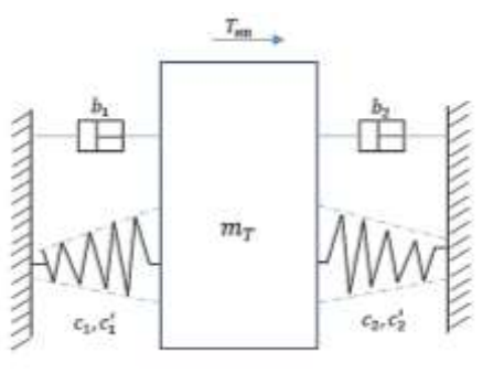
5-расм. Тавсия қилинган икки конуссимон пружинали кўзгалувчан тарелкалари бўлган игна ипини тарангловчи динамик модели.
