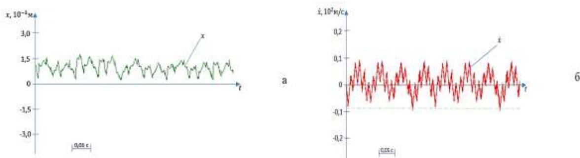
7 – расм. Игна ипини таранглагичи тарелкаларини тебранишидаги силжиш ва тезлигини тебраниш қонуниятларини конуссимон пружиналар бикрлик коэффициентларини c_1 > c_2 қилиб олингандаги кўринишлари.
