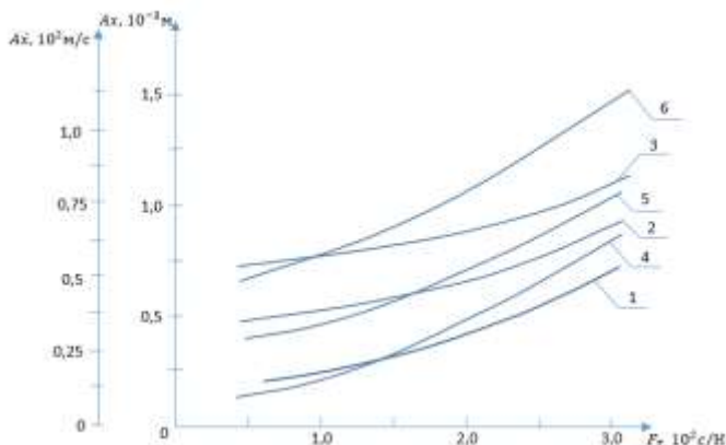
8-расм. Икки конуссимон пружинали игна ипини таранглагичи тарелкаларини силжиши ва тезлиги тебраниш амплитудаларини ташқи таранглаш кучини ўзгаришиға боғлиқлик графиклари.
