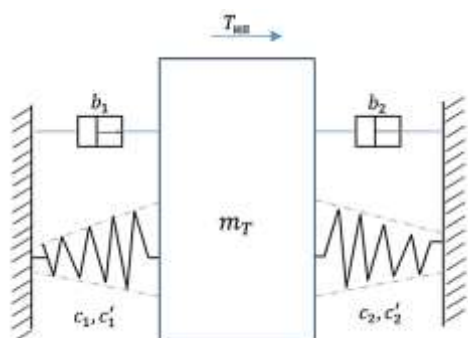
Рис. 5. Предлагаемая динамическая модель натяжения игольной нити с двумя коническими пружинами прижимающие тарелки
