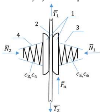
2-расм. Таранглагич ҳисоб схемаси
