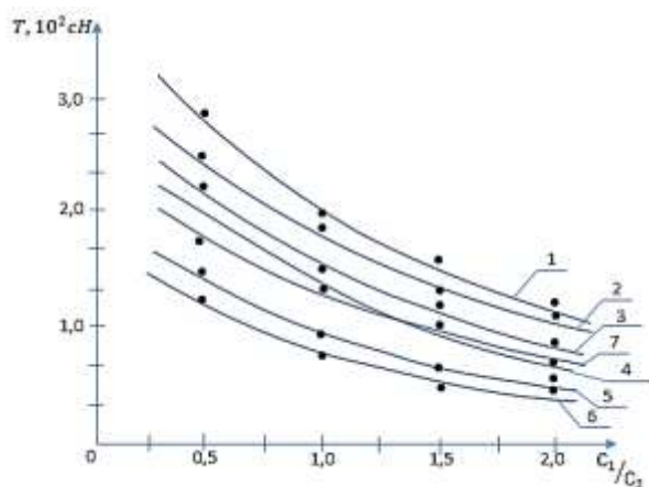
12– расм. Тавсия қилинган игна ипини таранглагичга ипни кириш ва чиқишидаги тарангликларини конуссимон базавий ва созловчи пружиналар бикрликлари нисбатини ўзгаришига боғлиқлик графиклари.
