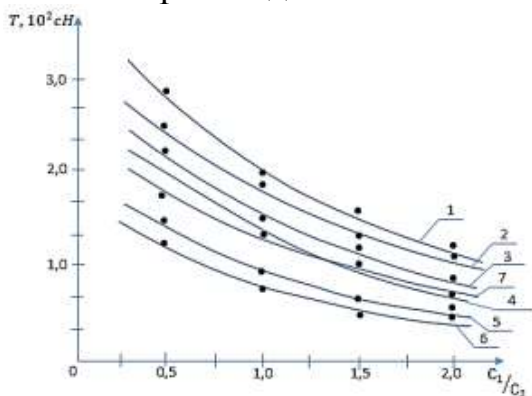
Рис. 12. Графические зависимости изменения натяжений на входе и выходе нити из рекомендованного натяжителя игольной нити от изменения соотношений жёсткостей конических базовой и регулирующей пружин
