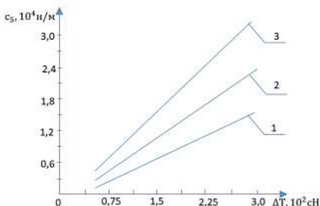
Рис. 4. Зависимости изменения линейной составляющей коэффициента жесткости прижимающей регулирующей конической пружины рекомендуемого натяжителя
