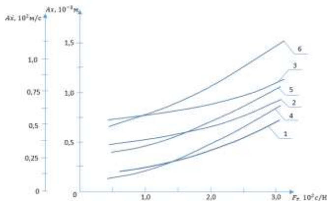
Рис.8. Графические зависимости изменения смещений и скоростей тарелок с двумя коническими пружин от изменения амплитуд колебаний силы внешнего натяжения.
