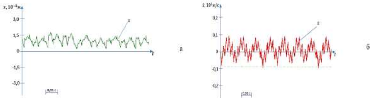
Рис. 7. Закономерности изменения смещении и скоростей колебаний тарелок натяжителя игольной нити при коэффициентах жёсткостей конических пружин c_1 > c_2
