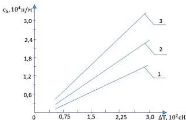
4-расм. Тавсия қилинган игна ипини таранглаши сиқувчи-созловчи конуссимон пружинаси бикрлик коэффициентини чизикли ташкил этувчи қийматини ип таранглигини фарқига боғлиқлик графиги.
