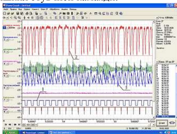
10-расм. Мавжуд тикув машинасидаги бош валнинг тезлиги (1), игна ипини таранглагичга кириш (2) ва чиқишидаги (3) таранглик кучларини ўзгариш қонуниятлари.
