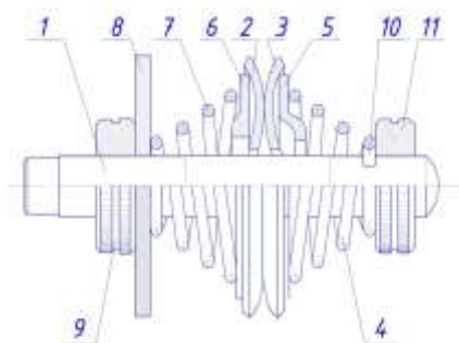
Рис.1. Конструктивная схема тарельчатого натяжителя игольной нити с двумя коническими пружинами
