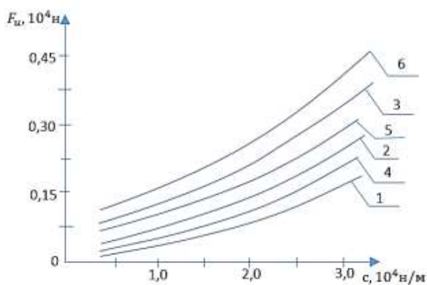
3-расм. Тавсия қилинган икки пружинали тарелкали ип таранглагичда ип билан тарелкалар орасидаги ишқаланиш кучини сиқувчи конуссимон пружиналар бикрлик коэффицентларига боғлиқлик графиклари.
