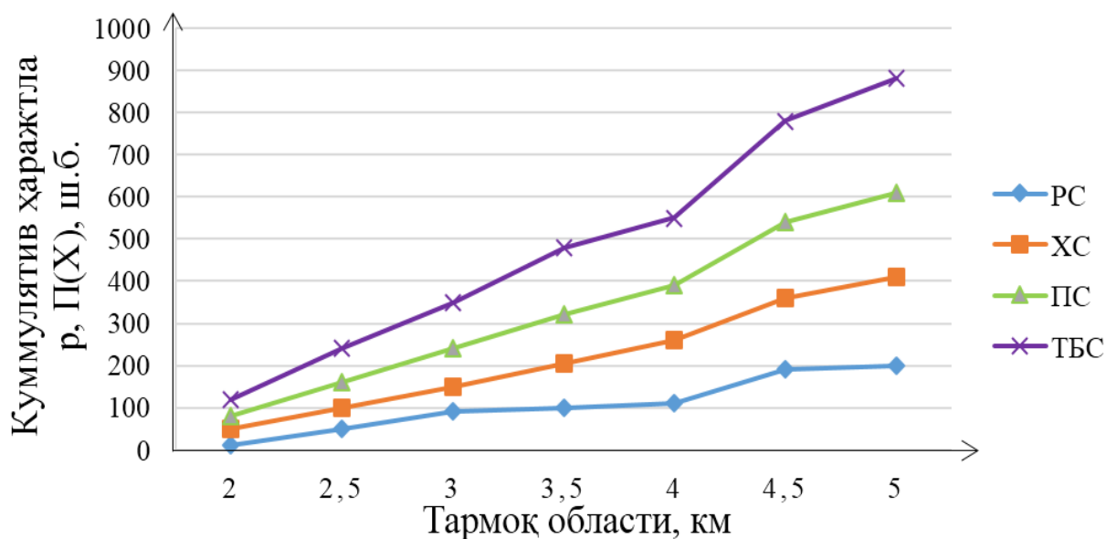
3-расм. Куммулятив ҳаражатларнинг тармоқ ўлчамига боғлиқлиги
