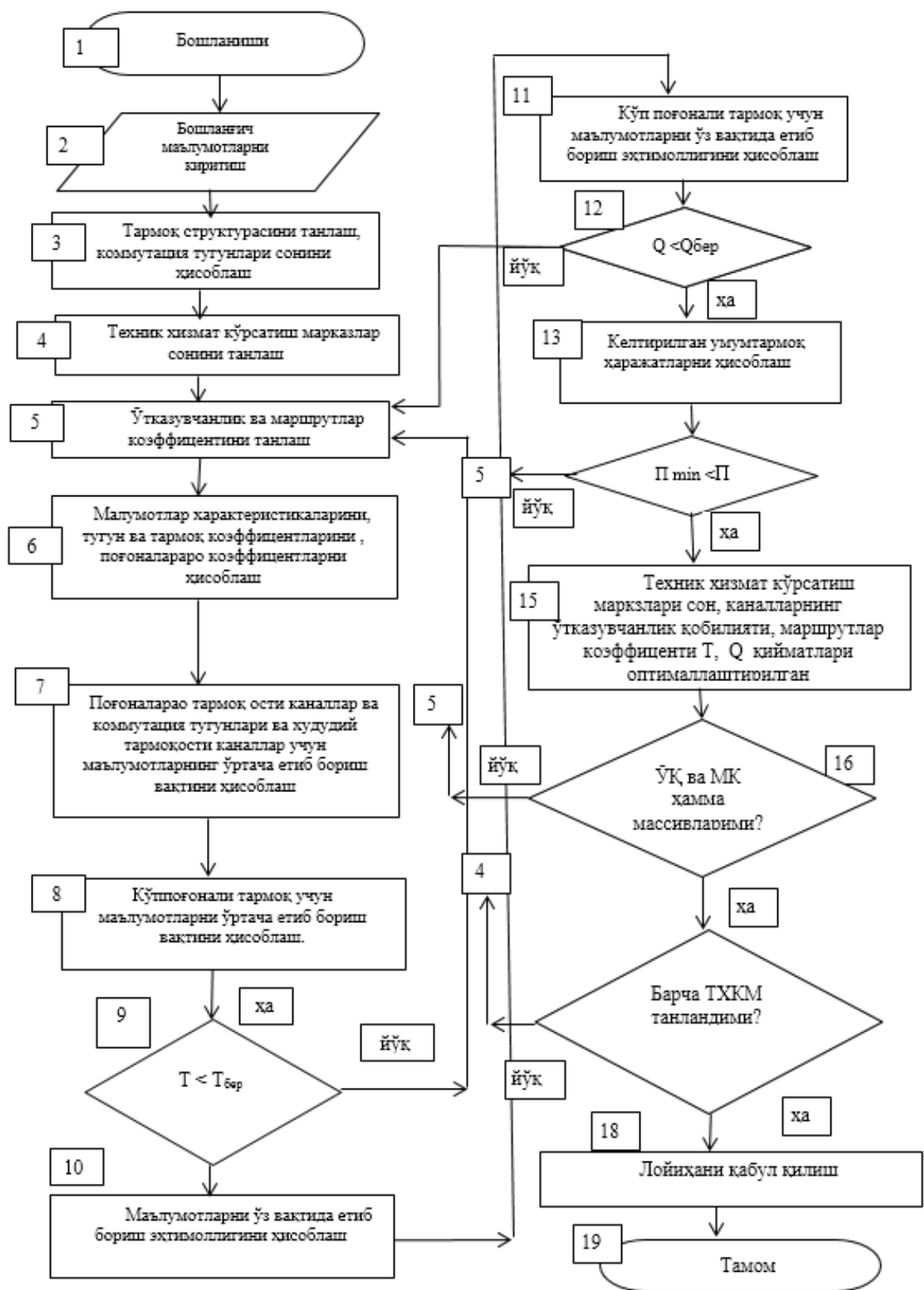
6-расм. Умумтармоқ куммулятив ҳаражатлар мезони бўйича тармоқ структурасини оптималлаштириш алгоритми
