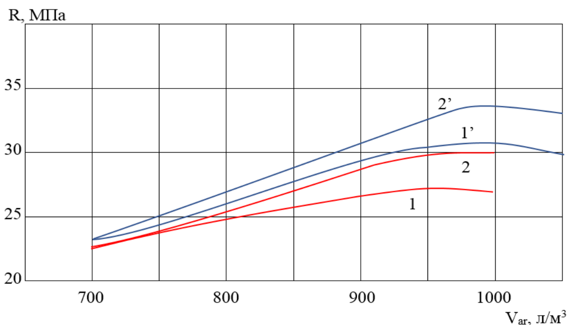
Рис. 3. Влияние расхода крупного заполнителя на прочность легкого бетона при: постоянной прочности растворной составляющей (1, 1') и постоянном расходе цемента (2, 2') ; 1, 2 – данные нашей работы для легкого бетона на новом пористом заполнителе; 1', 2' – данные работы для керамзитобетона.
