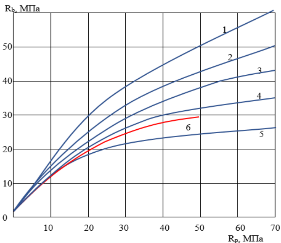
Рис. 5. Зависимость прочности бетона ( R_b ) от прочности растворной части ( R_p ): 1,2,3,4,5-прочность керамзитобетона на керамзите соответственно, 7,0; 6,0; 4,0; 3,0; 2,0 МПа по данным Ю.М. Баженова; 6-на новом пористом заполнителе из кварцевых порфиров и зауглероженной глины с прочностью 2,0-2,5 МПа.
