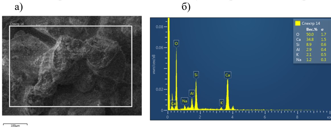
Рис.8.а)х100μм Микроструктура образца раствора: Цемент, песок и зола-унос; б) Рентгенофазовый анализ.
