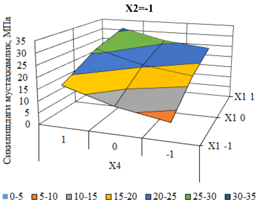
2-расм. Ўртача зичликнинг цемент сарфига ва С/Ц нисбатига полином боғлиқлиги.
