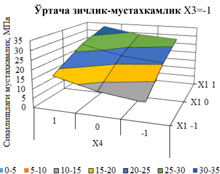
1-расм. Ўртача зичликнинг цемент сарфига ва С/Ц нисбатига чизиқли боғлиқлиги.
