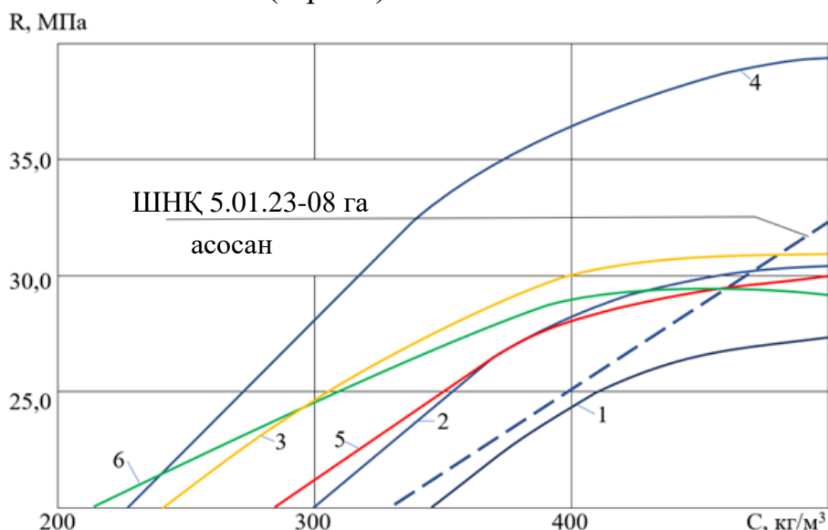
4-расм. Цемент сарфининг енгил бетон мустаҳкамлилигига таъсири: 1,2,3-керамзит R=2,8-3,2 МПа билан, мос равишда, 750, 850, 950 л/м 3 , 4-керамзит R=3,0-3,6 МПа билан, 950 л/м 3 маълумотлари бўйича, 5,6- янги зовак тўлдирувчили R=2,3-2,7 МПа, билан, мос равишда 950, 1050 л/м 3 .
