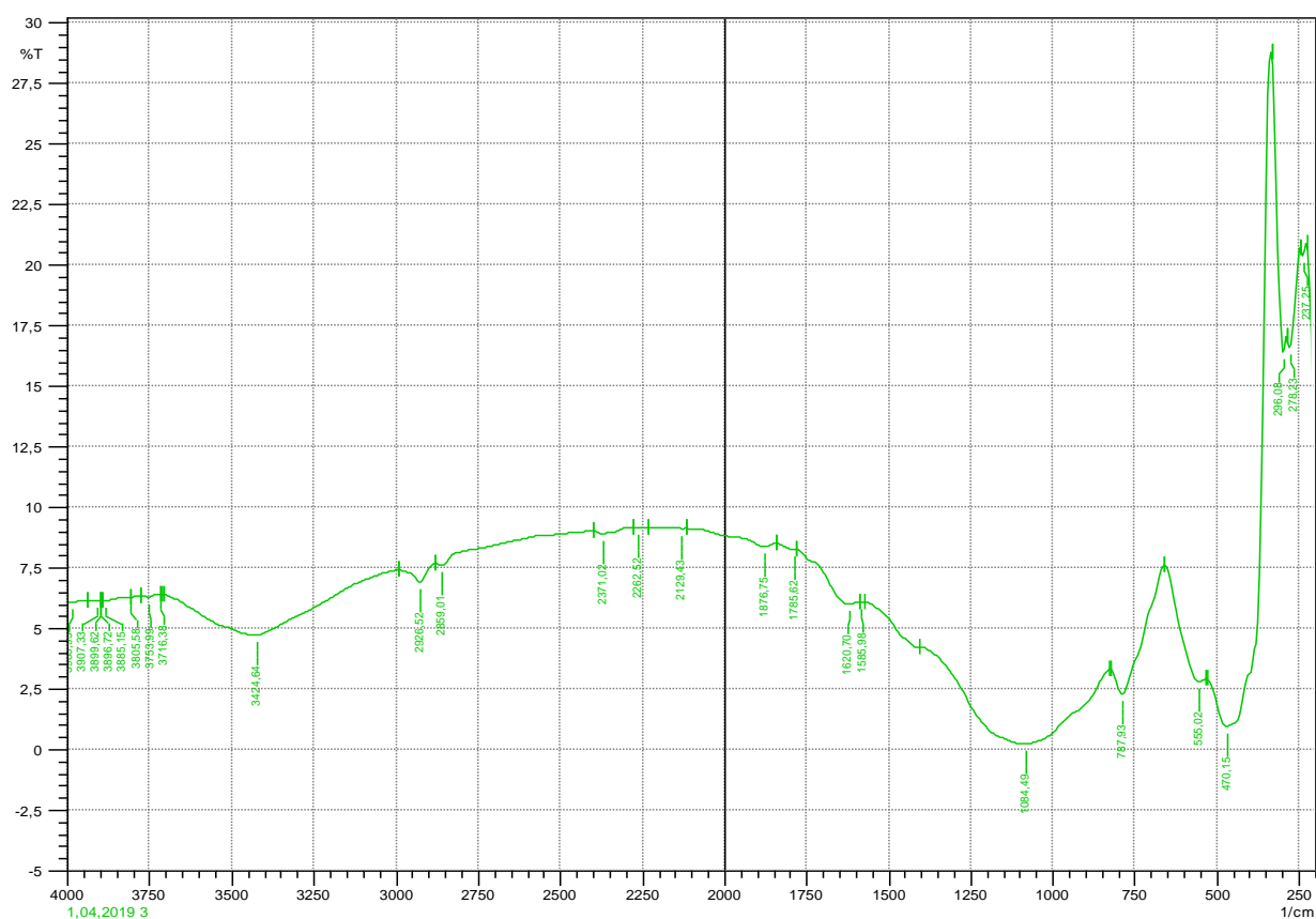
Рис. 6. ИК спектр золы-уноса Ангреного ТЭС
