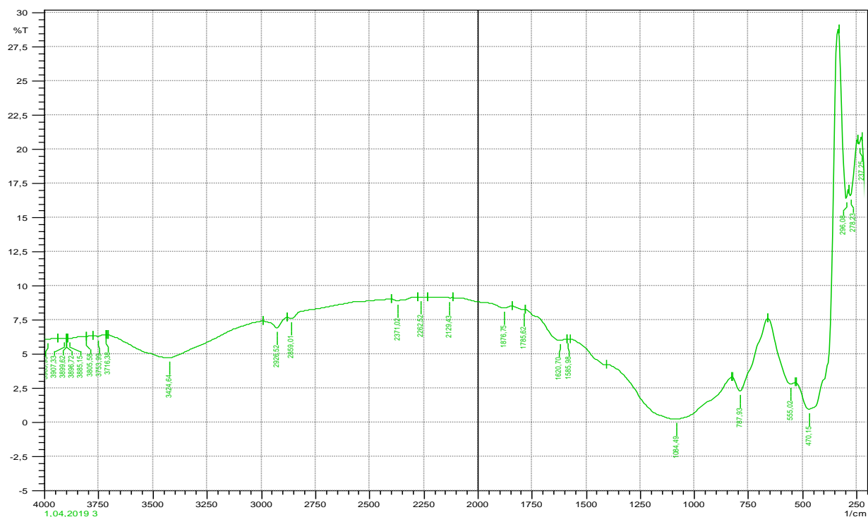
6-расм. Ангрэн ИЭС учувчан кулнинг ИҚ спектри
