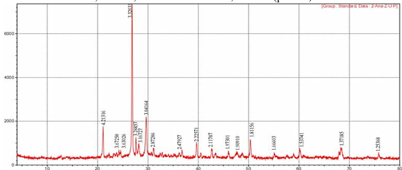
Рис. 7. Рентгенограмма (28 сут.) образца раствора: Цемента, песка и зола-уноса.
