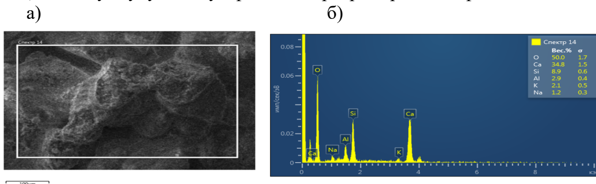
8-расм. а) \times 100\mu\text{m} қоришма наъмунаси микроструктураси: Цемент, қум ва учувчан кул; б) Рентгенофаза таҳлил.
