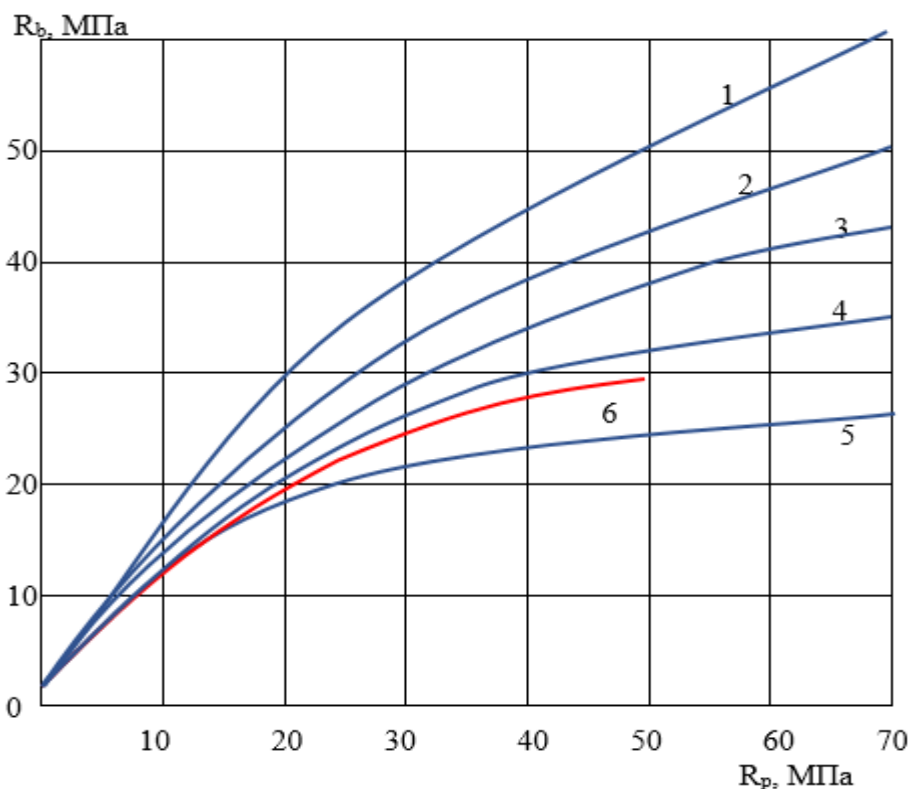
5-расм. Енгил бетон мустаҳкамлигининг ( R_b ) қоришма қисми мустаҳкамлигига ( R_p ) боғлиқлиги: 1,2,3,4,5-Ю.М. Баженев маълумотлари бўйича керамзитли керамзитобетоннинг мустаҳкамлиги мос равишда 7,0; 6,0; 4,0; 3,0; 2,0 МПа; 6- мустаҳкамлиги 2,0-2,5 МПа бўлган кварцли порфир ва кўмирланган гил тупроқли янги зовак тўлдирувчида.
