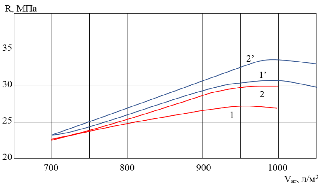
3-расм. Ғовак тўлдирувчи сарфининг энгил бетон мустаҳкамлилигига таъсири: қоршима таркибининг доимий мустаҳкамлиги (1, 1') ва цементнинг доимий сарфи (2, 2'); 1, 2 –янги ғовак тўлдирувчили энгил бетон учун тадқиқот маълумотлари; 1', 2' - керамзитобетон учун маълумотлар.
