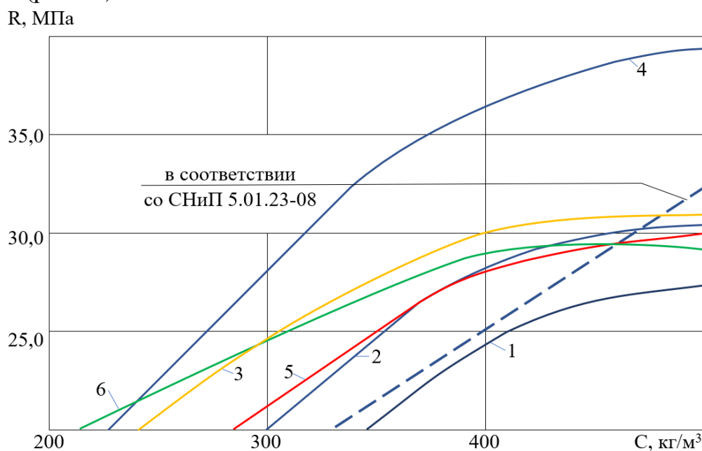
Рис. 4. Влияние расхода цемента на прочность легкого бетона при расходе: 1,2,3-керамзита с R=2,8-3,2 МПа, соответственно, 750, 850, 950 л/м 3 , 4-керамзита с R=3,0-3,6 МПа 950 л/м 3 по данным, 5,6-на новом пористом заполнителе с R=2,3-2,7 МПа, 950, 1050 л/м 3 .
