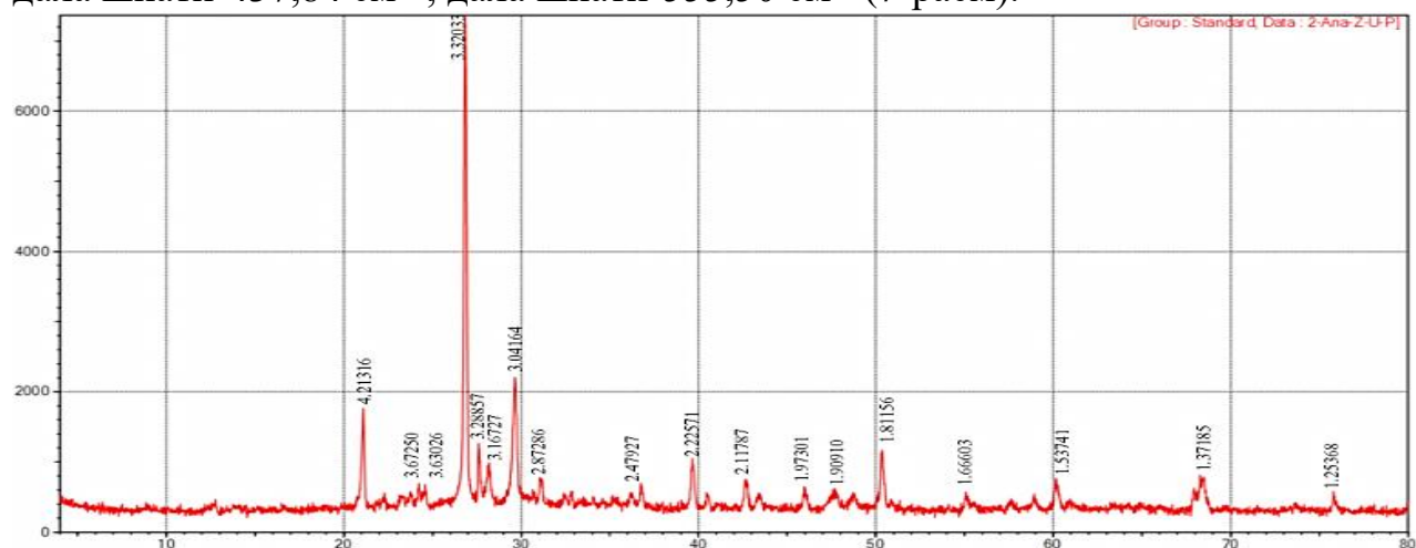
7-расм. Қоришма наъмунасининг рентгенограммаси (28 сут.): Цемент, қум ва учувчан кул.
