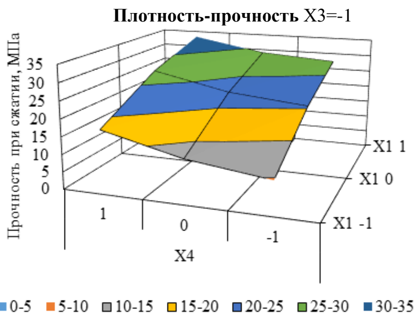
Рис. 1. Линейная зависимость плотности от расхода цемента и В/Ц.
