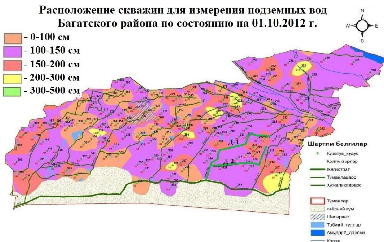
Рис. 5. Расположение скважин для измерения подземных вод исследуемых коллекторно-дренажных сетей в Багатском районе Хорезмской области
