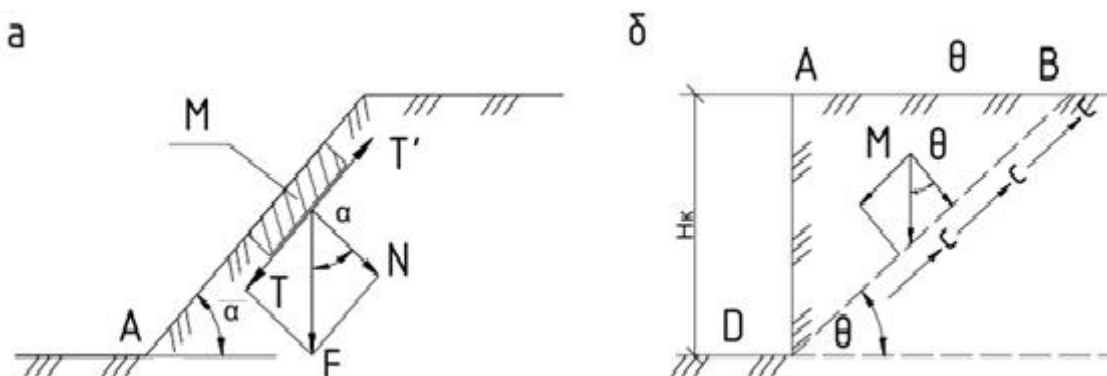
Рис. 8. Схема сил, действующих на частицу M на откосе: а – неуплотненный грунт; б- уплотненный грунт
