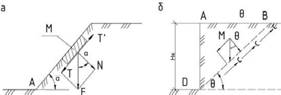
8-расм. Қияликдаги M заррасига таъсир этувчи кучлар схемаси: a – бирикмайдиган грунт; b - бирикувчан грунт
