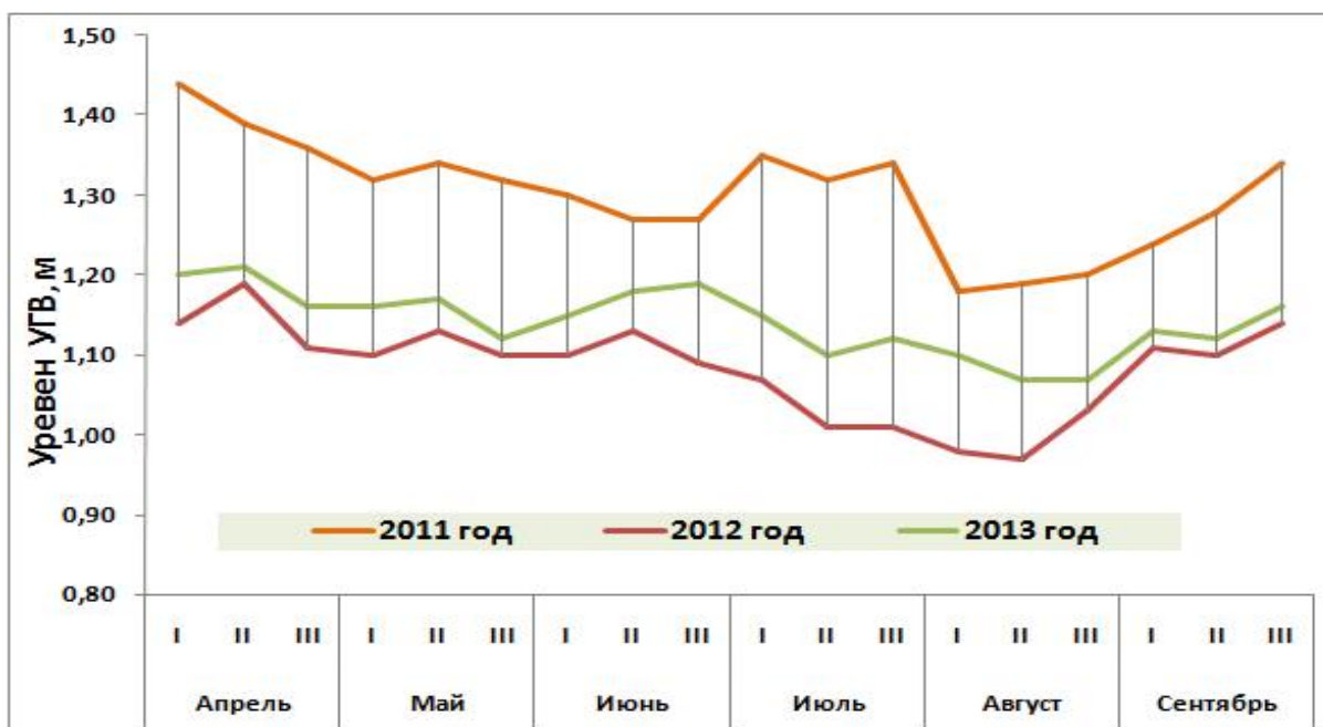
Рис. 6. Понижение уровня грунтовых вод после окашивания коллекторно-дренажной сети Д-1 с помощью ковш-косилкой
