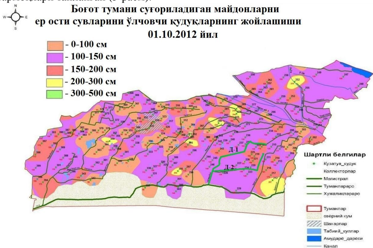
5-расм. Хоразм вилояти Боғот туманидаги ўрганилаётган очиқ коллектор ва зовур тармоқларининг ер ости сувларини ўлчовчи қудуқларнинг жойлашиши
