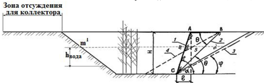
Рис. 7. Теоретическая схема расчета устойчивости откосов коллектора:
