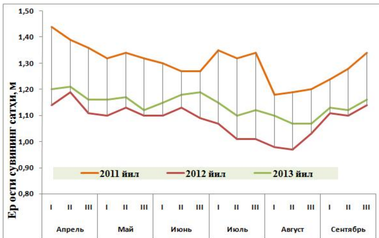
6-расм. Ковш-ўргич ёрдамида Д-1 коллектор-дренаж тармоғини ўриб олингандан сўнг ер ости сувларисатҳининг пасайиши
