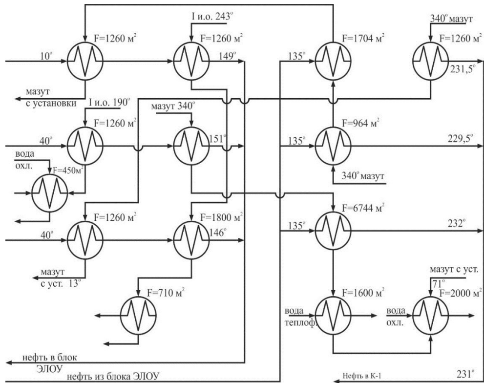
Рис. 2. Оптимальная система теплообмена установки при производительности 8 млн.т/год.
