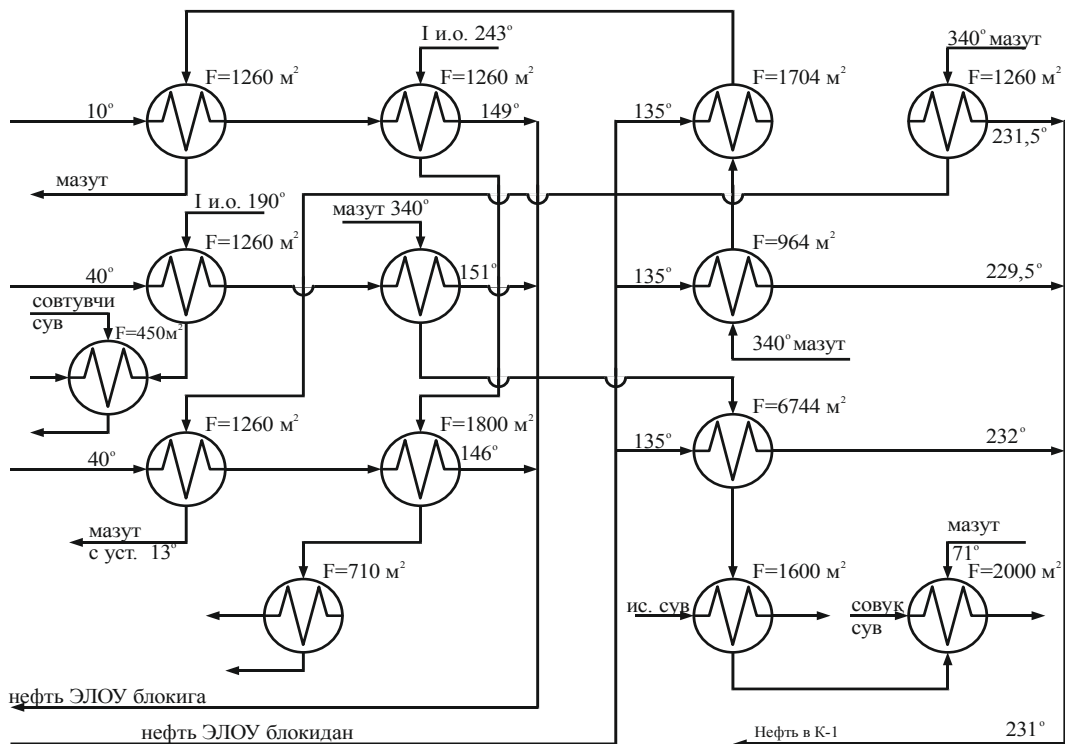
2-расм. Ишлаб чиқариш қуввати йилига 8 миллион тонна бўлган қурилманинг оптимал иссиқлик алмашиниш тизими
