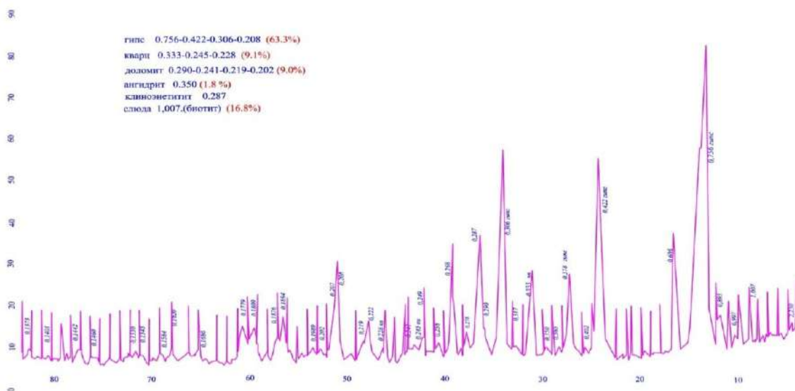
расм. Исмоил Сомоний мақбараси учун мўлжалланган модификацияланган қоришма рентгенограммаси.
