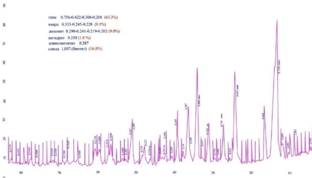
Рис. 1. Рентгенограмма модифицированного гипсового раствора разработанного для реставрации мавзолея Исмаила Самани
