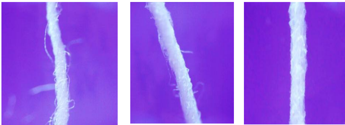
1-расм. а). Охорланмаган танда ип, б). Аънавий крахмал иштирокида охорланган ип, в). Крахмал+ГАЭ +Узхитан иштирокида охорланган ипнинг микрорасмлари.
