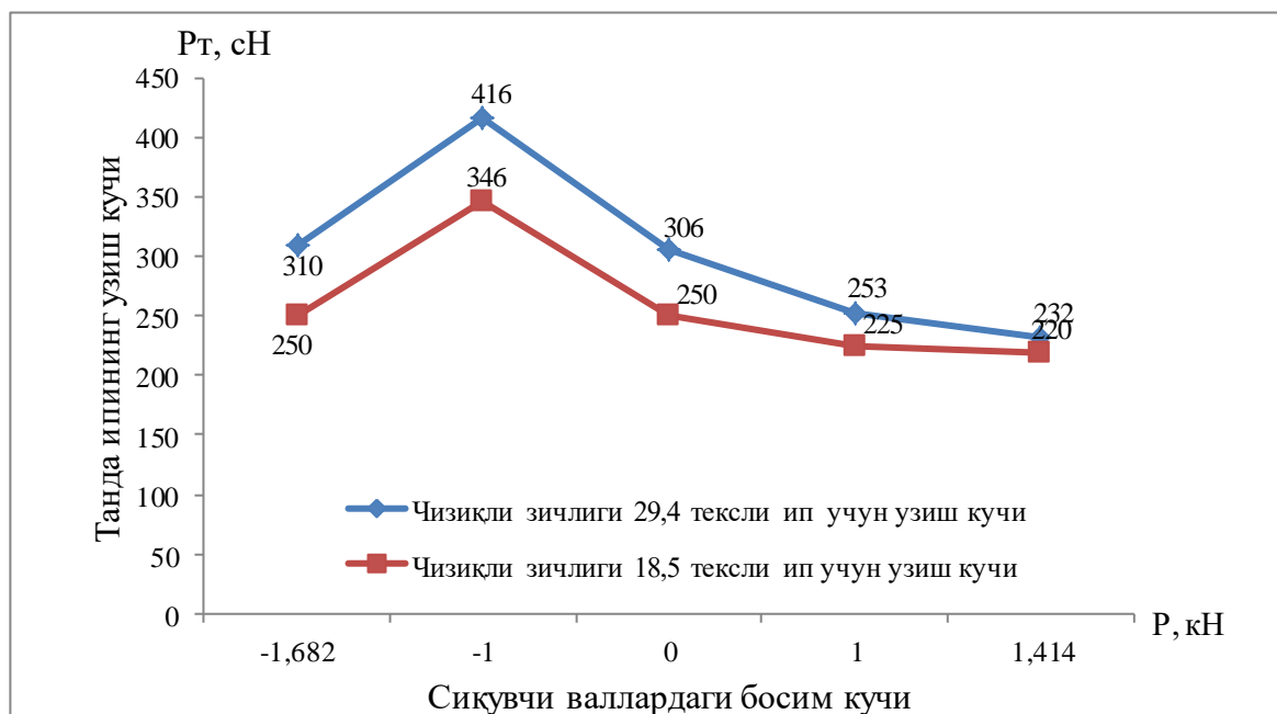
2-расм. Оҳорлаш машинасининг сиқувчи валларидаги босим кучини T_T=29,4 ва T_T=18,5 тексли ипларнинг узиш кучига таъсири.
