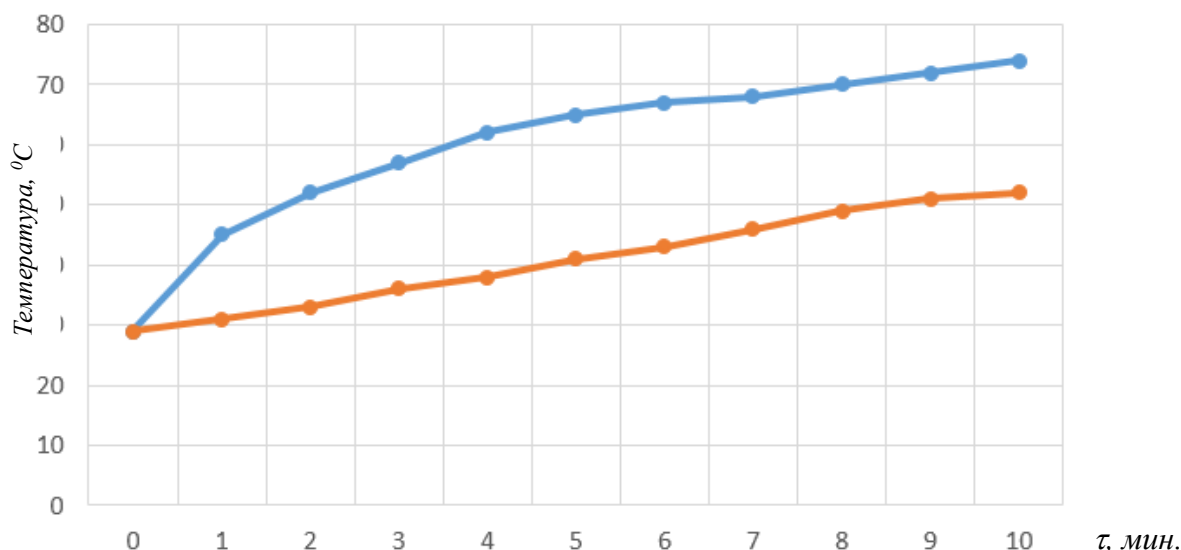
Рис.6. График изменения температуры кокона и оболочки во времени (при расстоянии между коконом и лампой 15 см):
