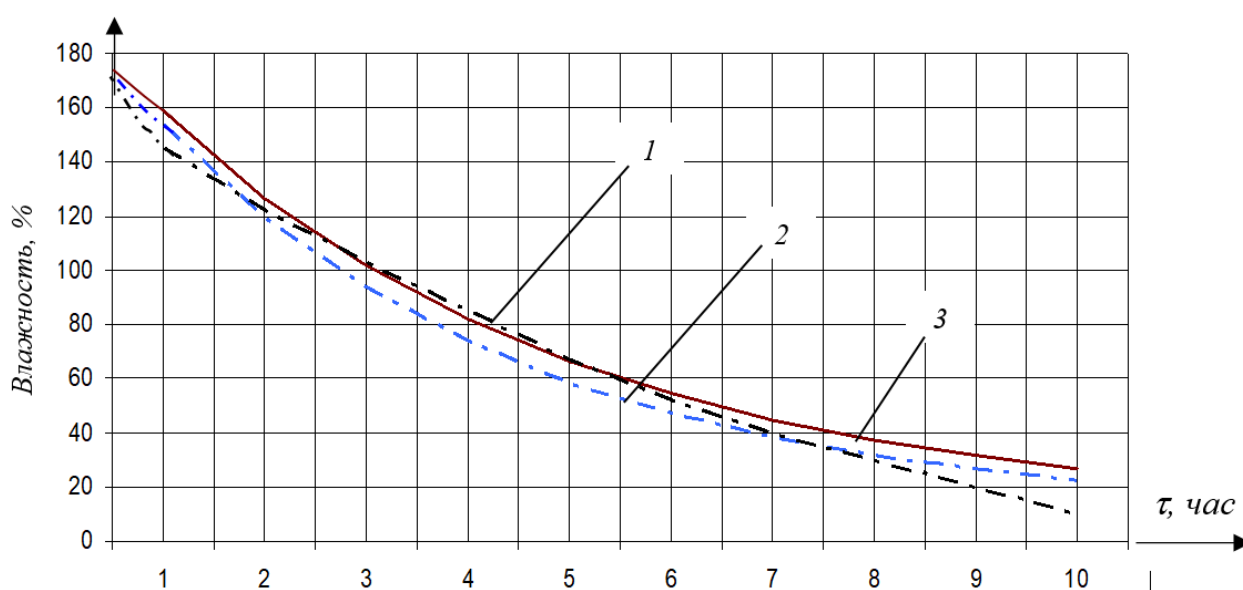
Рис. 2. График сушки коконов горячим воздухом:
