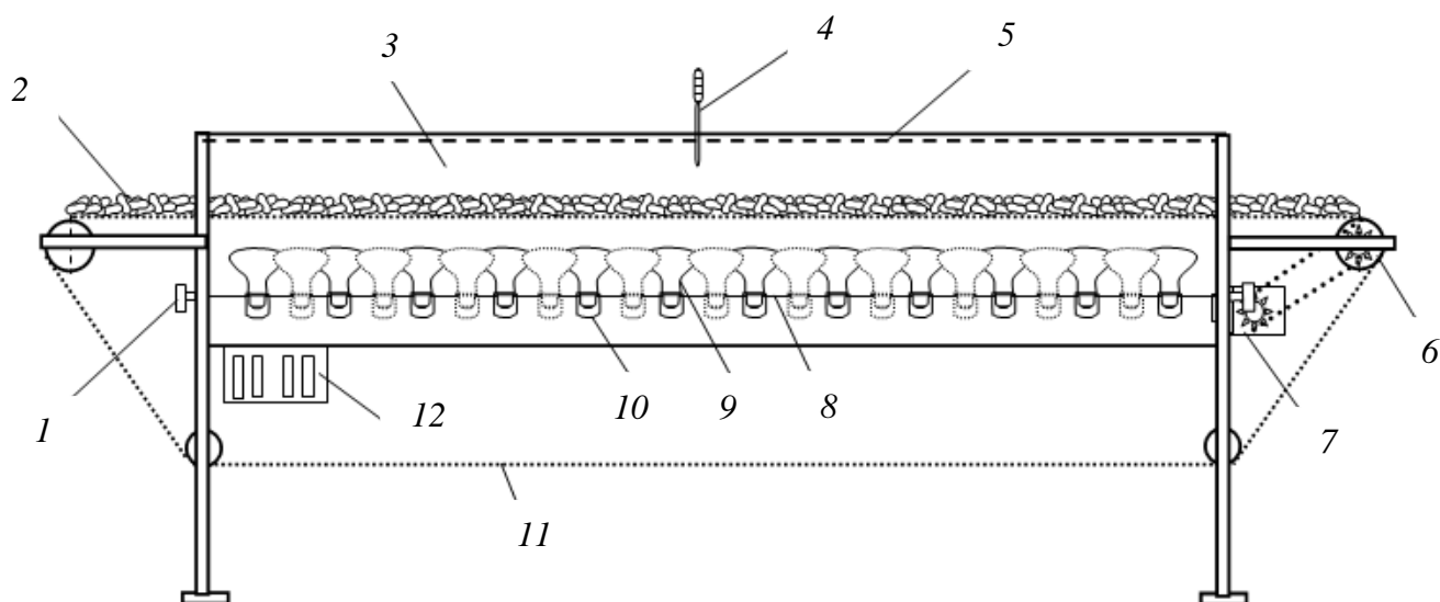
Рис.3. Технологический чертеж нового устройства для морки живой куколки шелкопряда под воздействием инфракрасного излучения
