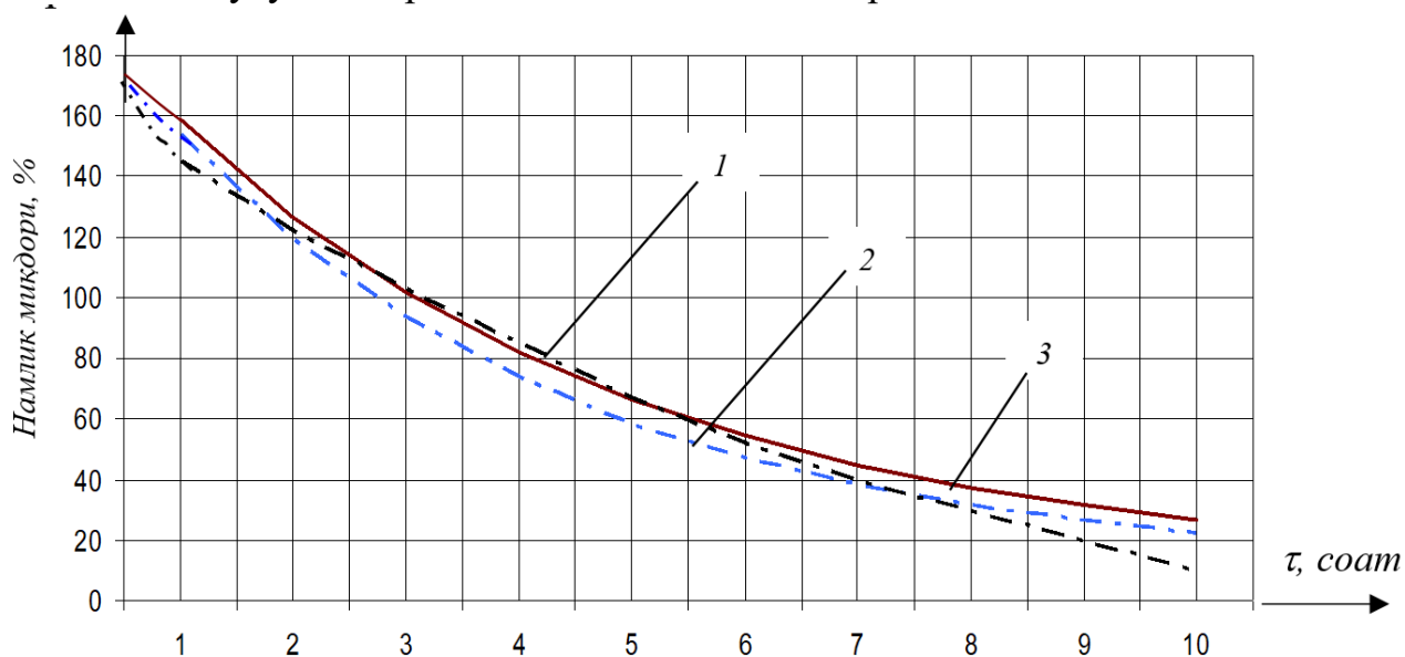
2-расм. Пиллаларни иссиқ ҳавода қуриш графиги
