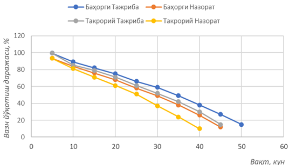
12-расм. Пиллаларни кондицион намликка қадар қуритиш давомийлигида унинг вазн ўзгаришига боғлиқлиги
