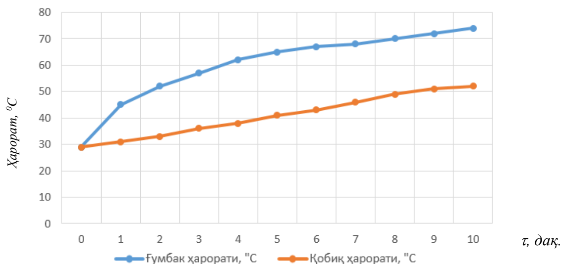
6-расм. Ғумбак ва қобиқ ҳарорати ўзгаришининг вақтга боғлиқлик графиги, (Пилла ва лампа орасидаги масофа 15 см бўлганда)
