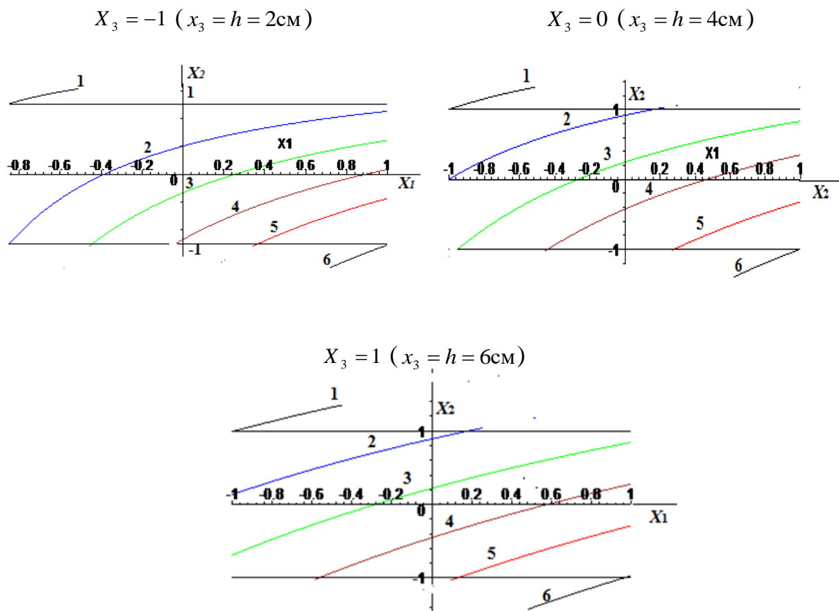
4-расм. X_2 омил (ишлов бериш вақти, мин) ва биринчи омил X_1 (пилла ва лампа орасидаги масофа, см) ларнинг ишлов берилаётган намуна қалинлиги, h=2\text{см} , h=4\text{см} ва h=6\text{см} бўлганда пилла ғумбагининг жонсизланиш даражаси \hat{y} (%) нинг ҳар хил қийматларидаги боғланиш графиклари
