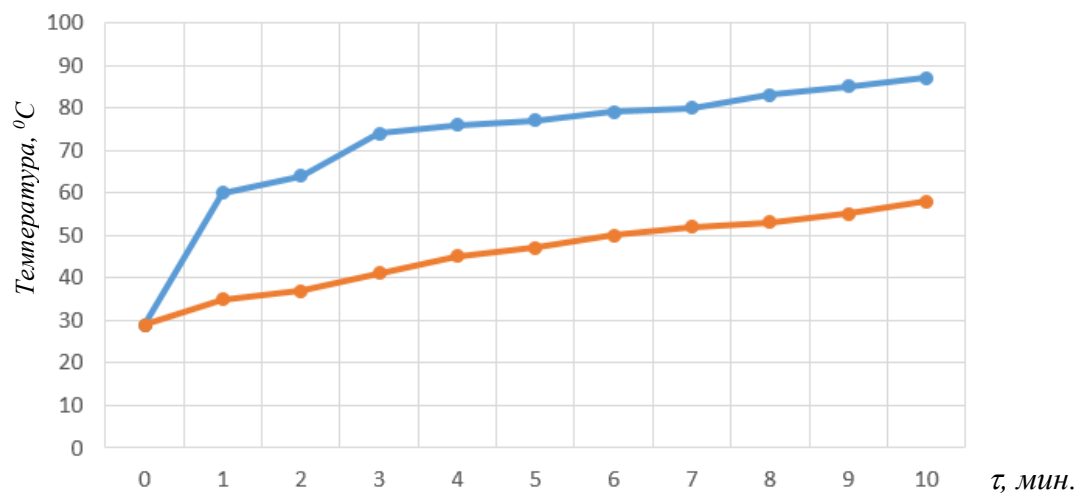
Рис.5. График изменения температуры кокона и оболочки во времени (при расстоянии между коконом и лампой 8 см); —●— температура куколки —●— температура оболочки
