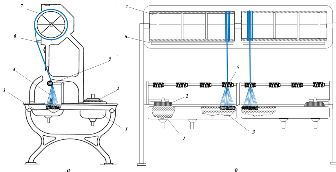
Рис.10. Технологическая схема, вид сбоку усовершенствованного механического станка для размотки дефектных коконов КМС-10ВУ:
