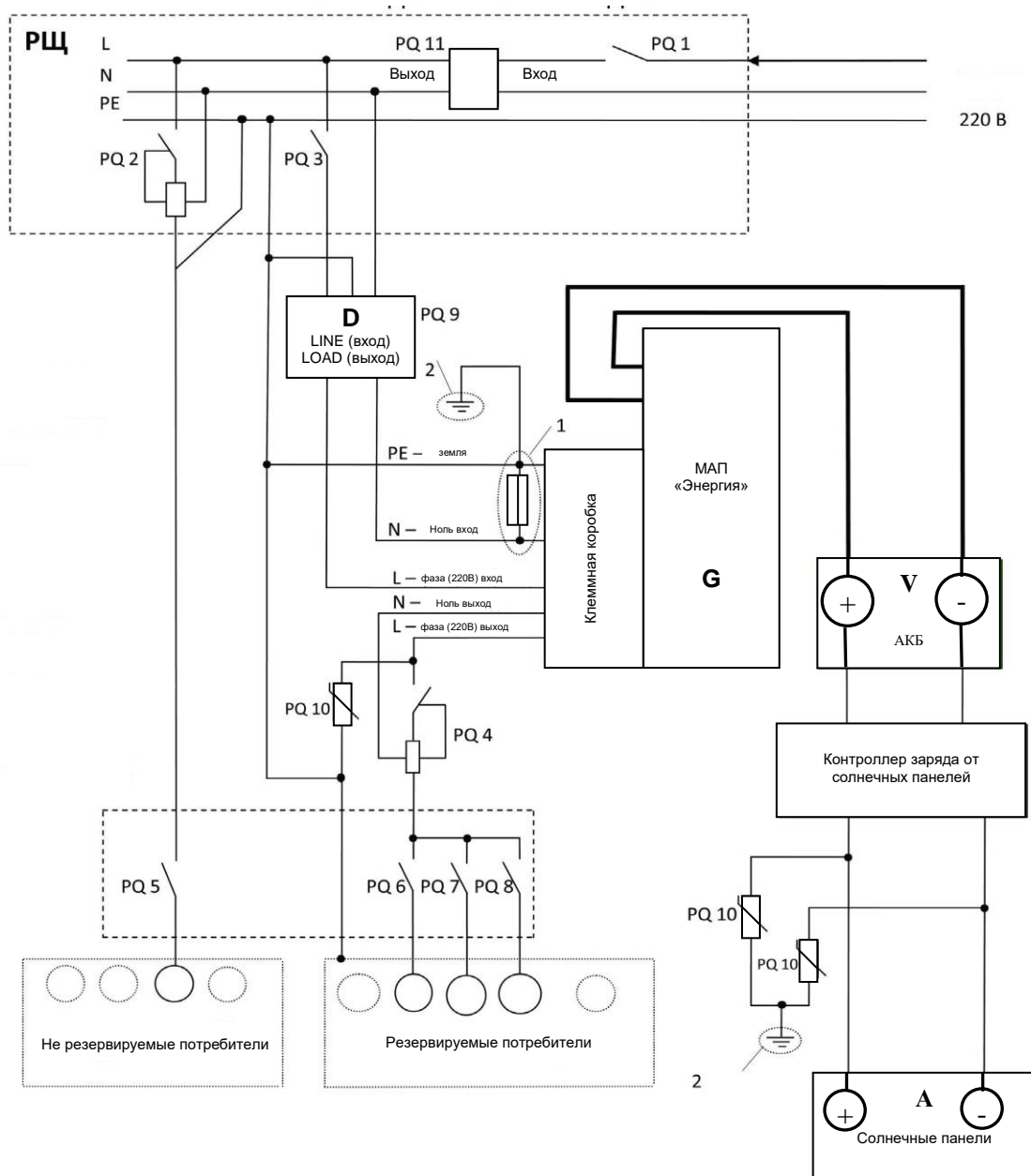
Рис.7. Схема модели фотоэлектрической системы ФЭС 100/12, обеспечивающей солнечной энергией новое устройство для замаривания куколки шелкопряда:
