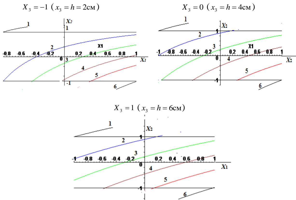
Рис.4. Связь между фактором X_2 (время обработки, мин) и первым фактором X_1 (расстояние между коконом и лампой, см) при различных значениях степени замаривания кокона (%) при толщине обрабатываемого образца h = 2 см, h = 4 см и h = 6 см.
