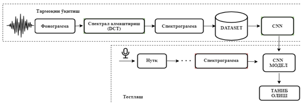
5-расм. Спектрограмма тасвирларига асосланган таниш жараёни
