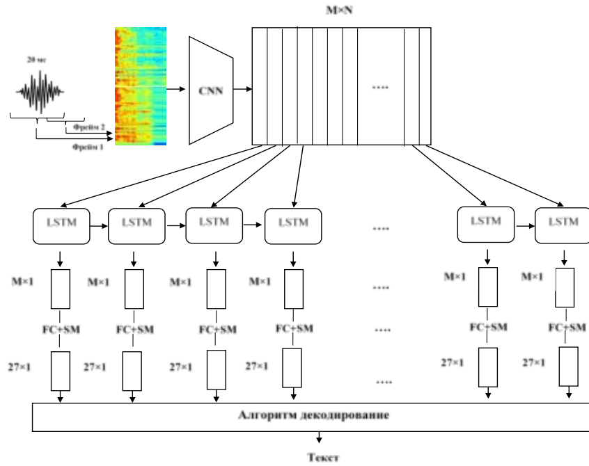
Рис. 9. Этапы акустического моделирования в рекуррентной сети Шаг 6. Процесс декодирования выполнялся на основе алгоритма CTC. Для этого вероятность всех возможных путей, представляющих метку, равна:
