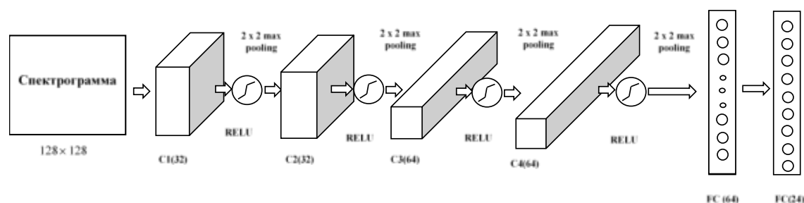
Рис.6. Архитектура CNN для распознавания речевых команд.
