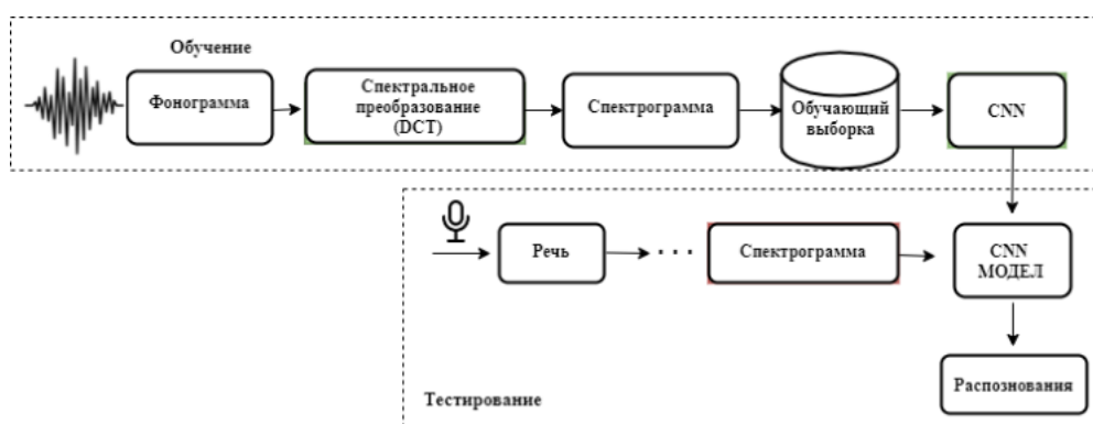
Рис. 5. Процесс распознавания речи на основе изображений спектрограмм
