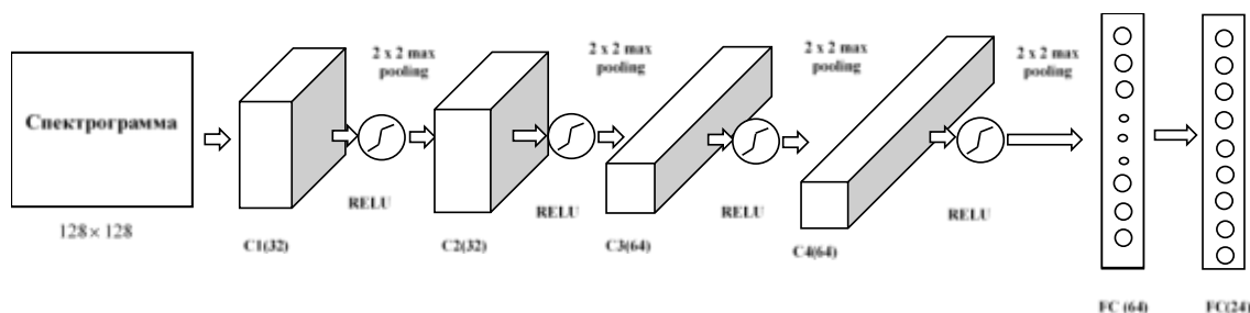
6-расм. Нутқ буйруқларини танишнинг CNN архитектураси
