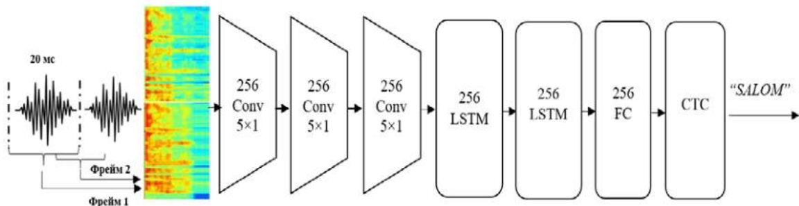
Рис. 10. Предлагаемая сетевая архитектура
