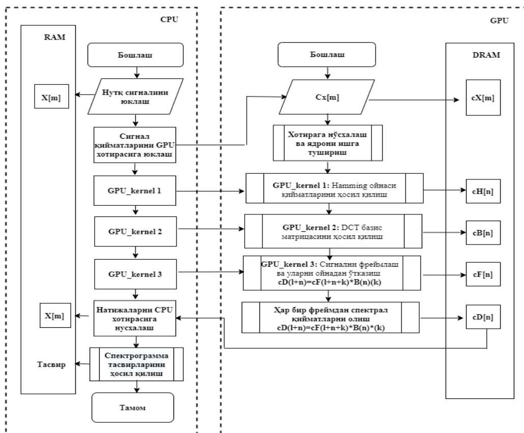
3-расм. GPU да спектрограмма тасвирларини ҳосил қилиш
