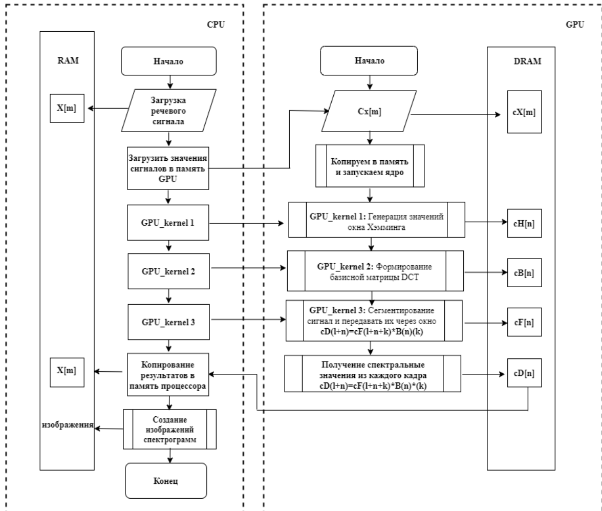
Рис. 3. Формирование изображений спектрограмм на GPU
