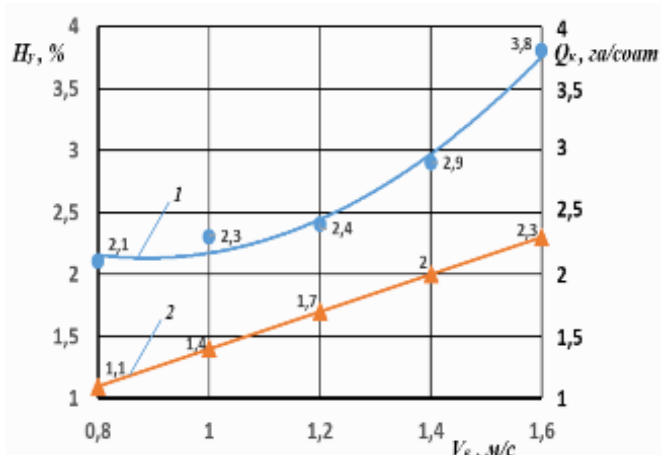
8-расм Комбайн иш тезлиги ( V_k ) нинг жаткадаги уруғ нобудгарчилиги ( H_u )га ва комбайнни иш унуми ( Q_k )га таъсири
