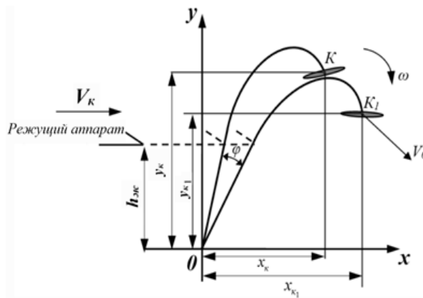
Рис.3. Схема для определения длины направителя делителя
