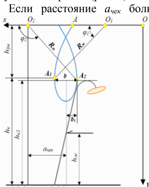
Рис.4. Траектория движения планок мотвила
