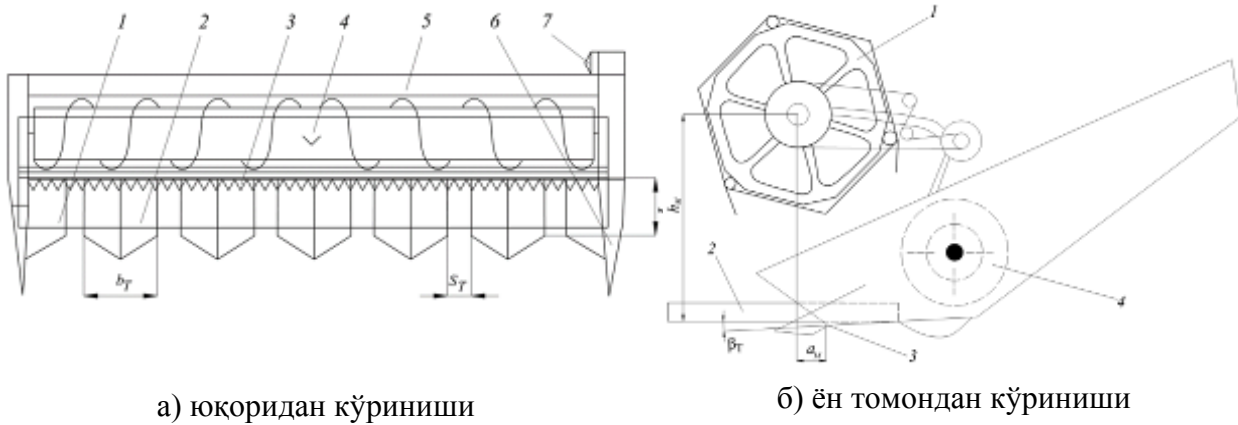
а) юкоридан кўриниши б) ён томондан кўриниши 1-расм. Кунгабоқар йиғштириш учун мослаштирилган жатка схемаси
