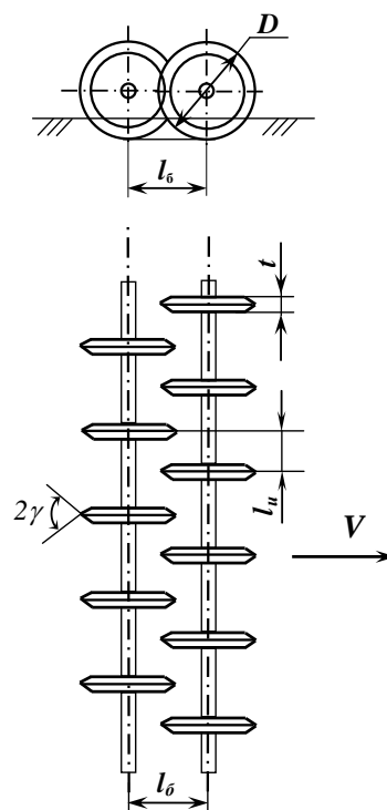
2-расм. Комбинациялашган машина ғалтакмолаларининг параметрлари
