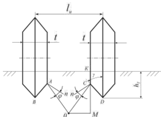
3-расм. Ғалтакмолалар дискларининг излари орасининг кенглигини аниқлашга доир схема
