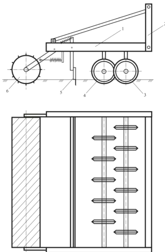
1-рама; 2-осиш қурилмаси; 3,4-дискли ғалтаклар; 5-текислагич; 6-планкали ғалтакмола 1-рasm. Янги шудгорланган далага ишлов беришда қўлланиладиган комбинациялашган машинанинг схемаси
