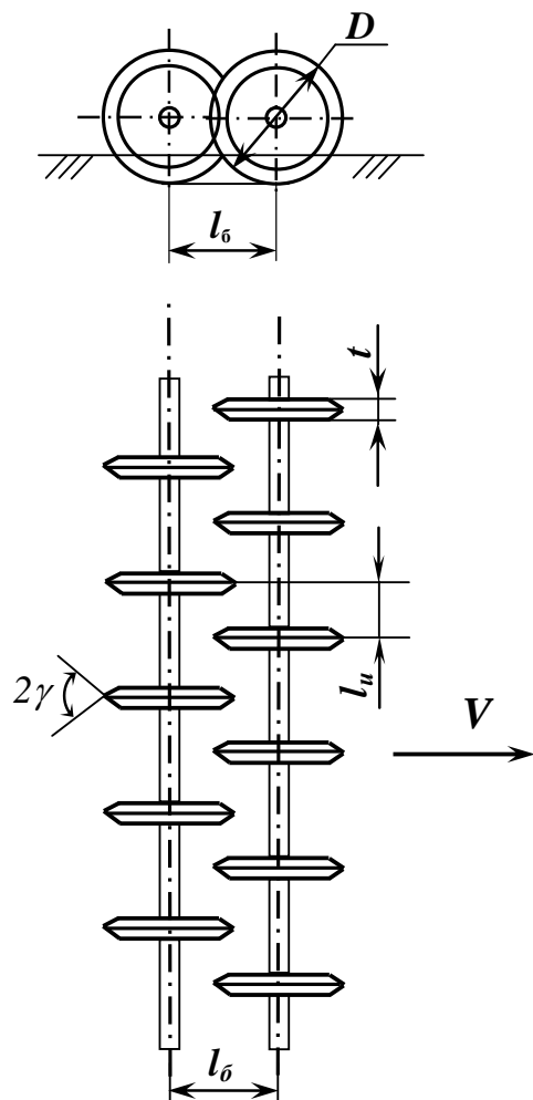
Рис. 2. Параметры дисковых катков комбинированной машины
