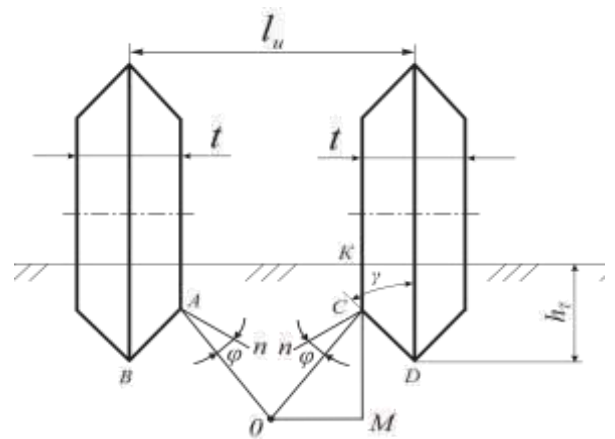
Рис.3. Схема к определению ширины междуследия дисков
