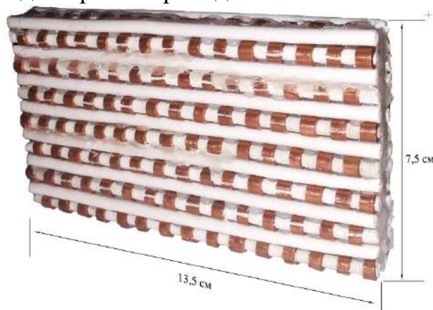
6-расм. Тақсимланган параметрга эга, адоқа линияси элементларидан иборат метаматериалнинг ҳажм бўйича катталаштирилган намунаси.
