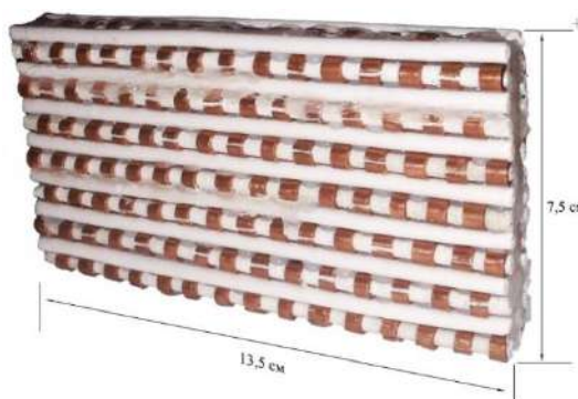
Рис.6. Увеличенный в объеме образец метаматериала, состоящий из элементов линии связи с распределенным параметром.
