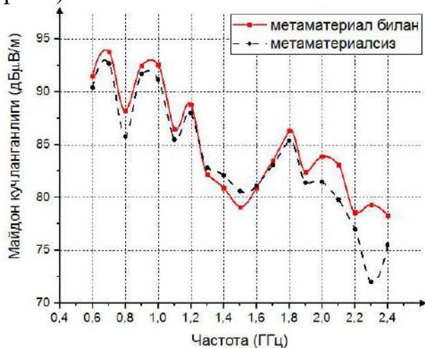
8-расм. Частота ва майдон кучлилиги ўртасидаги график: узлуксиз чизиқ – метаматериалли муҳит, узук чизиқ - метаматериалсиз муҳит.
