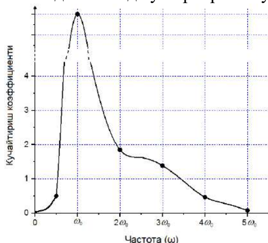
12-расм. Кучайтириш коэффициентининг частотага боғлиқлик графиги.
