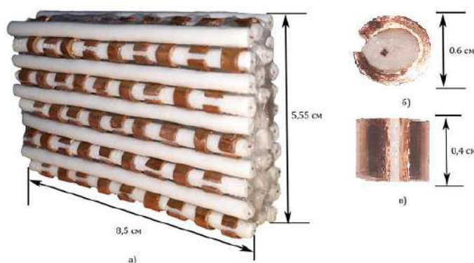
5-расм. Тақсимланган параметрларга эга, алоқа линияси элементларидан ташкил топган метаматериал (а), метаматериал элементининг юқоридан кўриниши (б), метаматериал элементининг ён томондан кўриниши (в).
