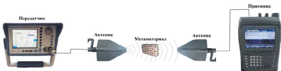
Рис.7. Установка, собранная для изучения эффективности метаматериала относительно антенно-фидерных устройств.
