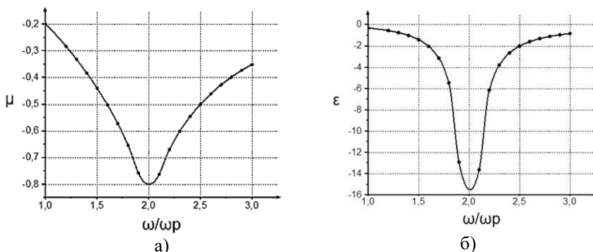
4-расм. Метаматериалнинг эквивалент схемаси бўйича магнит (а) ва диэлектрик (б) сингдирувчанликнинг частотага боғлиқ графиклари.
