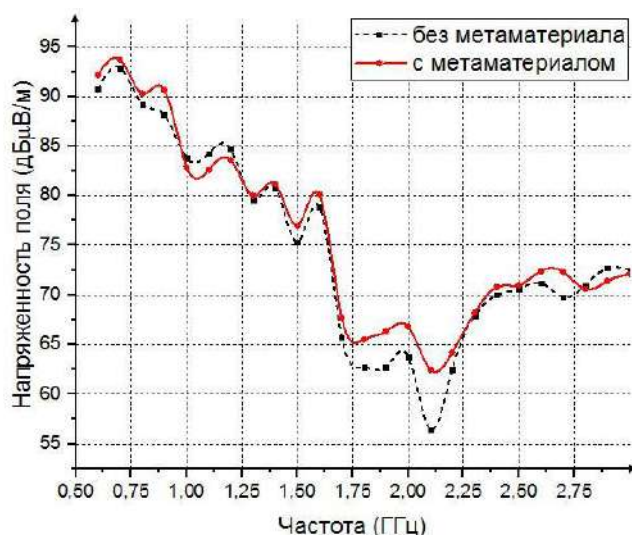
Рис.10. График между частотой и напряженностью поля метаматериала из двух слоев: сплошная линия – среда с метаматериалом, пунктирная линия – среда без метаматериала.
