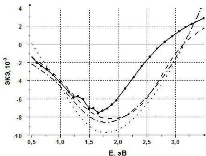
1-расм. Термо ишлов берилмаган (\text{CoFeZr})_x(\text{Al}_2\text{O}_3)_{(1-x)} нанокомпозит ( X=13\% ) учун экваториал Керр эффекти (ЭКЭ) қиймати спектрлари.
