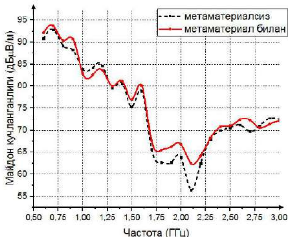
10-расм. Икки қатламли метаматериал: узлуксиз чизик– метаматериалли муҳит, узлукли чизик– метаматериалсиз муҳит.
