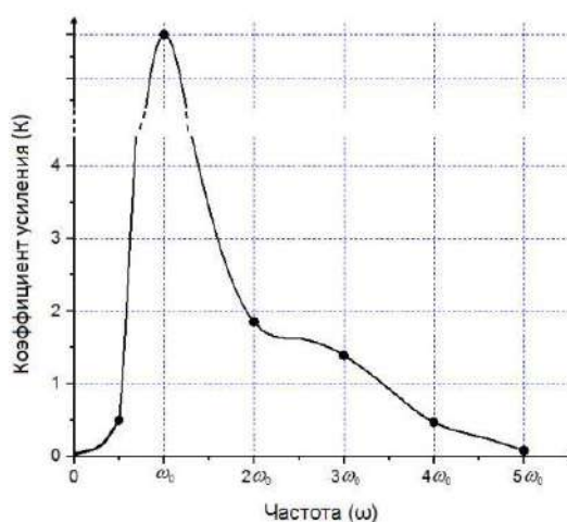
Рис.12. Зависимость коэффициента усиления от частоты.
