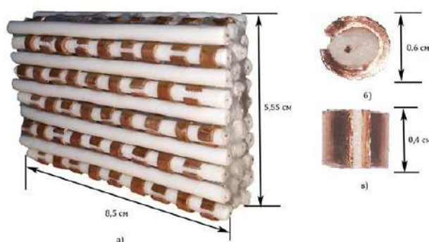
Рис.5. Метаматериал с распределенными параметрами (а), элементарная ячейка метаматериала вид сверху б), элементарная ячейка метаматериала вид сбоку (в).
