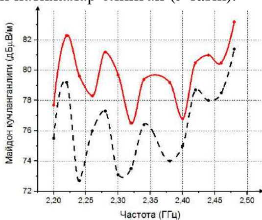
9-расм. Частота ва майдон кучлилиги ўртасидаги график: узлуксиз чизиқ – метаматериалли муҳит, узук чизиқ - метаматериалсиз муҳит.
