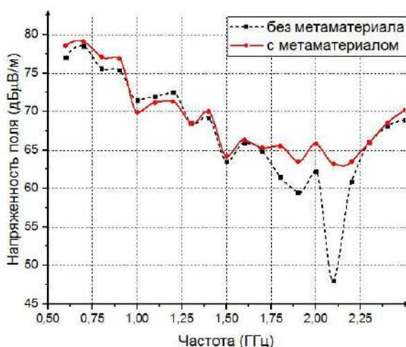
Рис.11. График между частотой и напряженностью поля метаматериала из трех слоев: сплошная линия – среда с метаматериалом, пунктирная линия – среда без метаматериала.
