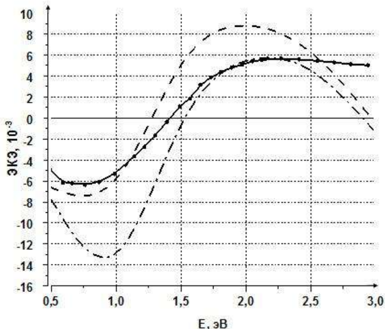
2-расм. Термоишлов берилган (CoFeZr)_x(Al_2O_3)_{(1-x)} нанокомпозит ( X=72\% ) учун экваториал Керр эффекти қиймати спектрлари.
