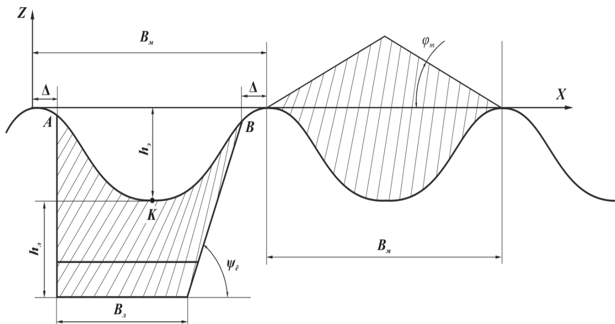
3-расм. Афдаргичли иш органи лемехининг тупроққа ботиш чуқурлиги ва пастки қисмининг камраш кенглигини аниқлашга доир схема
