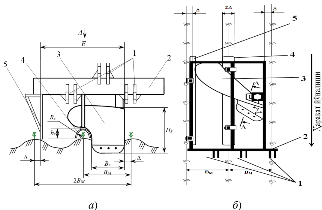
Рис.2. Конструктивная схема устройства для образования продольного пала в междурядьях хлопчатника
