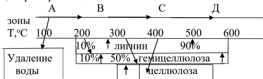
Рис.3. Схема термического разложения и горения древесины.
