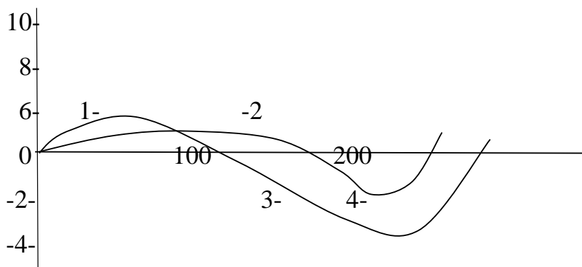
Рис. 2. Термомеханические кривые огнестойкого соснового волокна.
