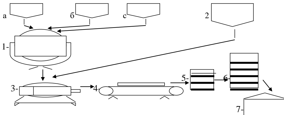
4-расм. Ғўза поя асосида оловбардош ЁҚПларни олишнинг технологик схемаси. а, б, с – ўлчагичлар, 1 – реактор-модификатор, 2 – бункер-дозатор, 3 – аралаштиргич, 4 – лентали транспортер, 5 – пресс, 6 – вагонетка, 7 – тайёр маҳсулот омбори.
