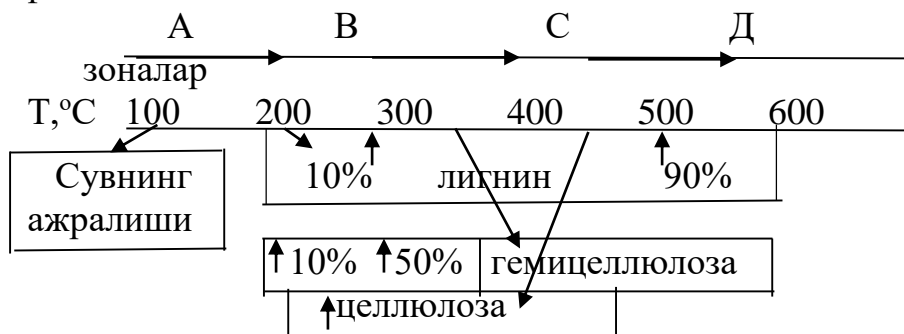
3-расм. Ёғочнинг термик парчаланиш ва ёниш схемаси.
