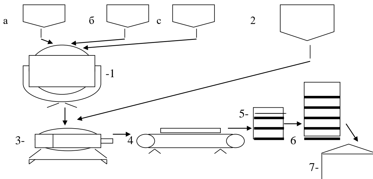
Рис.4. Принципиальная технологическая схема производства огнезащищенных ДСП из стеблей хлопчатника. а, б, с – мерники, 1 – реактор-модификатор, 2 – бункер-дозатор, 3 – смеситель, 4 – ленточный транспортер, 5 – пресс, 6 – вагонетка, 7 - склад готовой продукции.
