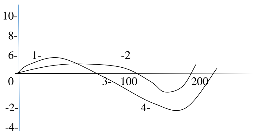
2-расм. Қарағай ёғоч толасининг термомеханик эгрлари
