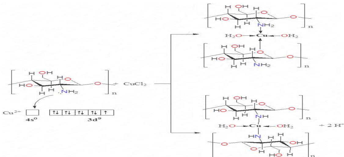
1-расм. Хитозан ва мис ионлари асосида ПМК ишлаб чиқаришда кимёвий реакциялар схемаси
