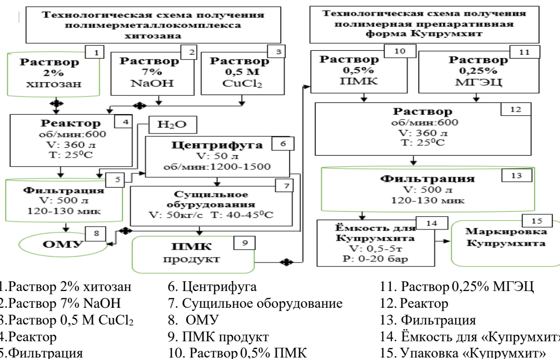
Рис.7. Последовательные стадии производства полимерной препаративной формы Купрумхита и ПМК
