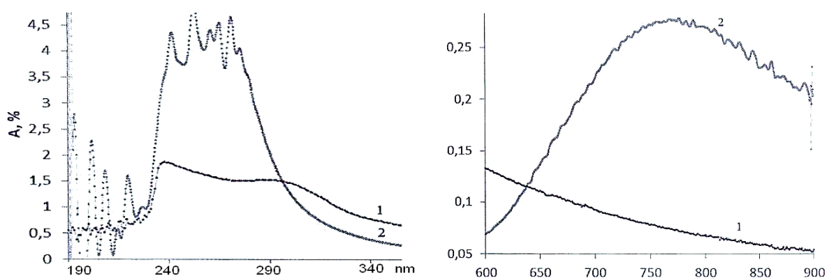
4-расм. Bombyx mori хитозани \text{X3-Cu}^{2+} металлокомплексларнинг УБ-спектрлари
