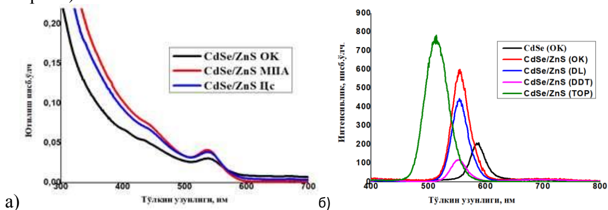
11-расм. Гибрид CdSe/ZnS (OK), CdSe/ZnS (Цс) ва CdSe/ZnS (MHA) ККНларнинг ютилиш (а) ҳамда CdSe/ZnS ККНларининг турли стабилизаторли люминесценция (б) спектрлари.
