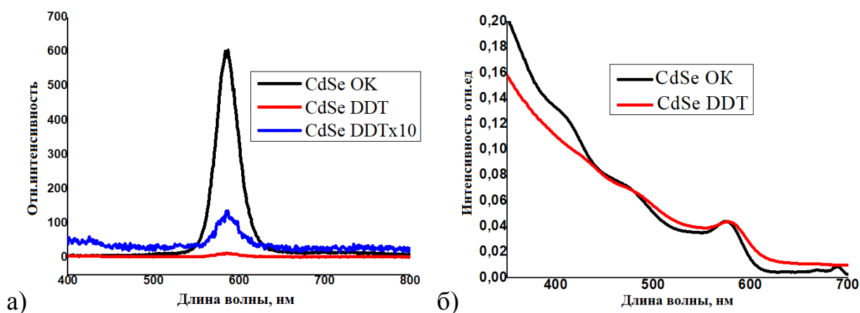
Рис.7. Спектры люминесценции (а) и поглощения (б) CdSe OK и CdSe DDT ККТ.
