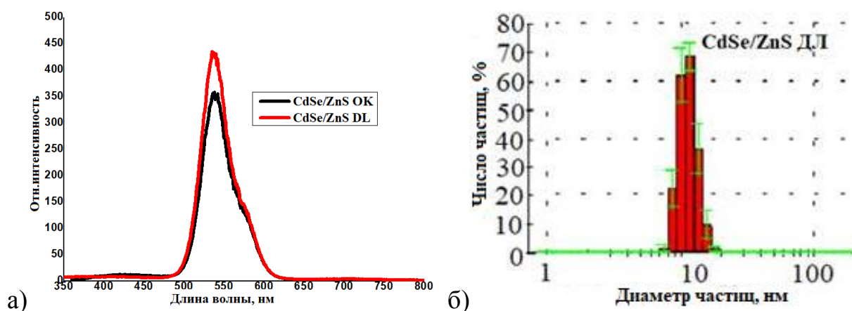
Рис.9. Спектров люминесценции CdSe/ZnS ОК (а) и CdSe/ZnS DL КТ и гистограмма среднего гидродинамического размерного распределения гибридных CdSe/ZnS DL ККТ (б).
