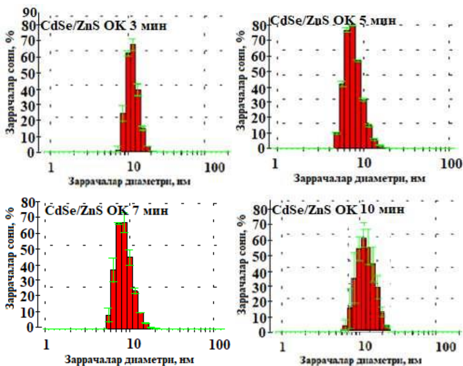
6-расм. Синтезнинг турли вақтида CdSe/ZnS (ОК) КН ларининг ўртача гидродинамик ўлчам тақсимоти гистограммалари.
