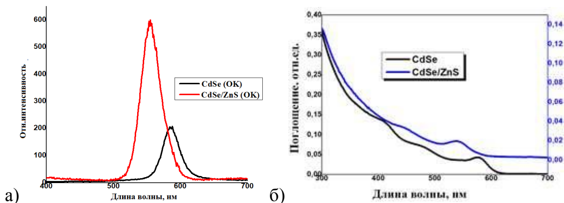
Рис.3. Спектры люминесценции (а) и поглощения (б) CdSe ОК и CdSe/ZnS ОК КТ
