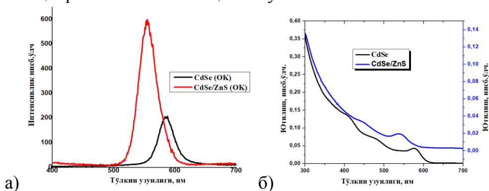
3-расм. \text{CdSe} (ОК) ва \text{CdSe/ZnS} (ОК) КН ларини люминесценция (а) ва ютилиш (б) спектрлари. Стабилизатор олеин кислота (ОК).
