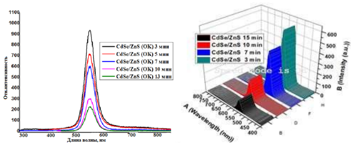
Рис.5. Люминесценция и трехмерные спектры люминесценции гибридных CdSe/ZnS ККТ (процесс синтеза проводились в разное время)
