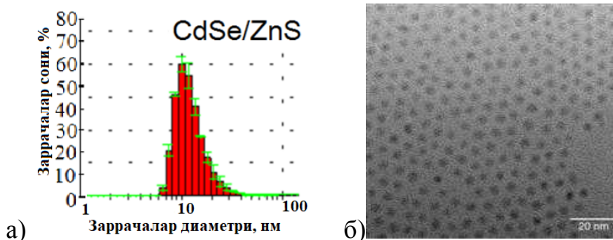
4-расм. CdSe/ZnS (ОК) КНларнинг ўртача гидродинамик ўлчам тақсимоти гистограммаси (а) ва электрон микроскоп (ТЕМ)да олинган тасвири (б)
