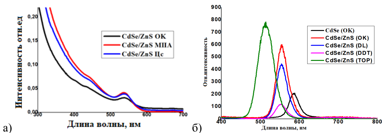
Рис.11. Спектры поглощения гибридных ККТ CdSe/ZnS (ОК), CdSe/ZnS (Цс) CdSe/ZnS (МПА) и спектры люминесценции различных стабилизаторов ККТ CdSe/ZnS.
