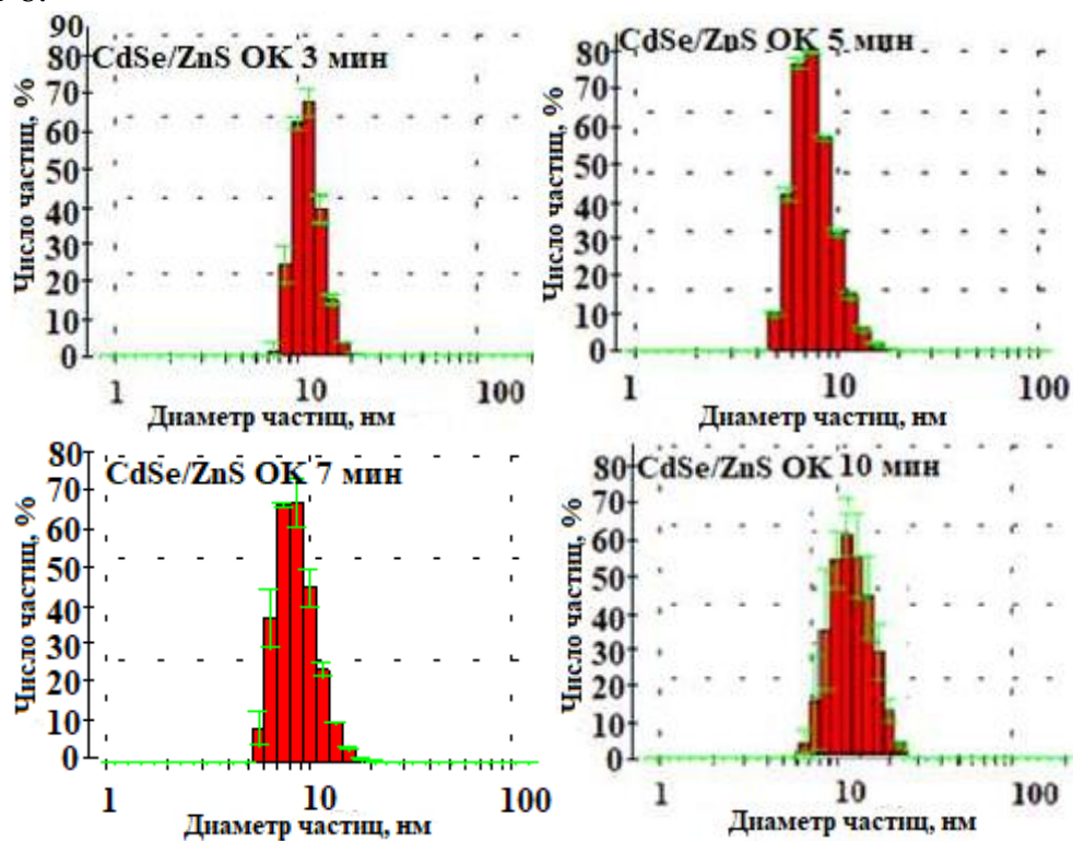
Рис.6. Среднее гидродинамическое распределение по размерам CdSe/ZnS ОК КТ в разное время синтеза.
