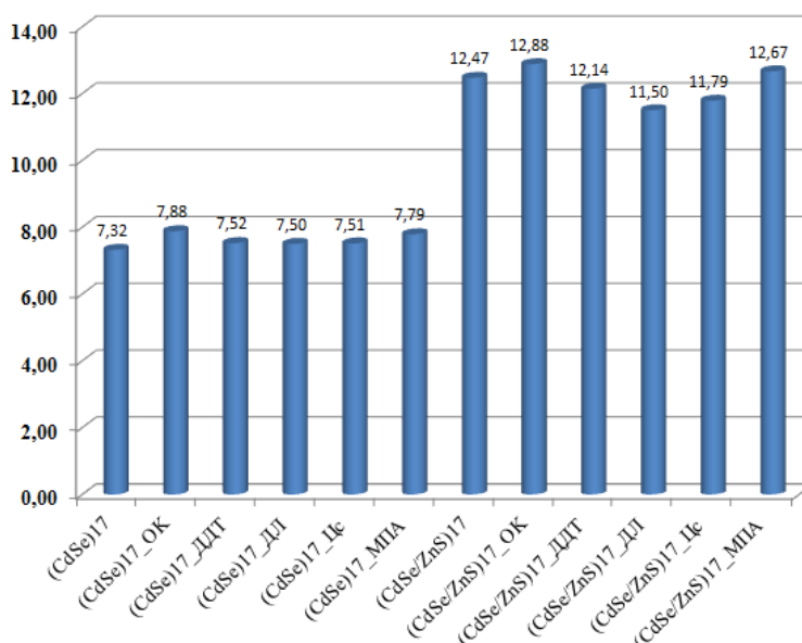
2-расм. (\text{CdSe})_{17} асосидаги квант нуқталар сирти турли стабилизаторлар билан қопланганда “электрон – тиркиш” жуфтлик энергетик даражасининг ўзгариши
