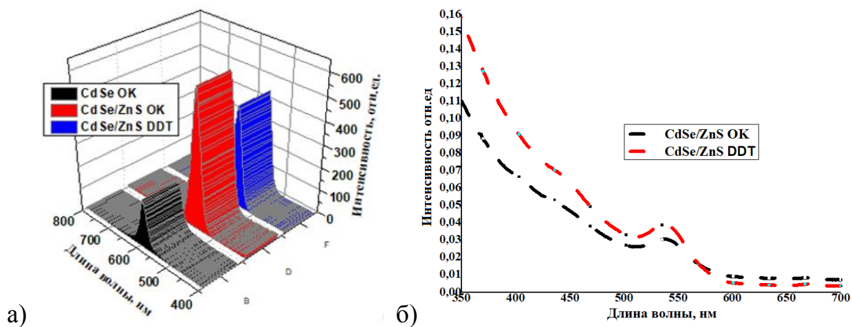
Рис.8. Трехмерные спектры люминесценции (а) и поглощения (б) CdSe OK, CdSe/ZnS OK и CdSe/ZnS DDT ККТ.
