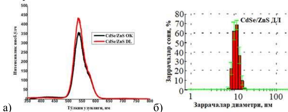
9-расм. Гибрид CdSe/ZnS (ОК) ва CdSe/ZnS (ДЛ) КҚНларнинг люминесценция спектрлари (а) ҳамда ўртача гидродинамик ўлчам тақсимоти гистограммаси (б)
