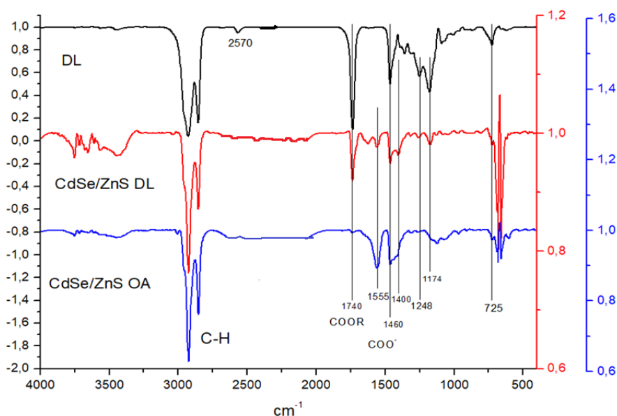
Рис.10. CdSe/ZnS ОК, CdSe/ZnS DL и додецилдигидро ИК-спектр эфира липоевой кислоты
