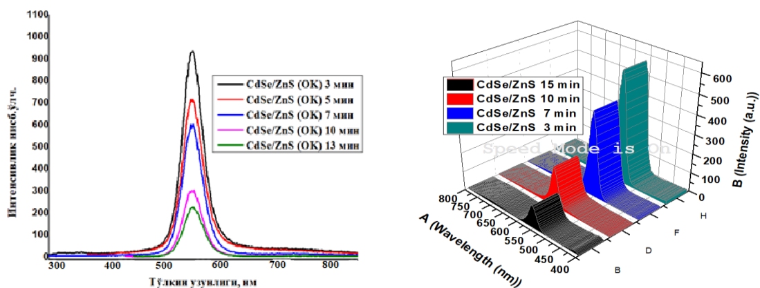
5-расм. Гибрид CdSe/ZnS ККНларнинг (турли синтез вақтидаги) люминесценция ва уч ўлчамли люминесценция спектрлари
