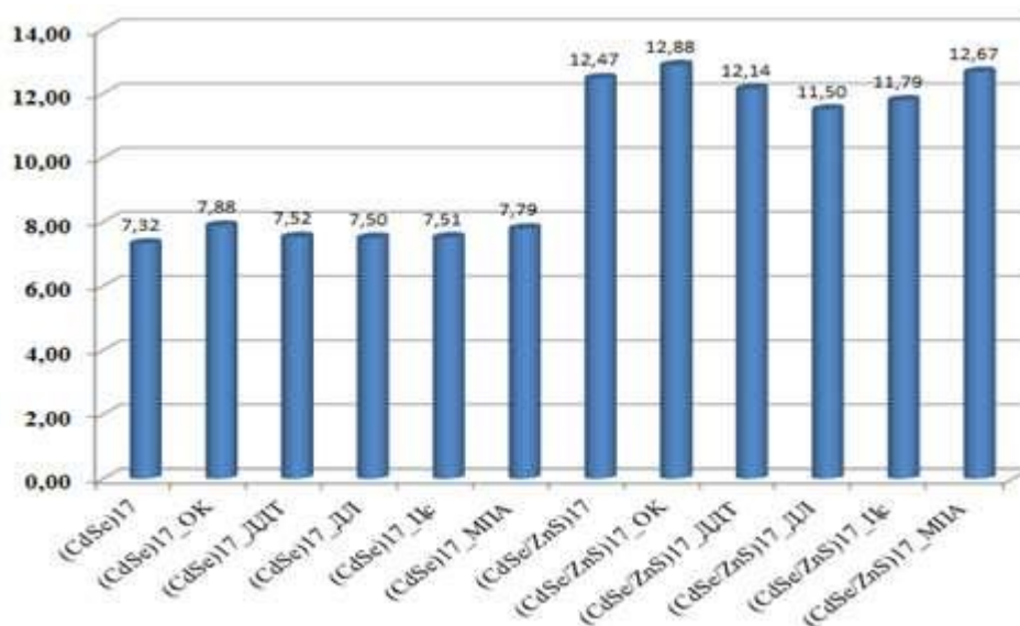
Рис 2. Изменение степени энергетических уровней пары «электронной щели» при покрытия поверхности квантовых точек (CdSe) 17 с различными стабилизаторам
