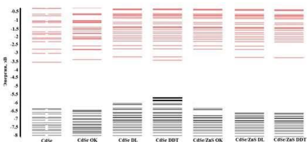
1-расм. Турли стабилизаторли кластерларнинг таъқиқланган зона кенглиги ва НОМО-ЛОМО молекуляр орбиталларнинг энергетик даражаси
