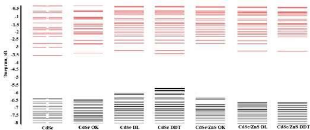
Рис.1. Ширина запрещенной зоны кластеров с различными стабилизаторами и степень энергетических уровней молекулярных орбиталей HOMO-LUMO.
