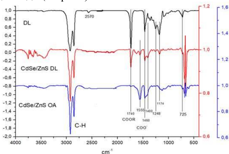
10-расм. CdSe/ZnS (ОК), CdSe/ZnS (ДЛ) ва додецилдигидро липоат кислота эфирли КҚНларнинг ИҚ спектрлари.
