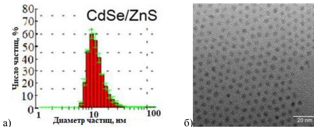
Рис.4. Гистограмма среднего гидродинамического размерного распределения CdSe/ZnS ОК КТ (а) и изображение, полученное с помощью ПЭМ (б)
