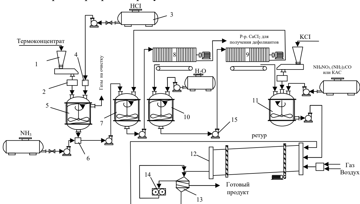
Рис. 1. Технологическая схема производства NP- и NPK- удобрений на основе мытого обожженного фосфоконцентрата, соляной кислоты, азотсодержащих компонентов и хлорида калия. 1-бункер, 2-дозатор, 3- бак, 4-расходомер, 5-реактор, 6-нейтрализатор, 7-рактор разбавления, 8- и 9-пресс фильтры, 10-репульпатор, 11-смеситель, 12-БГС, 13-сито, 14-мельница, 15-насос
