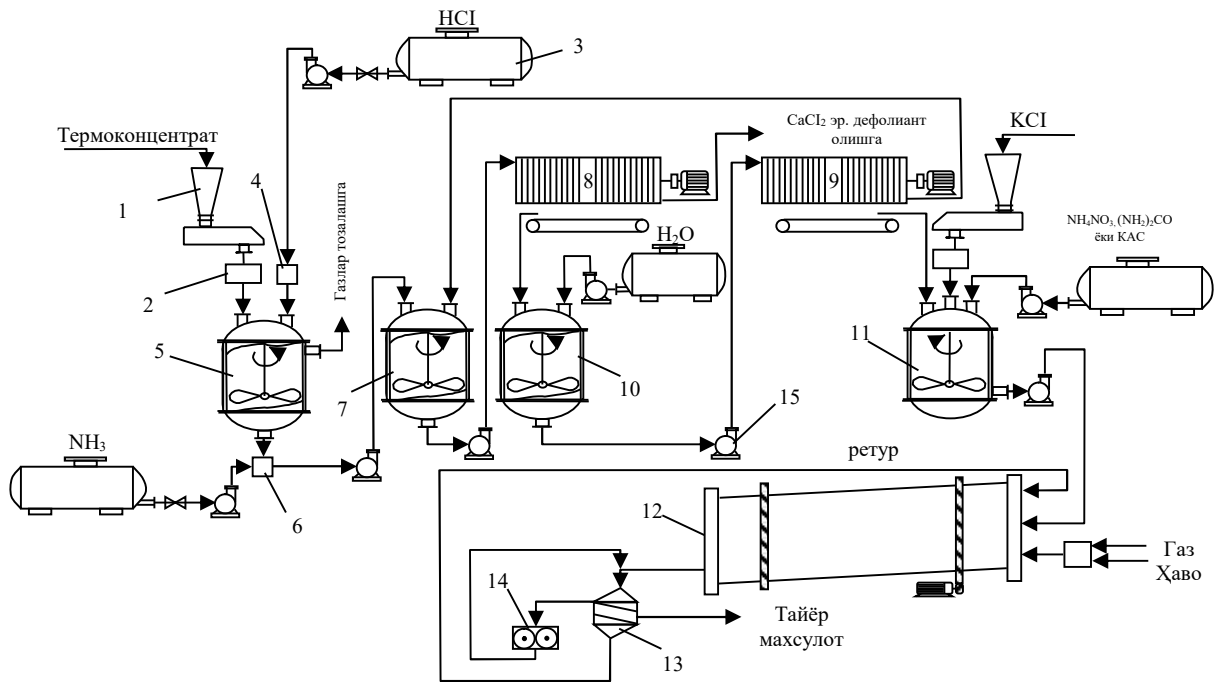
1-расм. Ювиб куйдирилган фосфо­концентрат, хлорид кислота, азот тутган компонентлар ва калий хлорид асосида NP- ва NPK-ўғитлар ишлаб чиқариш технологик схемаси. 1-бункер, 2-дозатор, 3- бак, 4-сарф ўлчагич, 5-реактор, 6-нейтрализатор, 7-суялтиргич, 8- ва 9-пресс филтр, 10-репульсатор, 11-аралаштиргич, 12-БДҚ, 13-элак, 14-тегирмон, 15-насос.
