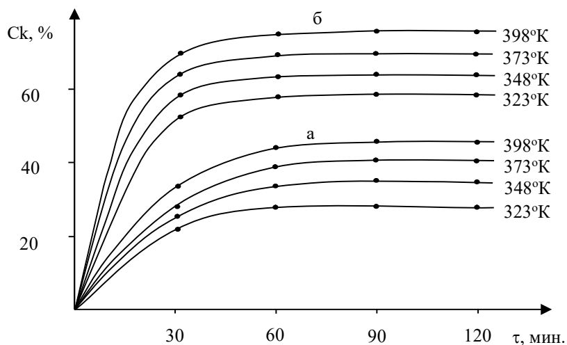
Рис. 2. Зависимость степени конверсии хлорида кальция с хлоратом натрия от температуры и продолжительности процесса. С выпаркой (а) и без выпарки (б) конверсионных растворов.
