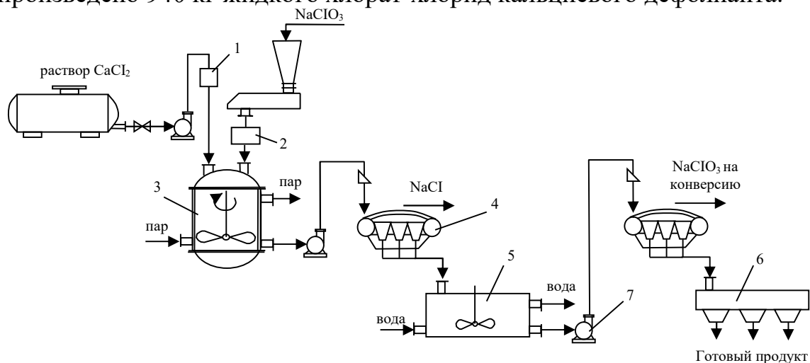
Рис.3. Технологическая схема получения жидкого хлорат-хлорид кальциевого дефолианта. 1-расходомер, 2-дозатор, 3-реактор для синтеза дефолианта, 4-вакуум-фильтр, 5-кристаллизатор, 6-затаривающее устройство, 7-центробежный насос.
