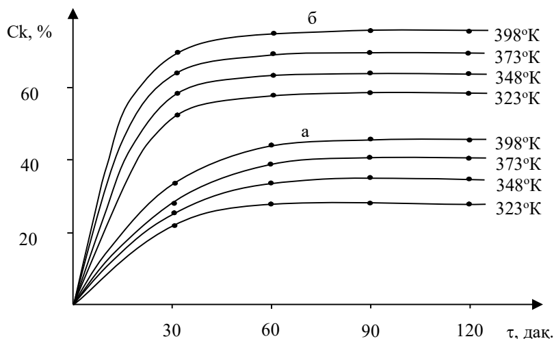
2-расм. Кальций хлориднинг натрий хлорат билан борадиган конверсия жараёнидаги конверсия даражасининг ҳарорат ва вақтга боғлиқлиги. Конверсион эритма: а-буғлатилмаган ҳолда; б- буғлатилган ҳолда.
