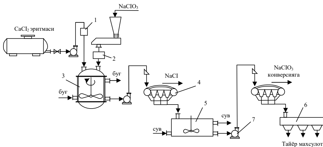
3-расм. Суюқ кальций хлорат-хлоридли дефолиант олишнинг технологик схемаси. 1-сарф ўлчагич, 2-дозатор, 3-дефолиант синтези учун реактор, 4-вакуум филтр, 5-кристаллизатор, 6-қадоклаш қурилмаси, 7-марказдан қочма насос.
