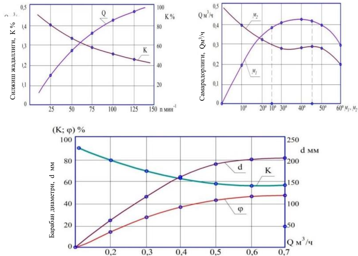
2-Расм. Қурилма унумдорлигининг ( Q ) ва аралаштириш интенсивлигининг ( K ) валнинг – қурилма шнекининг айланиш сонига (а) ва аралаштириш интенсивлигига ( K ), тўлдирма даражасига ( \phi ), барабан диаметрига ( d ) (б), тўғри ( \mu_1 ) ва тескари ( \mu_2 ) силжитадиган (в) парракларнинг қиялик бурчагига боғлиқлиги
