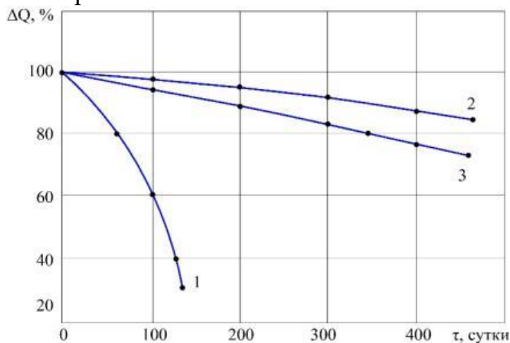
Рис. 6. Зависимость производительности насосов от срока эксплуатации без покрытия и с покрытием
