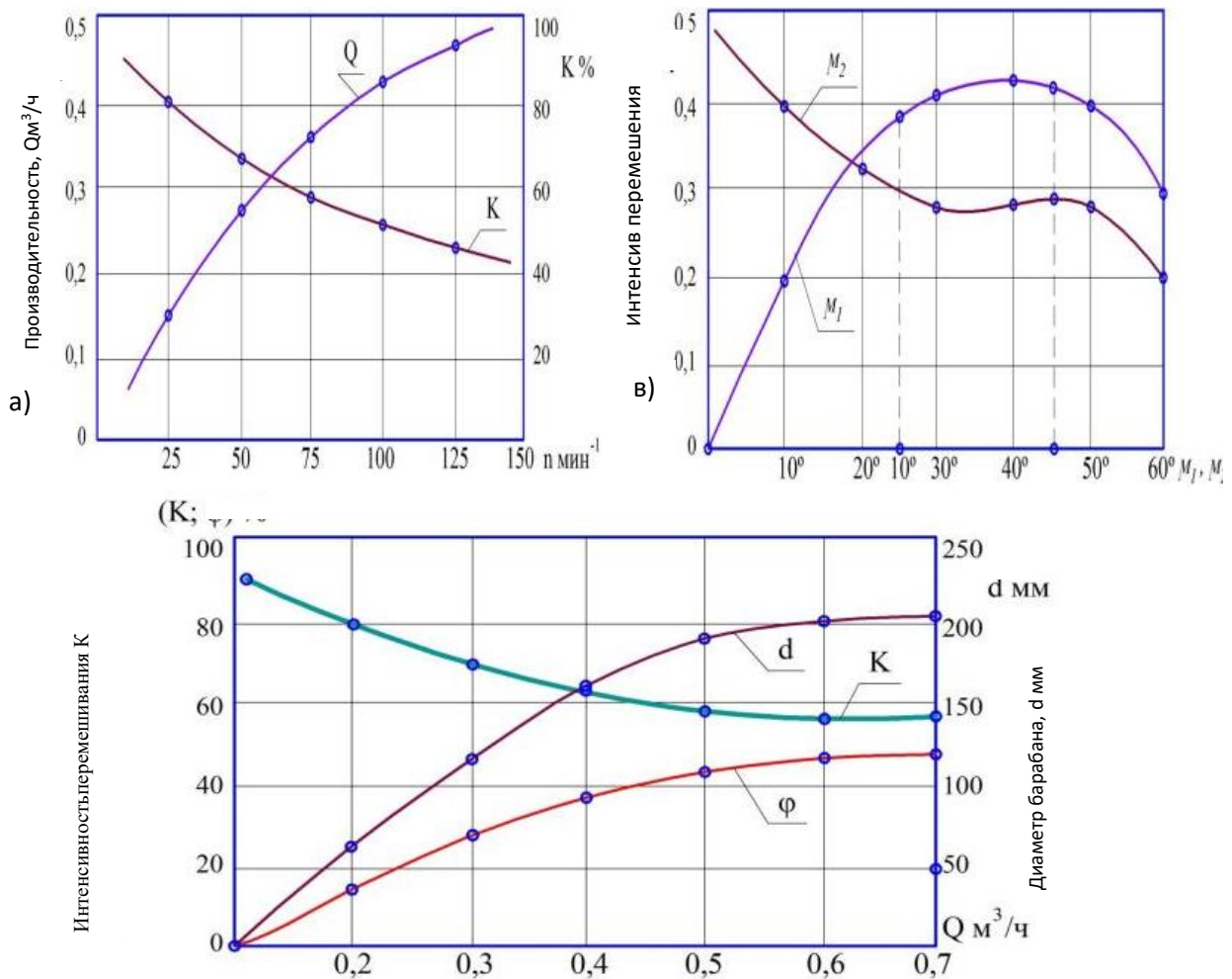
Рис. 2. Зависимость производительности установки (Q) и интенсивности перемешивания (K) от числа оборотов вала – шнека установки (а) и от интенсивности перемешивания (K), степени заполнения (φ) и диаметра барабана (d) (б), от угла наклона лопастей прямого ( \mu_1 ) и обратного ( \mu_2 ) хода (в)
