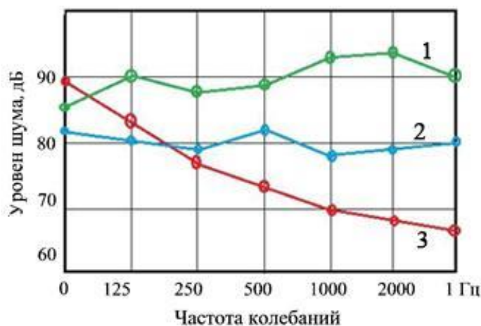
Рис. 5. Уровни звукового давления джина УМПД в Букинском и Пскентском хлопкоочистительном заводе
