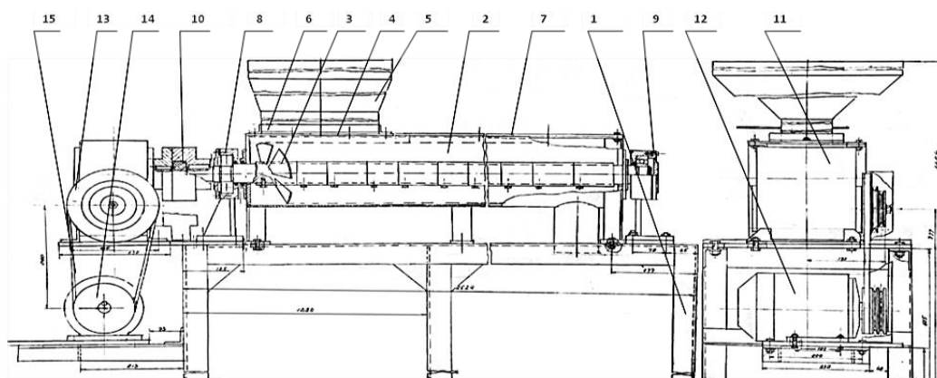
1-рама, 2-барабан, 3-шнек, 4-бункер қопқоғи, 5-секцияли бункер, 6-тақсимлагич, 7-барабан қопқоғи, 8,9-кронштейнлар, 10-муфта, 11-редуктор, 12-электр двигател, 13,14-шківлар, 15-тўқимачилик материалдан тайёрланган тасма
