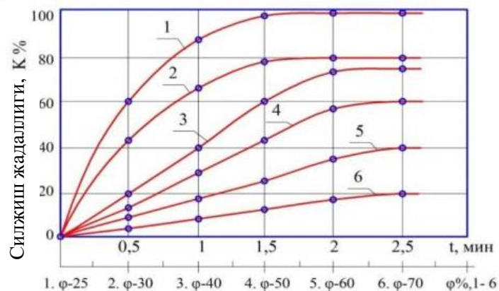
1 – Расм. Аралаштириш жадаллигини аралаштириш вақтига (t) ва шнекли аралаштиргич қурилмада турли миқдордаги арлашмани тўлдириш (φ) даражасига боғлиқлиги
