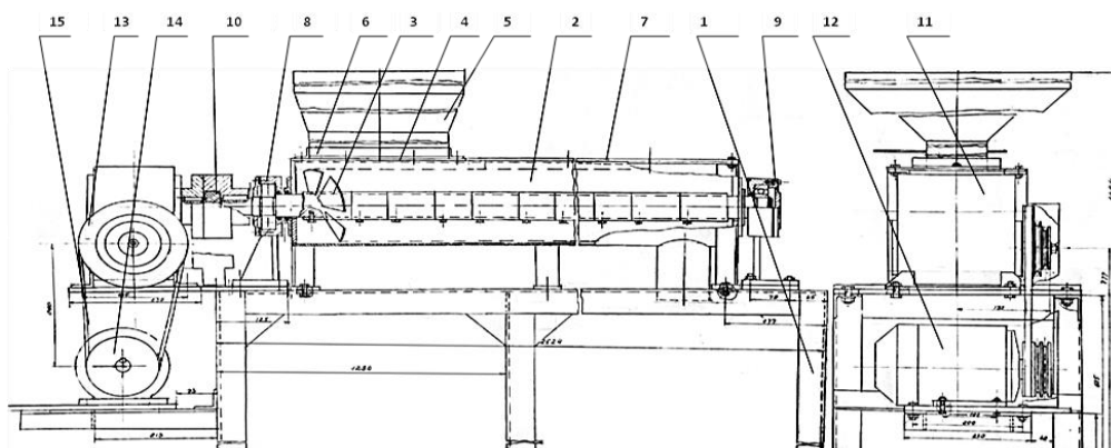
1-рама, 2-бункер, 3-шнек, 4-крышка бункера, 5- бункер секционный, 6-заслонки, 7-крышка из оргстекла, 8,9-кронштейны, 10-муфта, 11-редуктор, 12-электродвигатель, 13,14-шкивы, 15- текстильный ремень
