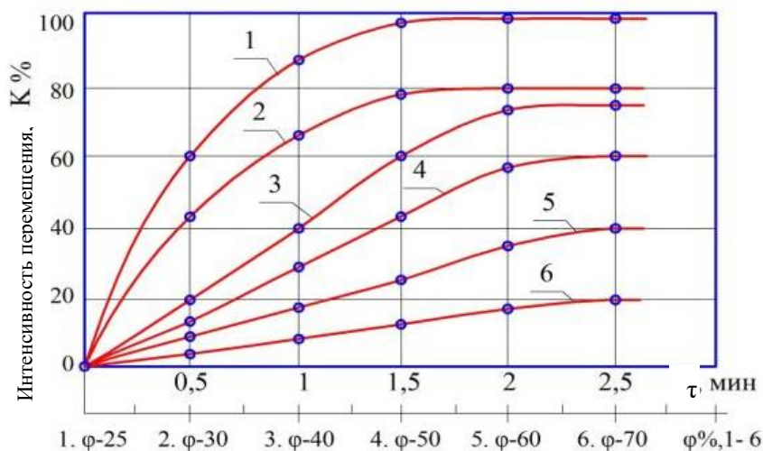
Рис. 1. Зависимость интенсивности перемешивания от времени перемешивания \tau и степени заполнения \phi смесительной шнековой установки при различных значениях заполнения
