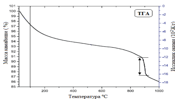
7-расм. ААО ғовакли мембранасининг ТГА таҳлил натижаси
