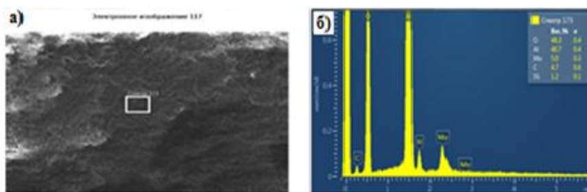
Рисунок 12. Результаты СЭМ (а) и ЭДС (б) анализа пористой нанокompозитной системы Ni-Mo/Al 2 O 3
