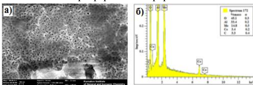
Рисунок 13. Результаты СЭМ (а) и ЭДС (б) анализа пористой нанокompозитной системы Co-Mo/Al 2 O 3
