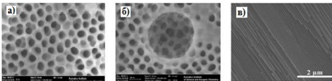
1-расм. Икки босқичли анодланган алюминий пластинкасининг СЭМ натижалари: а,б) устки томондан ва в) ён томондан кўриниши
