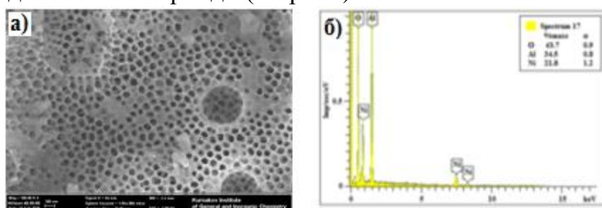
11-расм. Ni/Al 2 O 3 ғовакли нанокомпозит системанинг СЭМ (а) ва ЭДС (б) таҳлил натижалари
