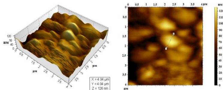
Рисунок 8. Результаты АСМ анализа АОА мембраны
