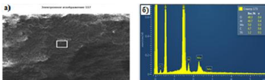
12-расм. Ni-Mo/Al 2 O 3 ғовакли нанокомпозит системанинг СЭМ (а) ва ЭДС (б) таҳлил натижалари
