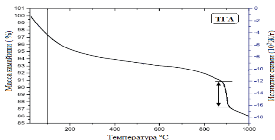
Рисунок 7. Результаты ТГА анализа АОА мембраны
