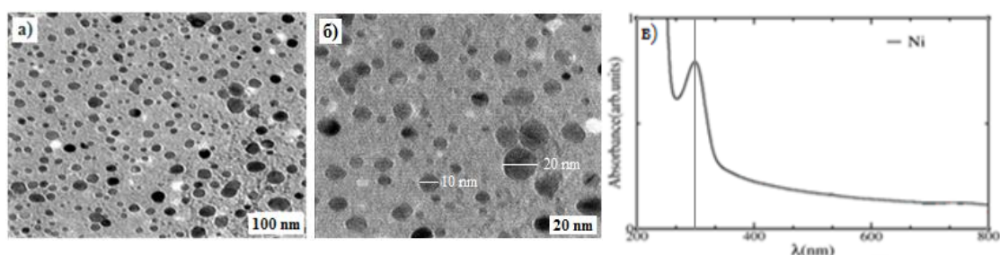
Рисунок 9. ПЭМ а) 100 нм, б) 20 нм и в) УФ-спектральные результаты наночастицы Ni полученные с экстрактом амаранта
