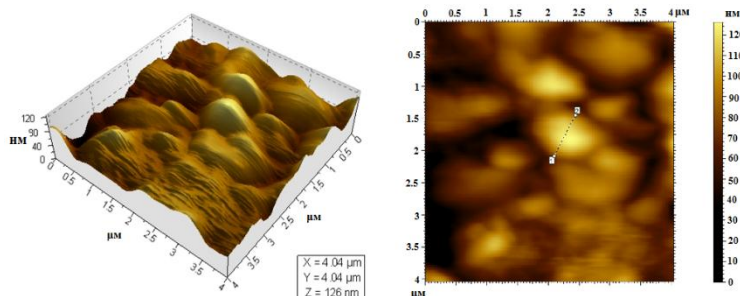
8-расм. ААО ғовакли мембранасининг АСМ таҳлил натижалари
