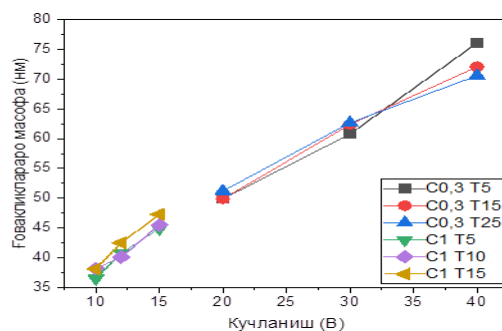
Рисунок 4. Зависимость расстояния между порами мембраны АОА от концентрации электролита, температуры и напряжения
