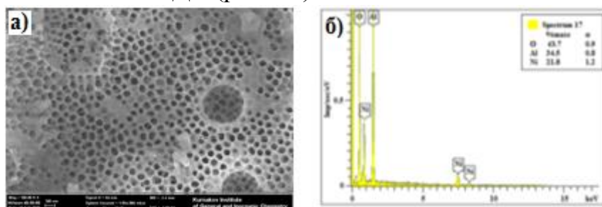
Рисунок 11. Результаты СЭМ (а) и ЭДС (б) анализа пористой нанокондитной системы Ni/Al 2 O 3
