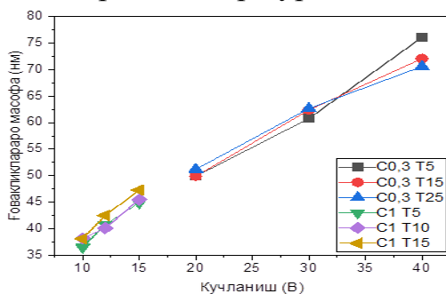
4-расм. ААО мембранаси ғовакликлараро масофасининг электролит концентрацияси, ҳарорат ва кучланишга боғлиқлиги
