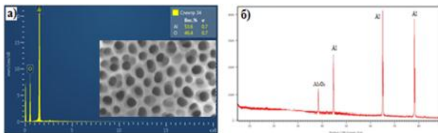
Рисунок 2. СЭМ-ЭДС (а) двухступенчатых анодированных пористых мембран и результаты рентгеноструктурного анализа (б)
