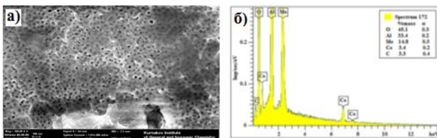
13-расм. Co-Mo/Al 2 O 3 ғовакли нанокомпозит системанинг СЭМ (а) ва ЭДС (б) таҳлил натижалари
