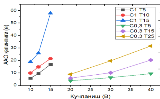
5-расм. ААО мембранаси оксид қатлам қалинлигининг электролит концентрацияси, ҳарорат ва кучланишга боғлиқлиги
