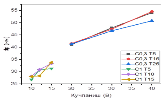
3-расм. ААО мембранасидаги ғовакликлар диаметрининг электролит концентрацияси, ҳарорат ва кучланишга боғлиқлиги
