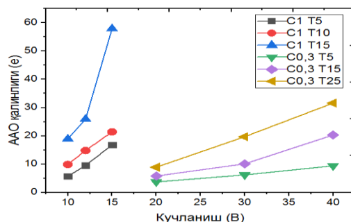
Рисунок 5. Зависимость толщины оксидного слоя мембраны АОА от концентрации, температуры и напряжения электролита
