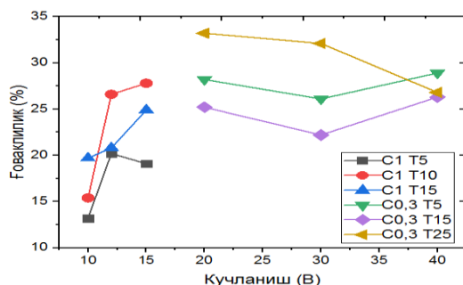
6-расм. ААО мембранаси ғоваклилик даражасининг электролит концентрацияси, ҳарорат ва кучланишга боғлиқлиги
