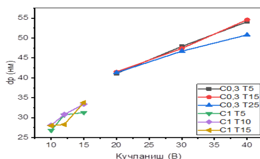
Рисунок 3. Зависимость диаметра пор на мембране АОА от концентрации электролита, температуры и напряжения
