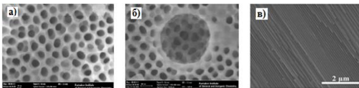
Рисунок 1. Результаты СЭМ двухэтапной анодированной алюминиевой пластины: а,б) вид сверху и в) вид сбоку
