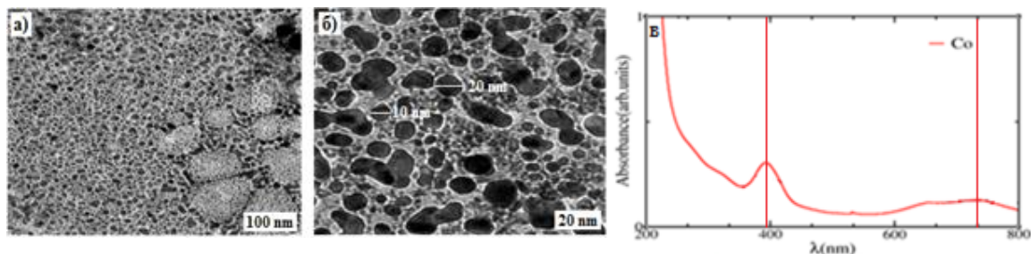
10-расм. Амаранта экстракти билан олинган Co нанозаррачаларининг ТЭМ а) 100 нм, б) 20 нм ва в) УБ- спектр натижалари
