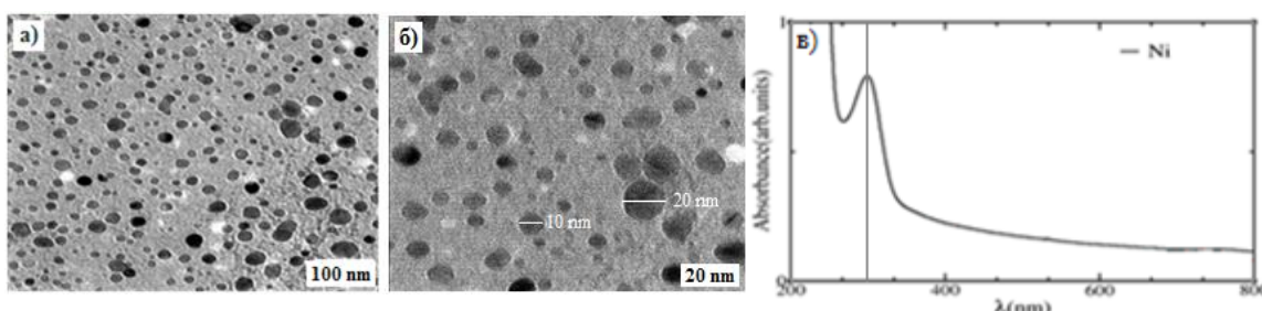
9-расм. Амаранта экстракти билан олинган Ni наноэраччаларининг ТЭМ а) 100 нм, б) 20 нм ва в) УБ- спектр натижалари
