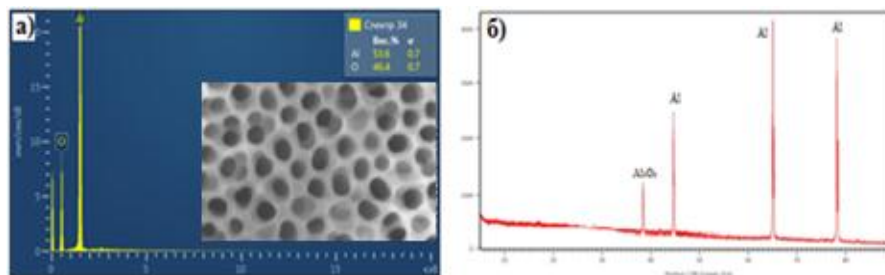
2-расм. Икки босқичли анодланган ғовакли мембраналарнинг СЭМ-ЭДС (а) ва XRD анализ (б) натижалари
