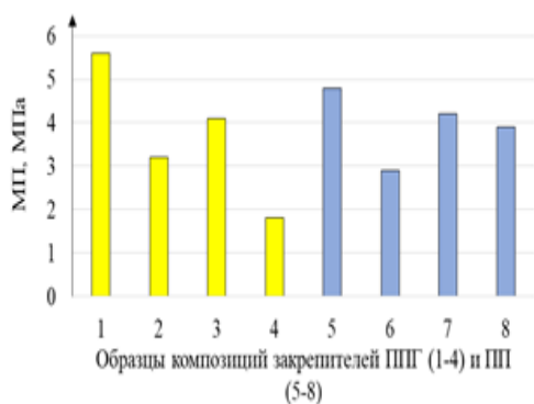
Рис. 3. Влияние состава композиций закрепителей на механическую прочность получаемых корок
