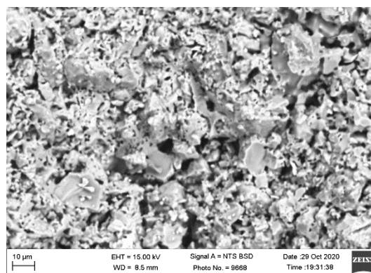
Рисунок 6. Электронно-микроскопические снимки образцов КГП-17 (а) и КГФ-14 (б)
