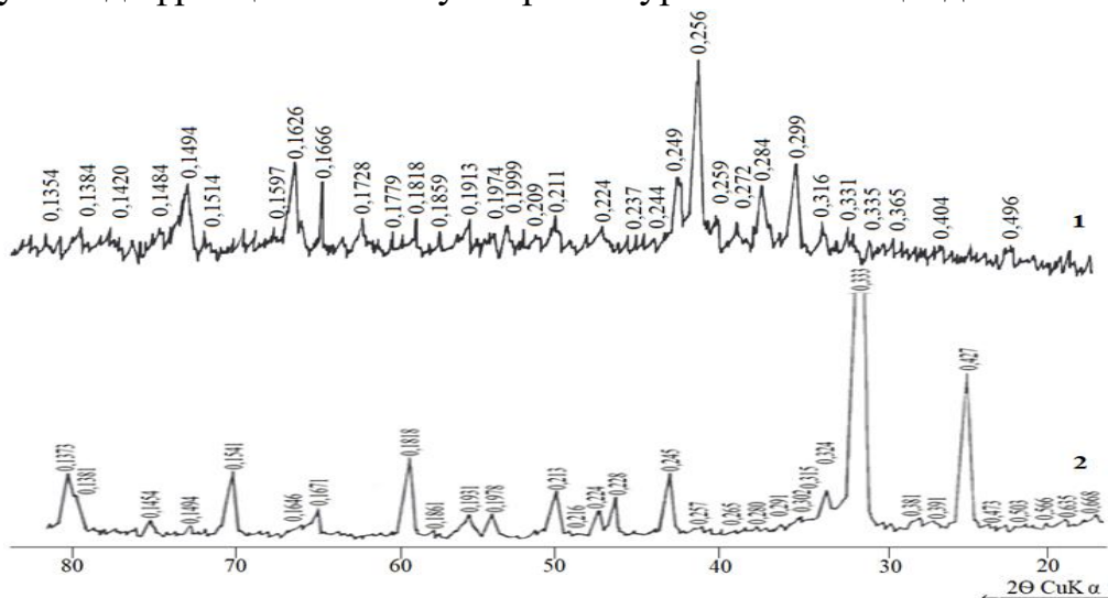
1-расм. ГТЧ (1) ва ФФБ (2) чиқиндилари намуналарининг рентгенограммалари
