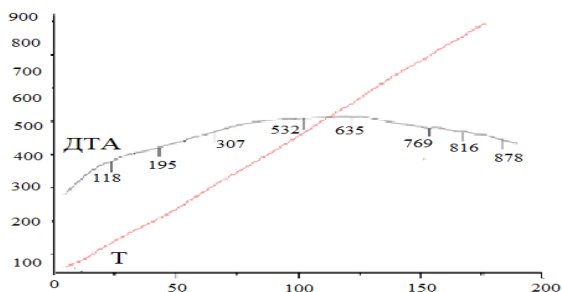
2-расм. Газни тозалаш чанги намунасининг дифференциал термик эгри чизиқлари.
