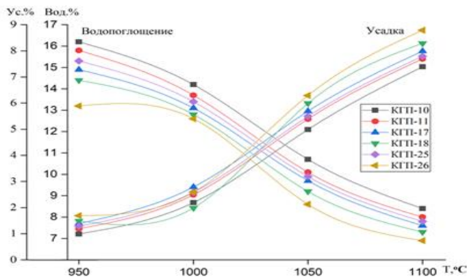
Рисунок 4. Влияние железо-содержащей пыли газоочистки на основные технологические характеристики керамической массы
