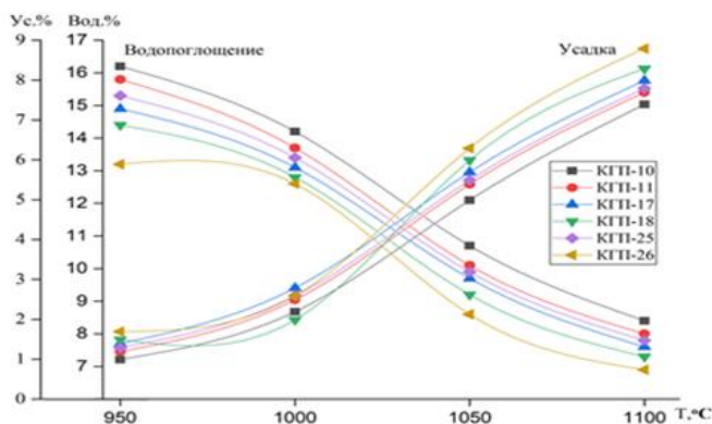
4-расм. Газни тозалаш темир таркибли чангининг керамик массанинг асосий технологик хусусиятларига таъсири
