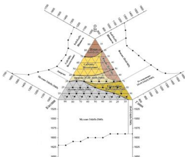
3-расм. Иккиламчи политемик кесимли «каолин-гил-ГТЧ» учламчи системанинг эриш диаграммаси
