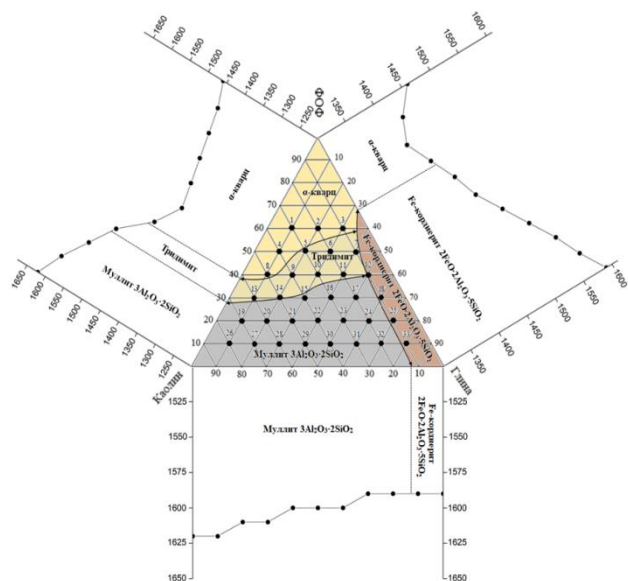
5-расм. “Каолин-глина-ГТЧ” учламчи системасининг иккилам-чи политермик кесимлари билан эриш диаграммаси
