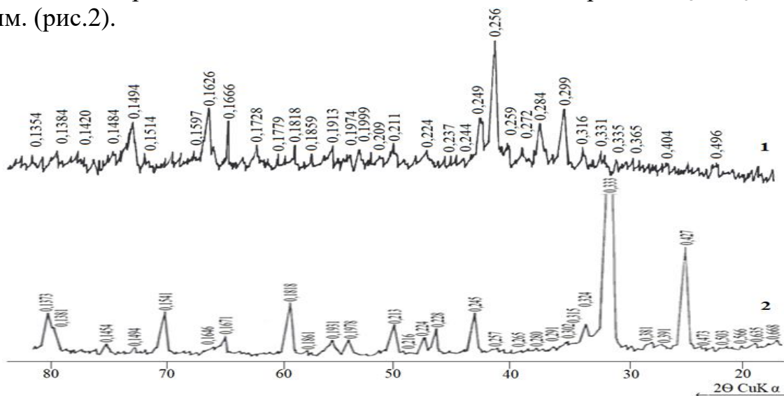
Рисунок 1. Рентгенограммы образцов отходов ПГО (1) и ФОФ (2)
