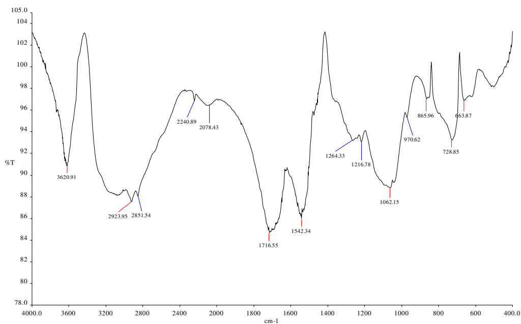
Рис .7. ИК спектр комплекса кадмия с МАК кислотой иммобилизованной на волокне СМА-1.
