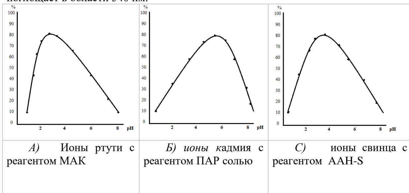
Рис. 3. Зависимость степени сорбции от кислотности раствора
