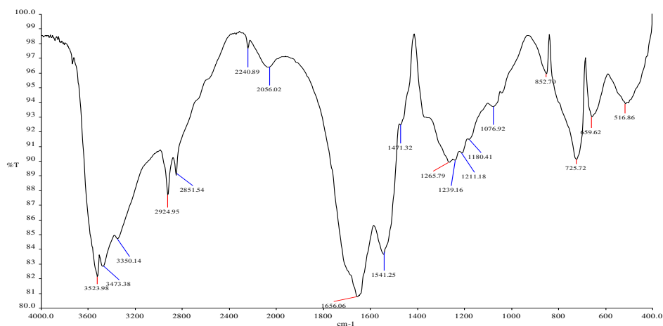
Расм 6. Имобилланган МАК кислота реагентининг ИК-спектри
