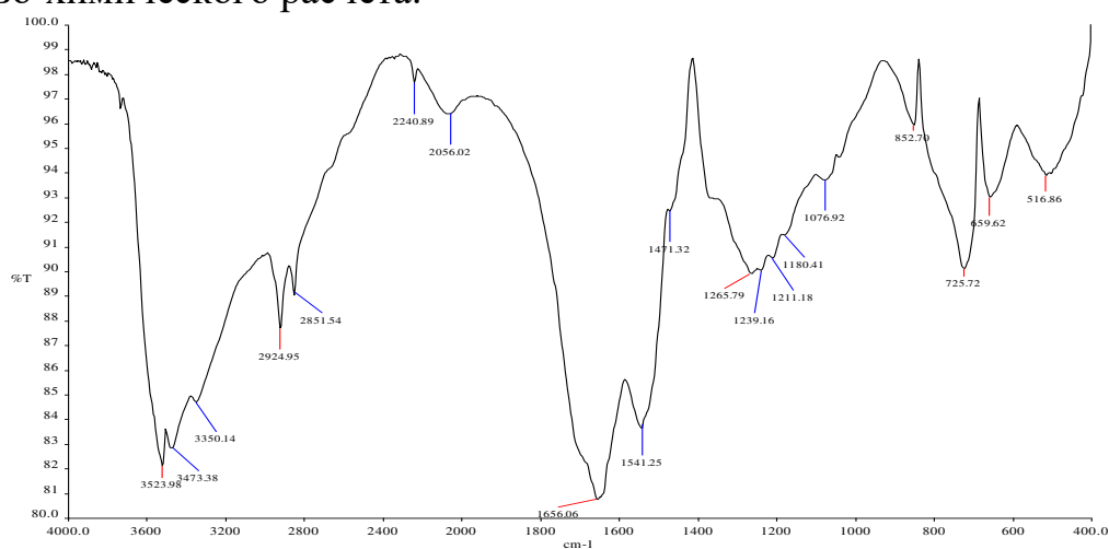
Рис 6. ИК спектры иммобилизованной МАК кислоты
