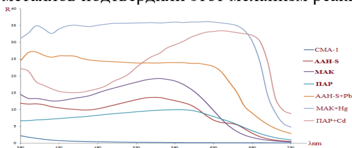
Рис.5. Спектры отражения иммобилизованных реагентов с ионами свинца кадмия и ртути.
