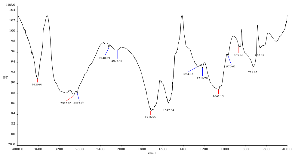
Расм 7. СМА-1 толасига имобилланган МАК реагентини кадмий ионини билан комплексининг ИК-спектри
