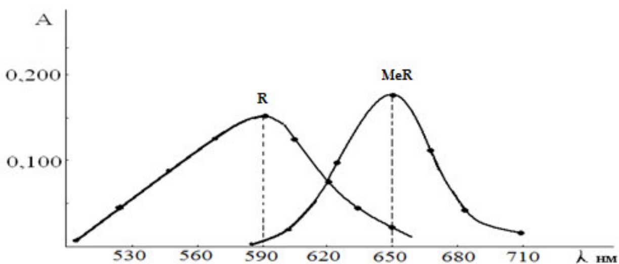
Рис.1. Спектры поглощения реагента ПАР соли и его комплекса с ионами Cd 2+
