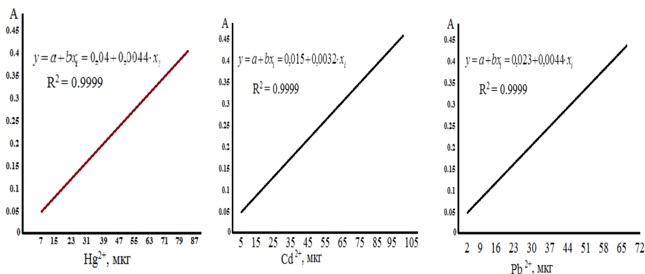
Рис.10. Градуировочные графики определения ионов свинца, кадмия и ртути с использованием иммобилизованных МАК, PAR соли и ААН-S соответственно.
