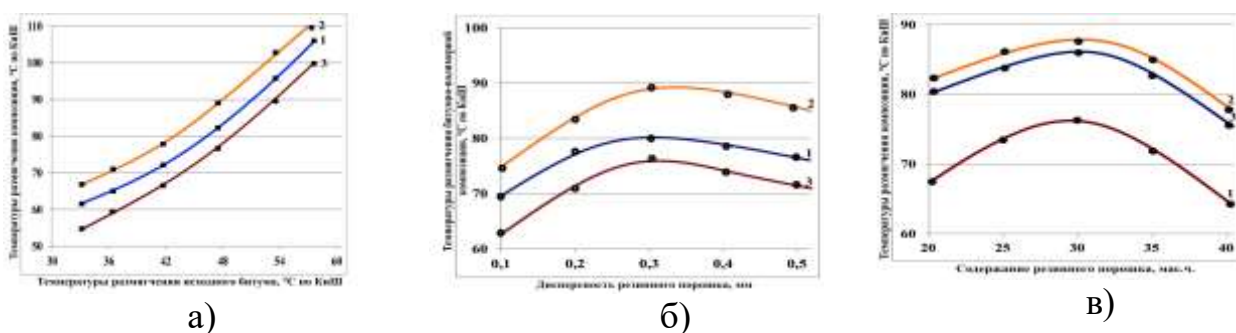
Рис.1. Зависимость температуры размягчения битумно-полимерной композиции от температуры размягчения исходного битума (а) дисперсности (б) и содержания (в) резинового порошка при различном наполнении резиновым порошком
