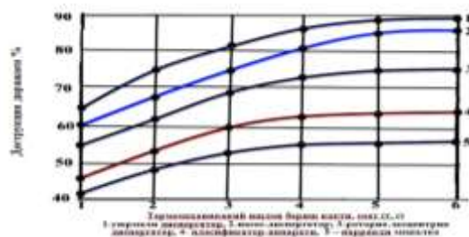
3-расм. Диспергатор (а) ва парракли аралаштиргичда (б) термомеханик ишлов беришда битумнинг дастлабки ўзгаришига Тр га боғлиқ равишда деструкция даражасининг ўзгариши
