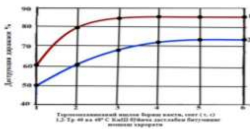
3-расм. Диспергатор (а) ва парракли аралаштиргичда (б) термомеханик ишлов беришда битумнинг дастлабки ўзгаришига Тр га боғлиқ равишда деструкция даражасининг ўзгариши
