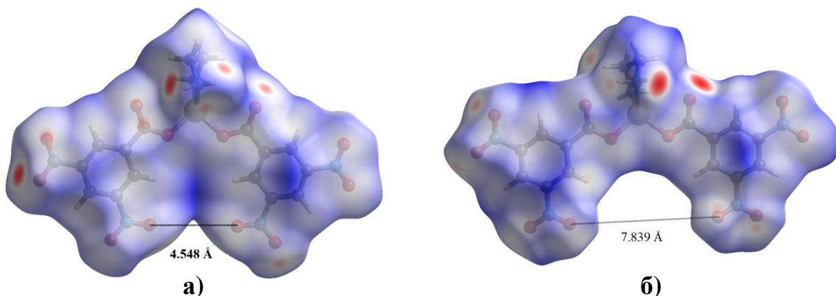
Рисунок 7. Поверхности Хиршфельда моноклинного (а) и орторомбического (б) полиморфа комплекса [Zn(ДНБК)_2(ЭДА)] .
