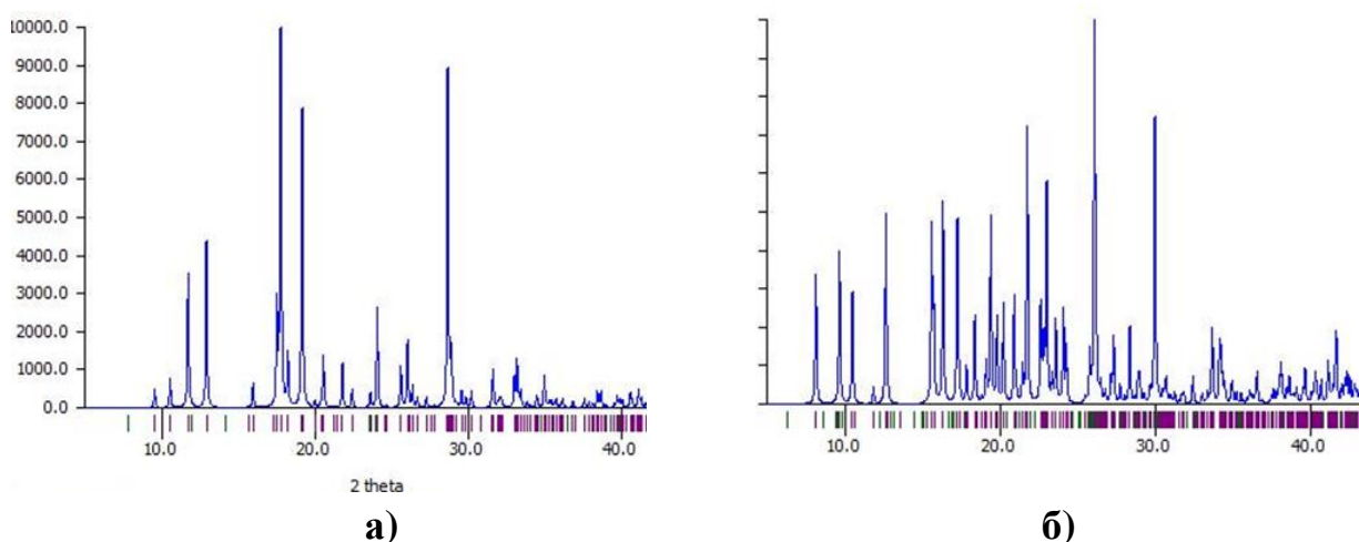
Рисунок 5. Дифрактограммы моноклинного (а) и орторомбического (б) полиморфа комплекса [Zn(ДНБК)_2(ЭДА)] .
