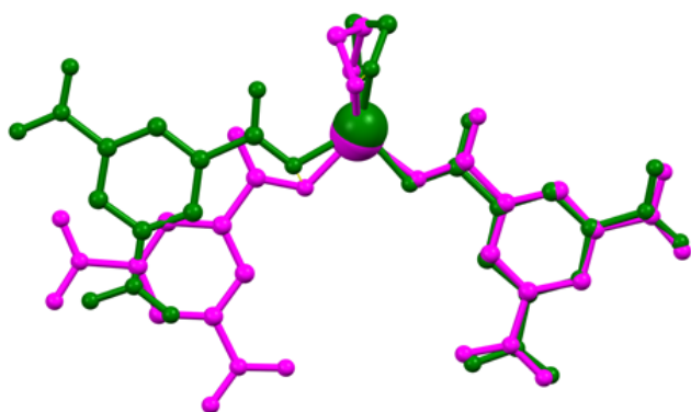
Рисунок 6. Разница в конформации комплексных молекул в моноклинном (розовый) и орторомбическом (зеленый) полиморфах комплекса [Zn(ДНБК)_2(ЭДА)] .
