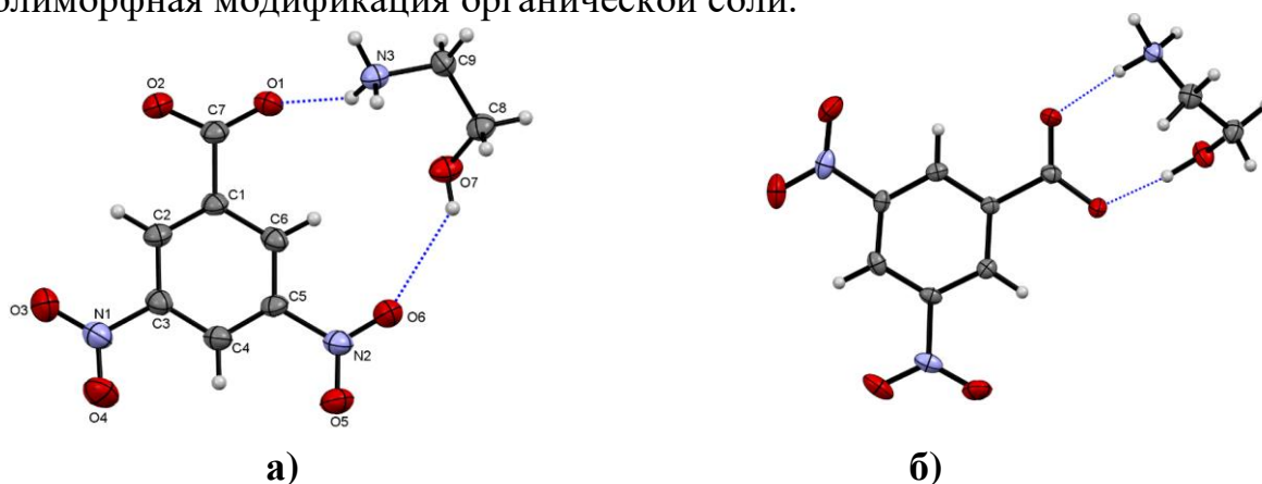
Рисунок 1. Асимметричная часть элементарной ячейки органической соли (ДНБК - ·МЭА + ): новый моноклинный полиморф, полученный в настоящей работе (а) и известный орторомбический полиморф с ref-кодом ICIMOX (б). Эллипсоиды тепловых колебаний неводородных атомов нарисованы с вероятностью 30%.
