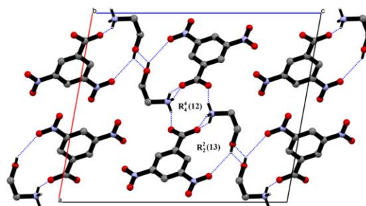
Рисунок 2. Упаковка молекул в кристаллах соли ДНБК - ·МЭА + .
