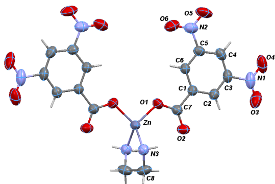
Рисунок 4. Строение комплексной молекулы в моноклинном полиморфе соединения [Zn(DNBK)_2(EDA)] .
