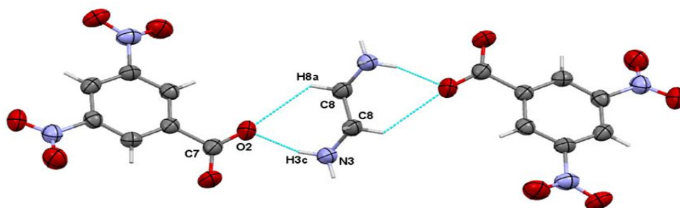
Рисунок 3. Ассоциация анионов с катионами в органической соли ДНБК - ·ЭДА + .
