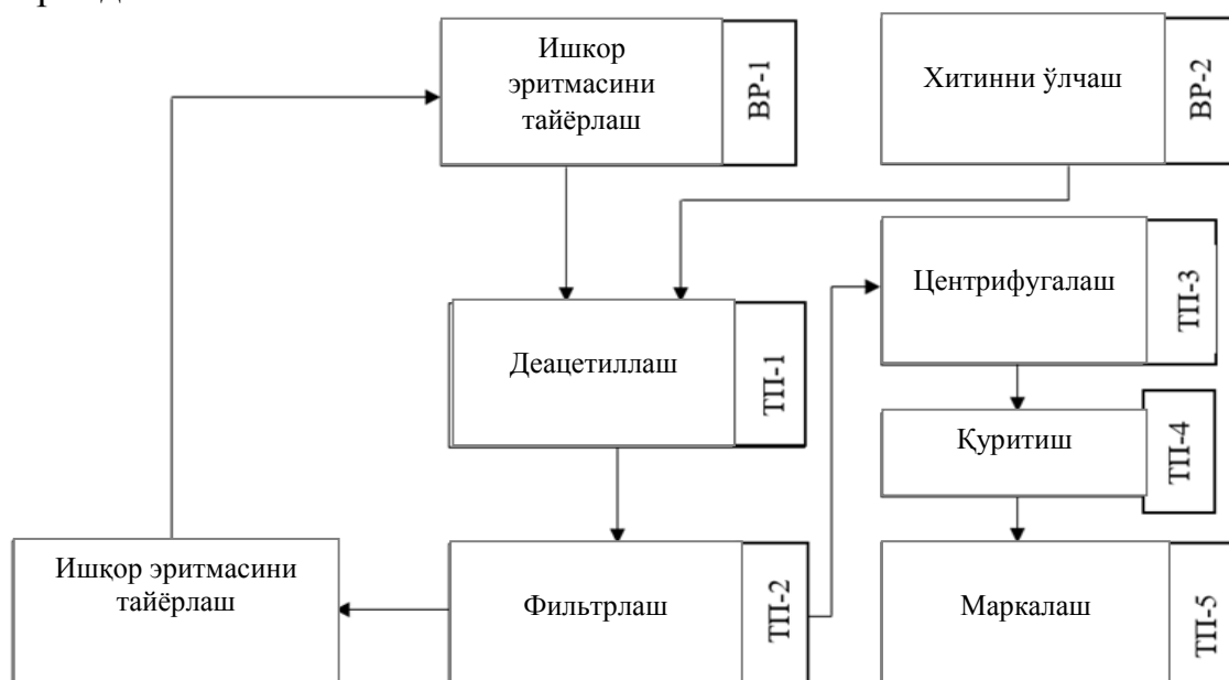
5-расм. Хитозанни ажратиш олиш технологик схемаси
