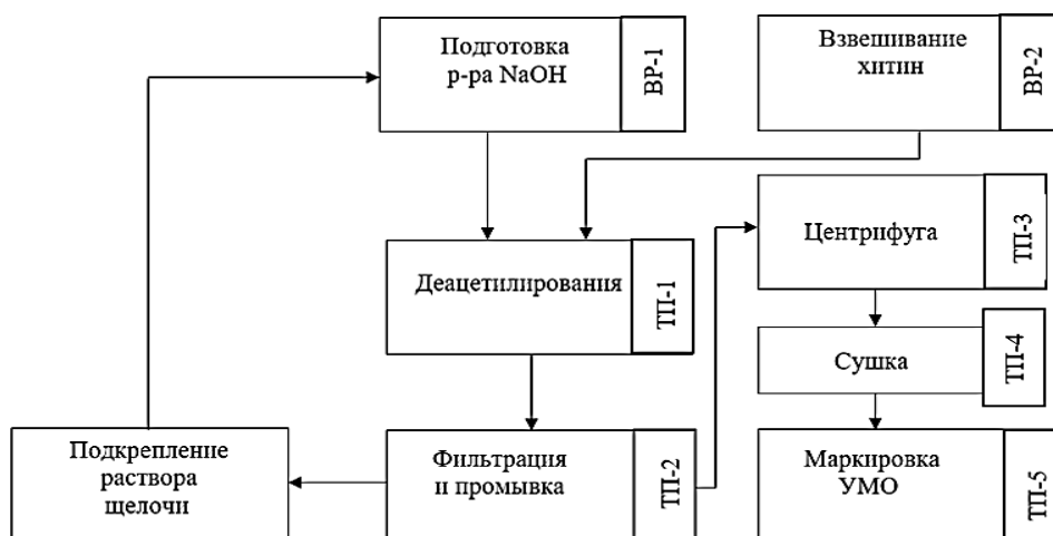
Рис. 5. Схема технологии выделения хитозана
