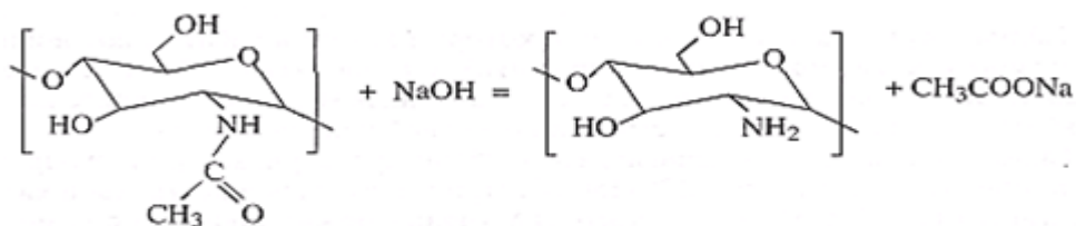
Рис. 1. Реакция образования хитозана с помощью щелочной деацетилирования хитина
