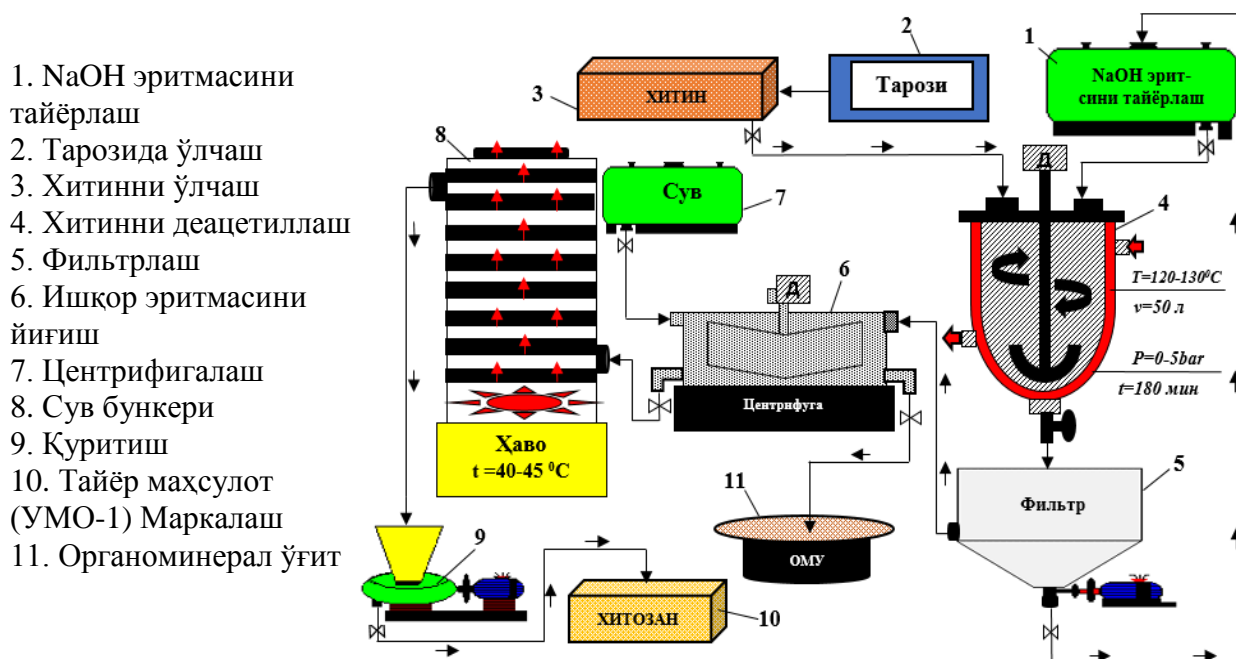
2-схема. Хитозан ишлаб чиқаришнинг технологик схемаси
