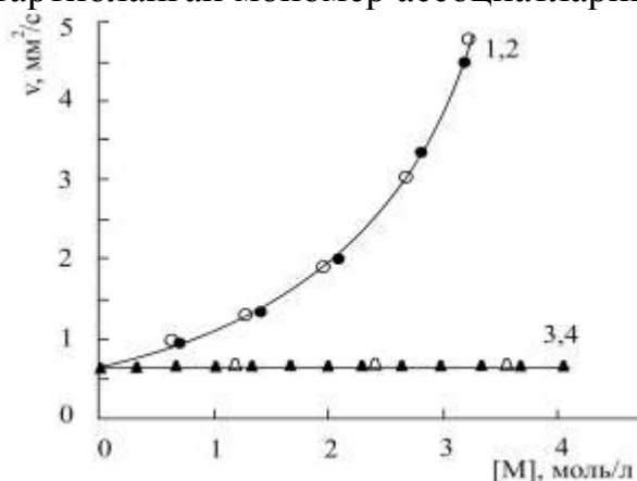
4-расм. Кинематик қовушқоқликнинг ( \nu , mm^2/s ) ПМА(1), СМА(2), ЛМА(3), ОМА(4) ларнинг бензолдаги эритмалари учун мономерлар концентрациясига ( [M] , мол/л) боғлиқлиги. Ҳарорат 20 °С.
