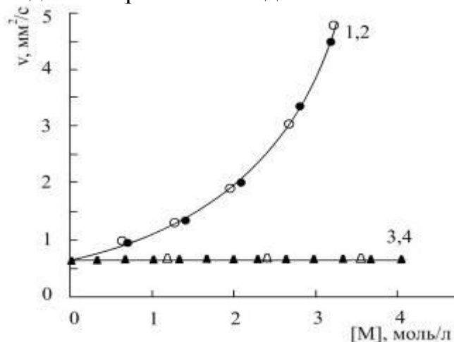
Рис. 4. Зависимость кинематической вязкости ( v, mm^2/c ) от концентрации мономеров ( [M], mole/l ) для бензоловых растворов ПМА(1), СМА(2), ЛМА(3), ОМА(4). Температура 20^0C .
