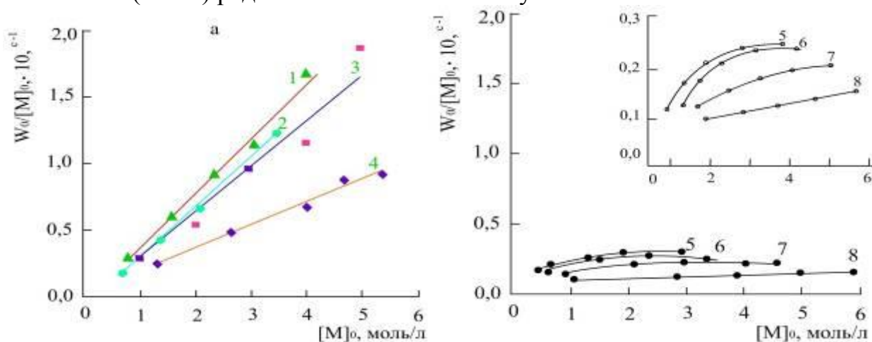
Рис. 3. Влияние начальной концентрации мономеров ( [M]_0 , моль/л) на приведенную скорость гомополимеризации алкилакрилатов (а) и алкилметакрилатов (б) в бензоле ( W_0/[M]_0, c^{-1} ): 1-ПА, 2-СА, 3-ЛА, 4-ОА, 5-ПМА, 6-СМА, 7-ЛМА, 8-ОМА
