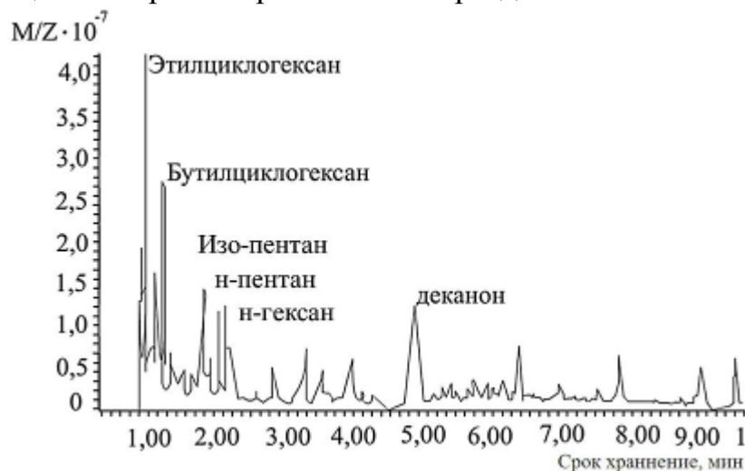
Рис. 1. Хромато-масс-спектропия жидкой фракции вторичного сырья для производства полиэтилена.
