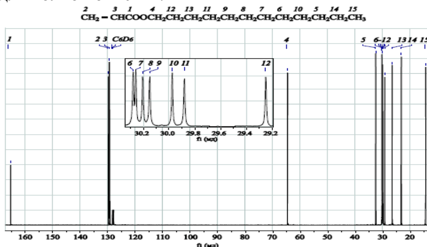
Рис. 5. ЯМР 13 С спектр додецилакрилата в C 6 D 6 (концентрацией 80% мас., 2.8 моль/л)
