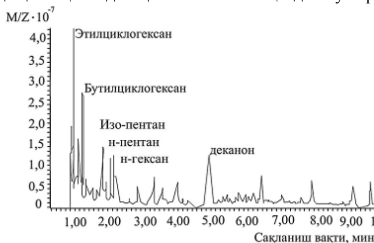
1-расм. Полиэтилен ишлаб чиқариш иккиламчи хом-ашёси суюқ фракцияни хромато-масс-спектроскопияси
