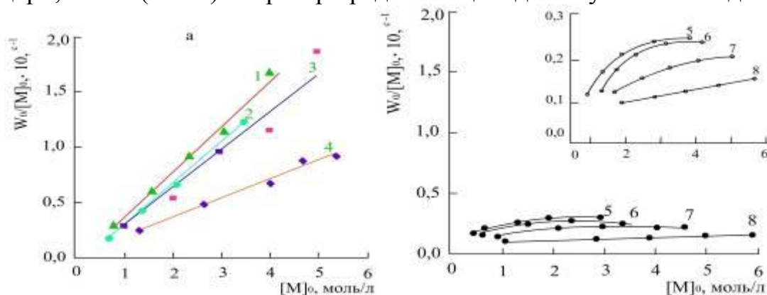
3-расм. Мономерлар бошланғич концентрацияси ( [M]_0 , мол/л) нинг бензолда алкилакрилатлар (а) ва алкилметакрилатлар (б) гомополимерланишининг келтирилган тезлиги ( W_0/[M]_0 , s^{-1} ) га таъсири: 1-ПА, 2-СА, 3-ЛА, 4-ОА, 5-ПМА, 6-СМА, 7-ЛМА, 8-ОМА
