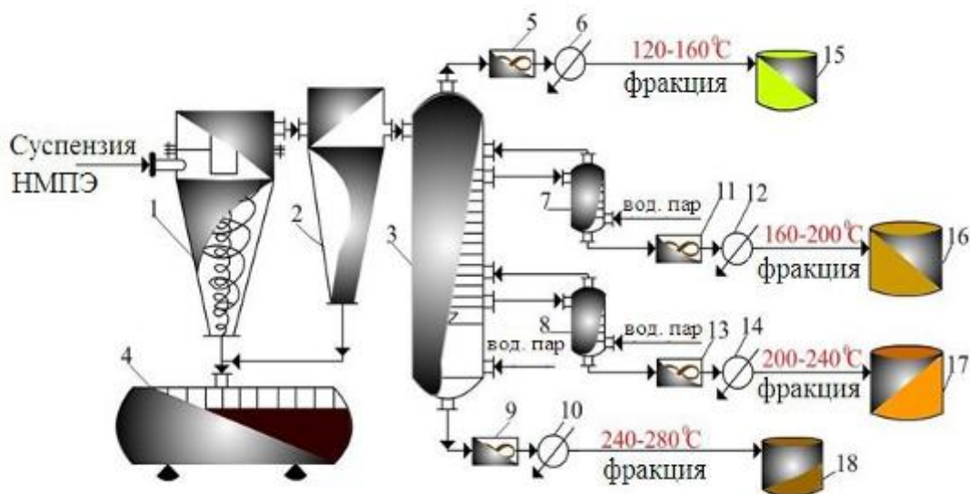
Рис. 2. Технологическая схема центрифугирования НМПЭ, сушки и ректификации жидких фракций: 1,2–циклоны, 3–ректификационная колонна, 4–фильтр, 5,9,11,13–воздушные охладители, 6,10,12,14–водяные охладители, 7,8–дефлегматоры, 15,16,17,18–сборники
