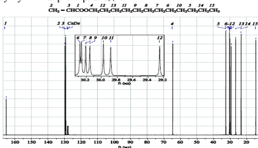
5-расм. C_6D_6 да додецилакрилатнинг ЯМР ^{13}C спектри (концентрацияси 80 % мас., 2.8 мол/л)
