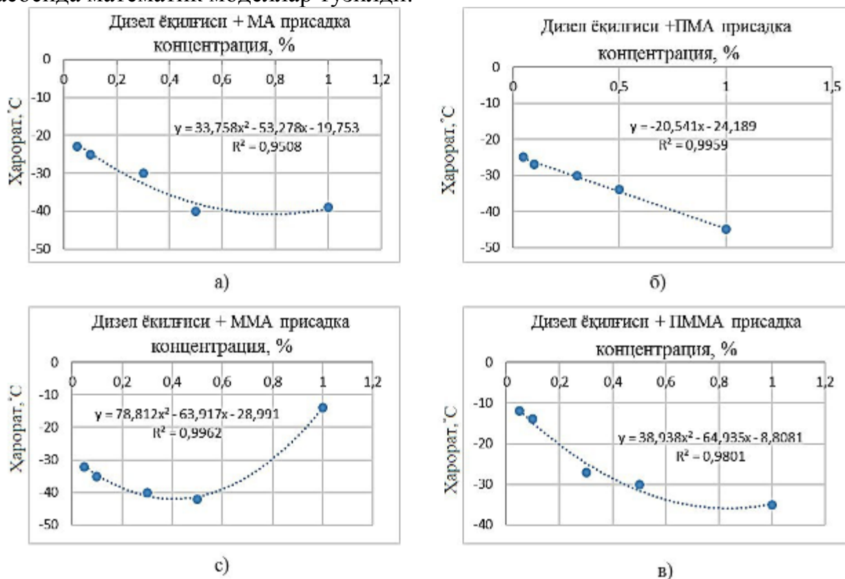
6-расм. Присадкалар бўйича тажриба нуқталари ва уларга мос регрессия тенгламалари, детерминация коэффициентлари: а-ДЁ ва МА, б-ДЁ ва ПМА, с-ДЁ ва ММА, в-ДЁ ва ПММА.
