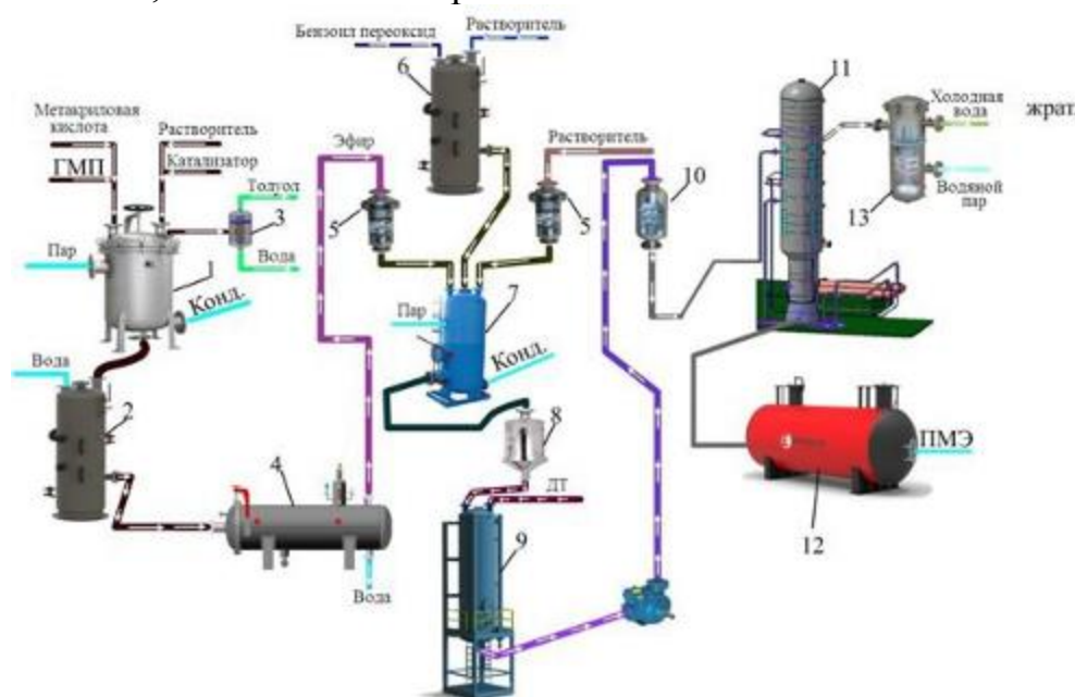
Рис 7. Технологическая схема системы получения депрессорно- диспергирующих присадок с поли(мет)акрилатами: 1 - этерификатор, 2-нейтрализатор, 3, 13-холодильник-сепаратор, 4-сепаратор, 5-дозатор, 6, 9-смеситель, 7-полимеризатор, 8-осадитель, 10-фильтр, 11-испаритель, 12-ёмкость для готового продукта, 13-холодильник-сепаратор.
