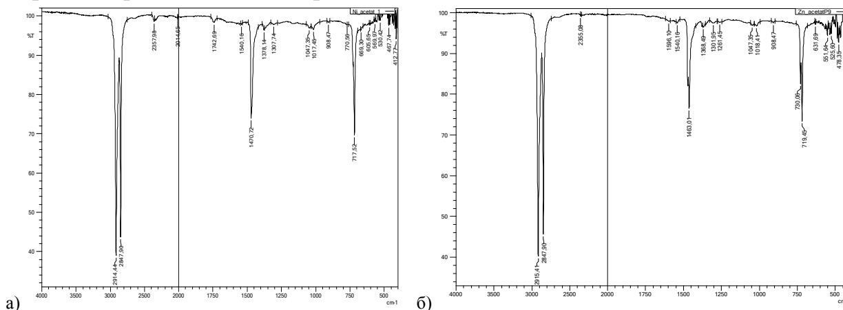
7-расм. а) ПЭ + Ni ацетат 3,0 %; б) ПЭ + Zn ацетат 3,0 %. ИҚ спектрида кўриниши.
