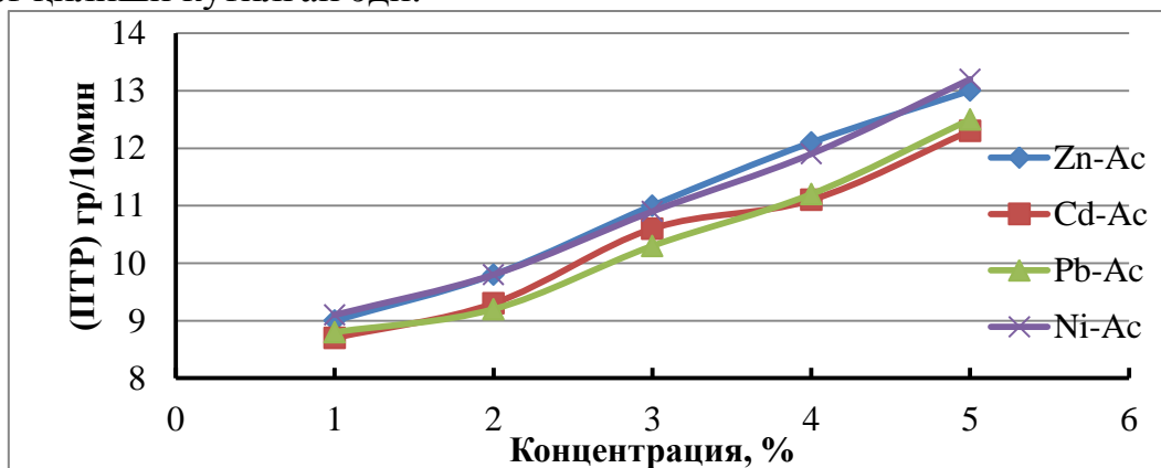
1 - расм. СОК (ПТР) нинг модификатор концентрациясига боғлиқлиги.
