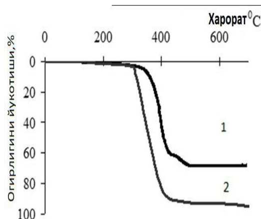
б 1 - ПП + 3,0 % қўрғошин (II) ацетат; 2 - намуна ПП J350 ТГА натижалари композитлари термограммаси.
