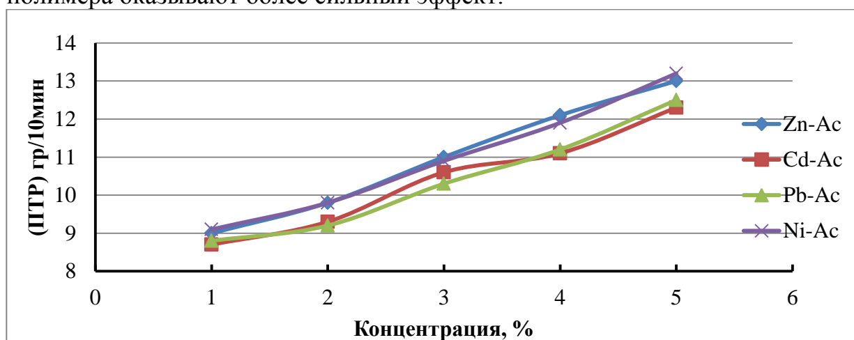
Рис. 1. Зависимость (ПТР) от концентрации модификатора.
