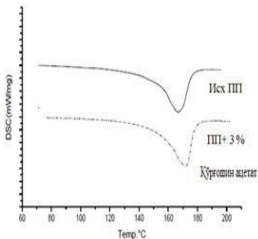
а 3-расм. а) 3,0 % металл ацетатлар билан модификацияланган ПП композитлари термограммаси
