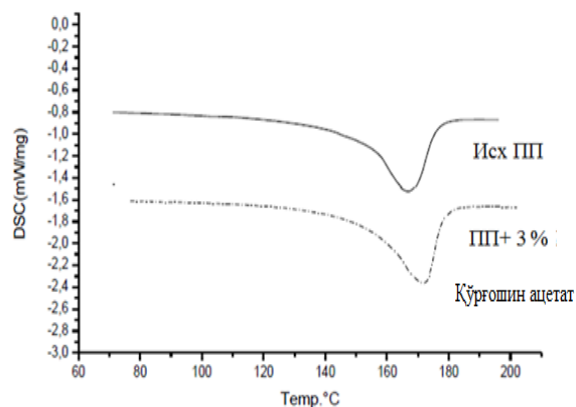
Термограмма модифицированных композитов ПП с 3,0 % ацетатами металлов.
