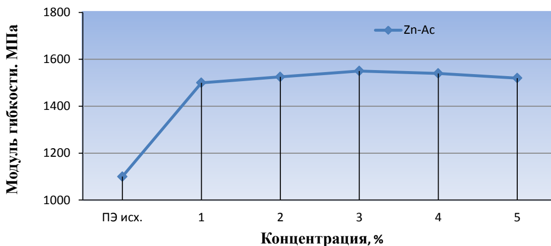
Рис. 2. Композиты от а) зависимости модуля упругости к значению модификатора
