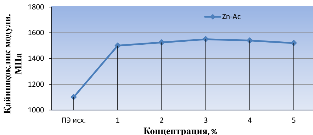
2-расм. Композитларнинг қайишқоқлик модулининг модификатор миқдорига боғлиқлиги.
