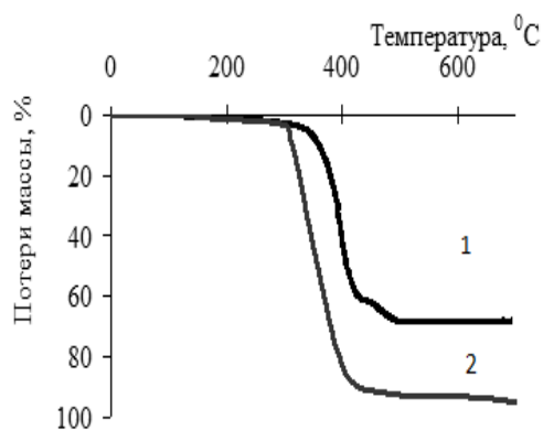
Рис. 3. 1 - ПП+3,0 % ацетат свинца; 2-исх ПП J350 Термограмма композитов результатов ТГА.
