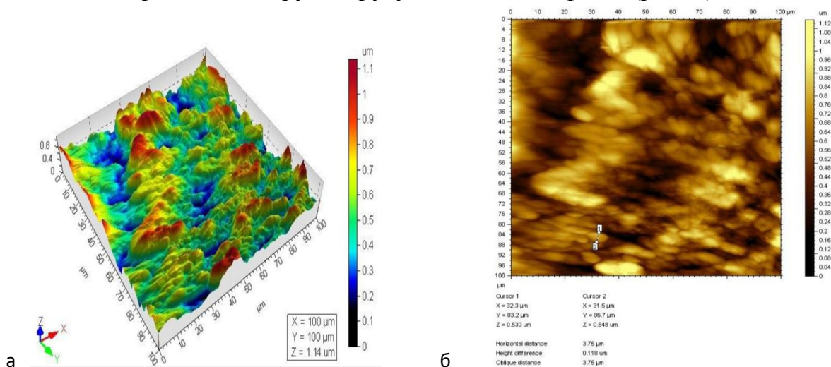
Рис. 5. Кадмий ацетат/ПП: а) – трехмерное изображение б) – двумерное изображение.
