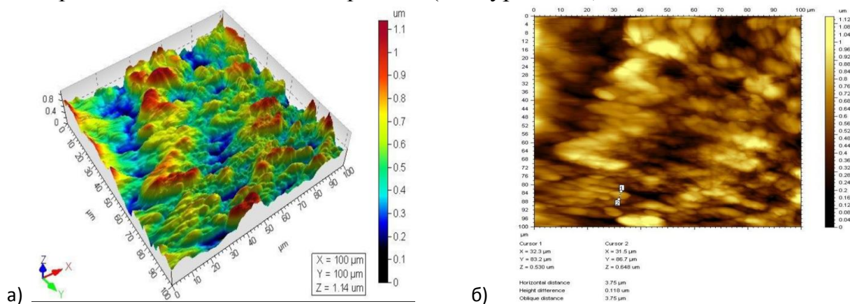
5-расм. Кадмий ацетат/ПП: а) уч ўлчамли расм б) икки ўлчамли расм.
