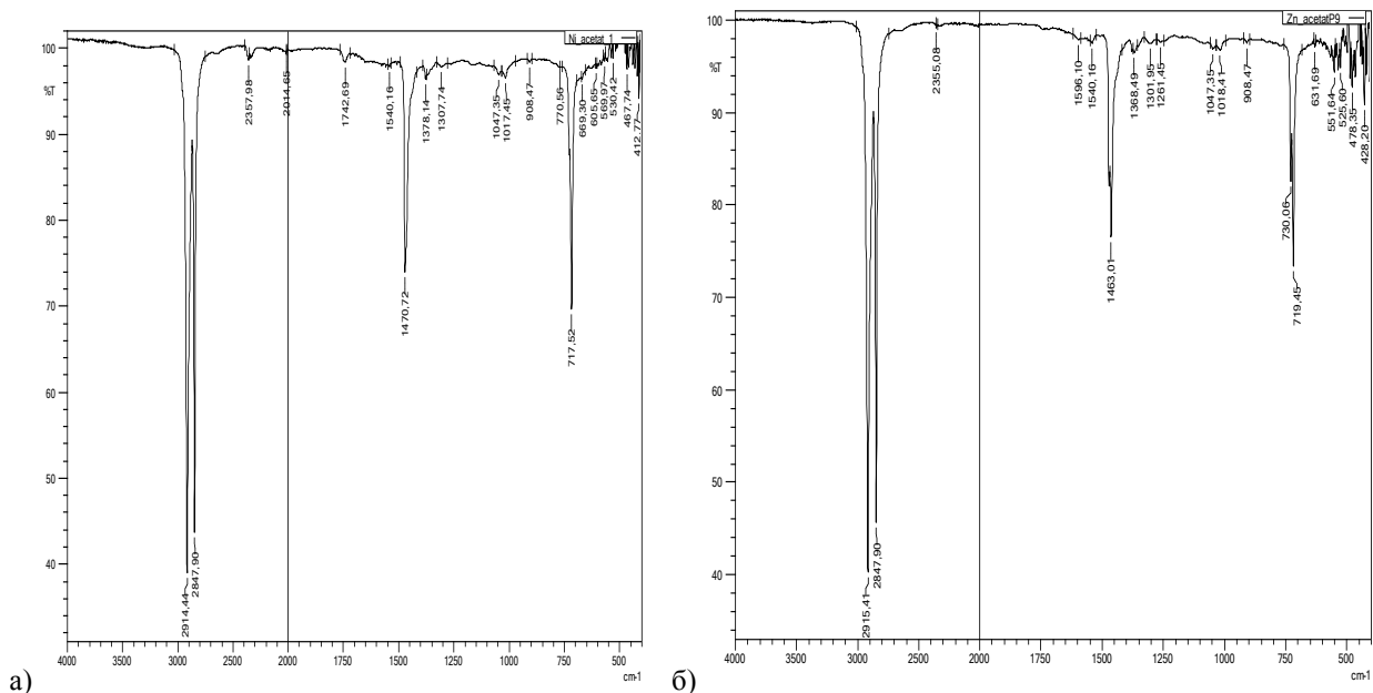
Рис. 7. а) ПЭ+Ni ацетат 3%, б) ПЭ+Zn ацетат 3%. Вид в ИК-спектре.
