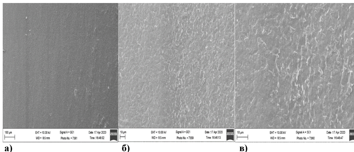
4-расм. а) ПП/Zn ацетат 3,0 % - 100 марта, б) ПП/Zn ацетат 3,0 % - 500 марта, в) ПП/Zn ацетат 3,0 % - 1000 марта катталаштирилган СЭМ микроскопида ўрганилган наъмуналар.
