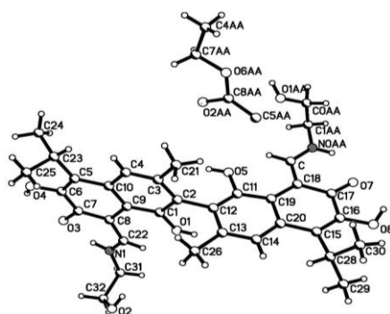
Рис. 5. Конформация молекул и нумерация атомов в структуре клатрата госсиполиден-ди(моноэтанолamina) с этилацетатом
