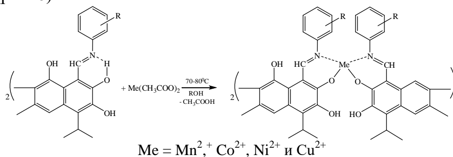
Рис. 6. Схема синтеза металлокомплексов оснований Шиффа
