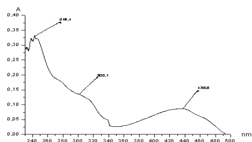
Рис. 2. УФ спектр госсиполиден-ди(2-амино-4,6-диметилпиридина)
