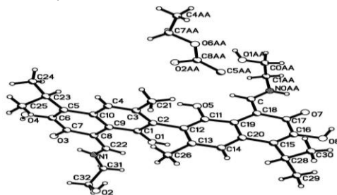
5-расм. Госсиполиден-ди(моноэтанолламин)нинг этилацетат билан клатрат тузилишидаги молекулаларнинг конформацияси ва атомларнинг номерацисы
