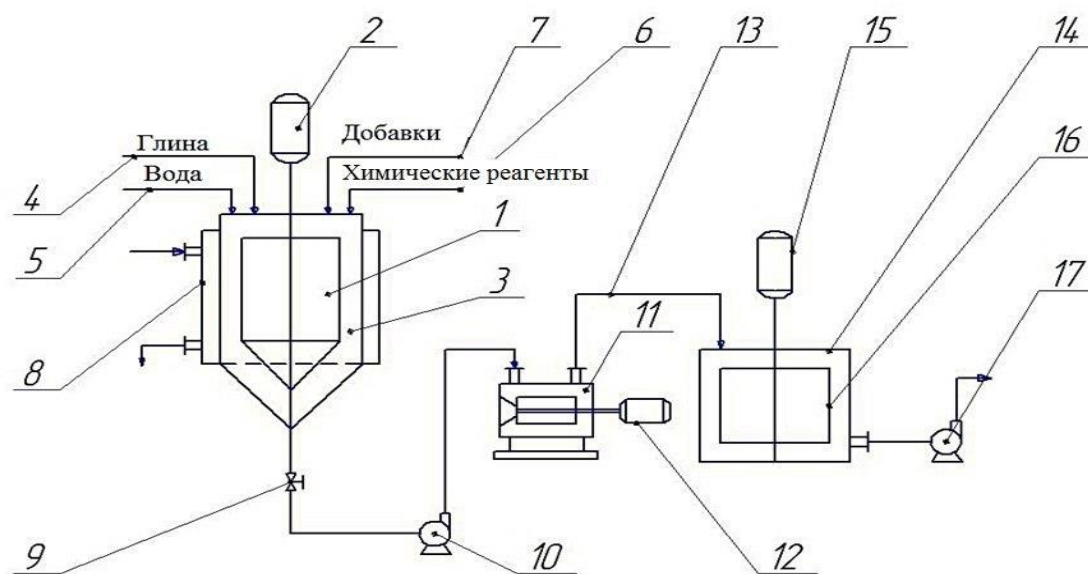
1-реактор-смеситель; 2, 15-двигатель; 3, 16-мешалка; 4-линия подачи глины; 5-линия подачи воды; 6-линия подачи хим.реагентов; 7-линия подачи добавок; 8-рубашка; 9- вентиль; 10, 17-насос; 11-МХД; 12-двигатель; 13-линия подачи готового раствора; 14- сборник.
