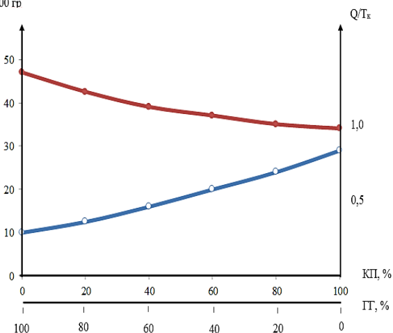
2 расм. Бурғилаш эритмаси композициясида карбонатли палигорскит ва гидрослюдали гилнинг миқдорига боғлиқ равишда катионли алмашинуви йиғиндиси (-○-) ва тузга чидамлик коэффициенти қийматларининг ўзгариши.
