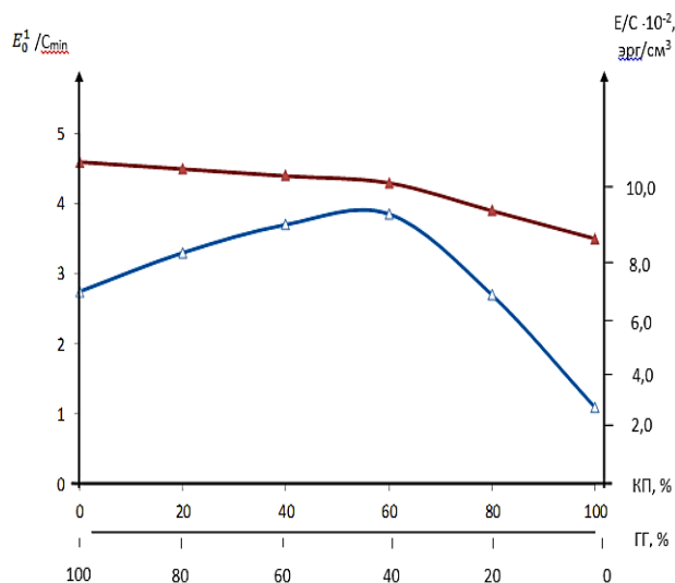
Рис. 3. Изменение значений \epsilon^1_0/C_{min} (-△-) и удельной энергии связи (-▲-) в зависимости от содержания карбонатного палыгорскита и гидрослюдистой глины в композиции бурового раствора.
