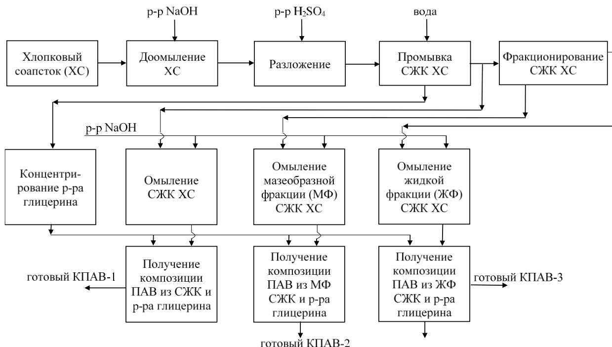
Рис. 1. Блок-схема получения композиции ПАВ на основе раствора концентрированного глицерина и СЖК XC и их фракции
