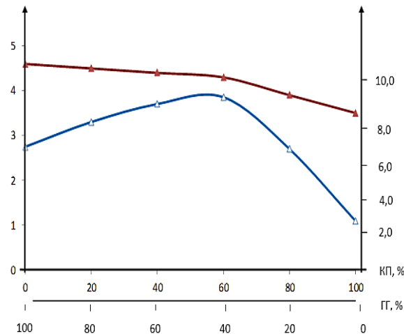
3 расм. Бурғилаш эритмаси композициясида карбонатли палигорскит ва гидрослюдали гилнинг миқдорига боғлиқ равишда \epsilon_0^1 / C_{min} (-Δ-) ва боғланишнинг солиштирма энергияси қийматларининг ўзгариши.
