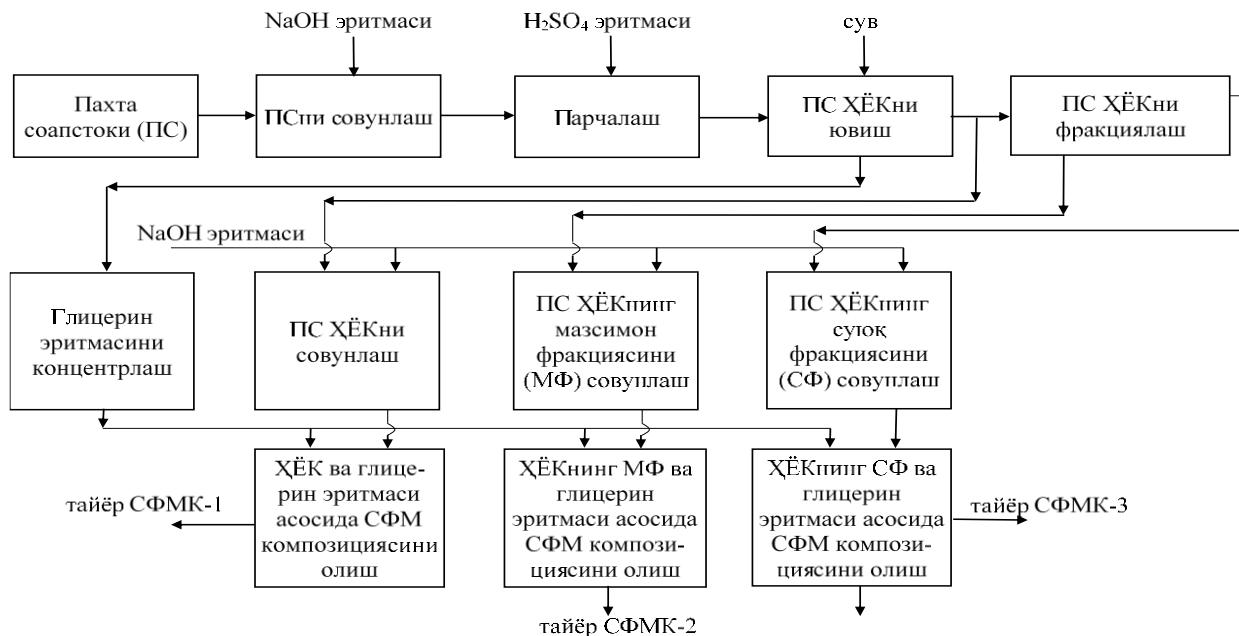
1-расм. ПС ХЁК ва унинг фракцияси ҳамда концентрланган глицерин эритмаси асосида СФМ композициясини олиш блок-схемаси
