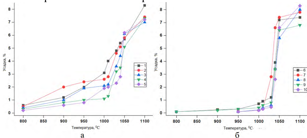
Рис. 9. Изменение усадки образцов двойных систем «щелочноземельный бентонит – барханный песок» при уменьшении содержания бентонита с 100 до 60 масс.% (а) и с 50 до 10 масс.% (б) с увеличением температуры их обжига
