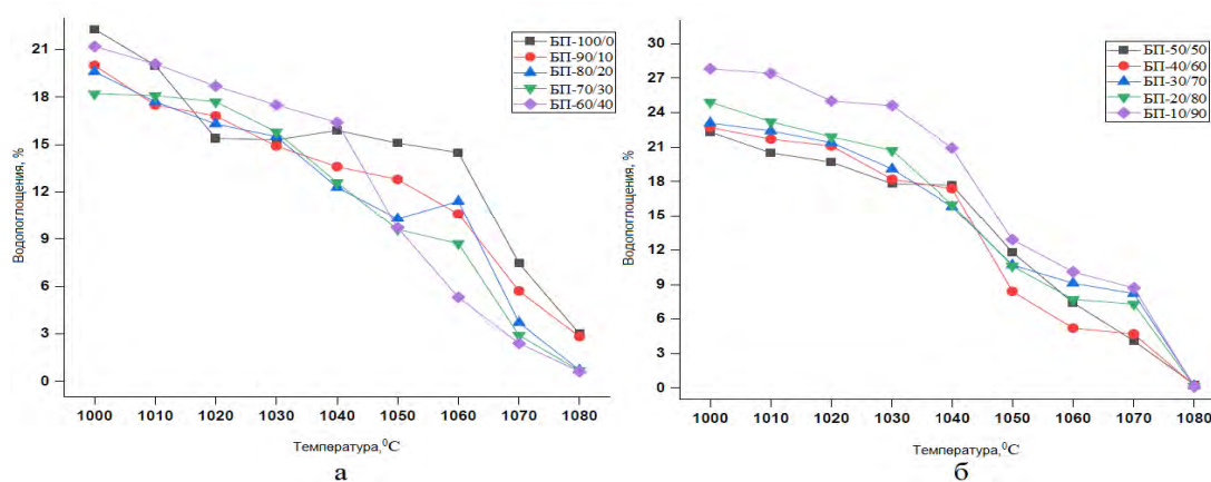
Рис.7. Зависимость изменения водопоглощения образцов из композиций БП-100/0 – БП-10/90 от температуры их обжига (а, б)
