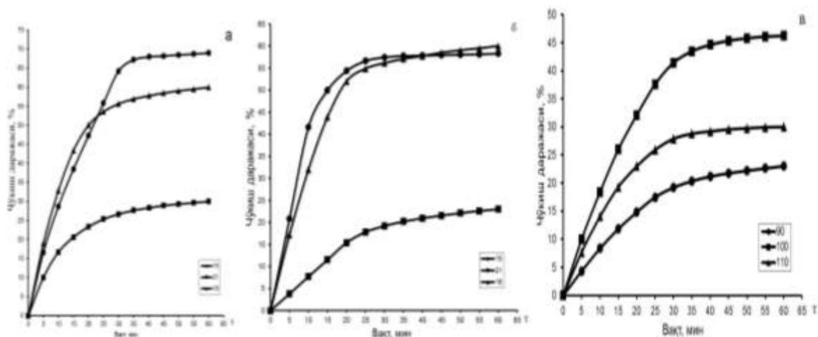
1-расм. Оҳак сути концентрациясига ва меъёрига боғлиқ равишда калий карбонат конверсияси натижасида ҳосил бўлган суспензиянинг тиниш тезлиги: а) K_2CO_3 - 40%, меъёр - 90%; б) K_2CO_3 50%, меъёр - 90%; в) K_2CO_3 - 50%, Ca(OH)_2 – 15%.
