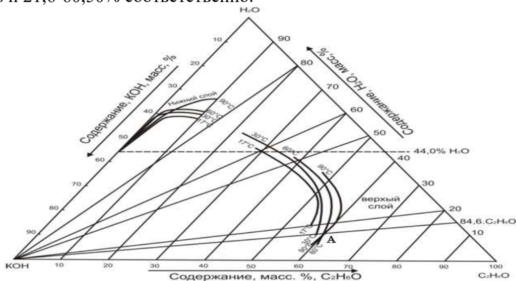
Рис. 3. Политерма системы C_2H_5OH-KOH-H_2O .
