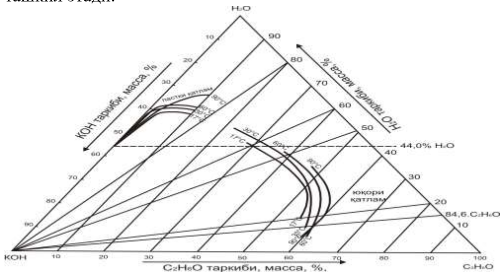
3-расм. \text{C}_2\text{H}_5\text{OH}-\text{KOH}-\text{H}_2\text{O} системаси политемик
