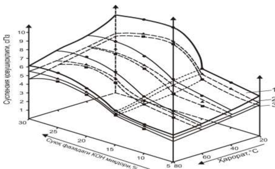
2-расм. Поташни оҳакли сутда конверсияси натижасида ҳосил бўлган кальций карбонат ва калий гидроксид тутган суспензиянинг зичлигини(а) ва қовушқоқлигини (в) аниқлаш учун номограмма
