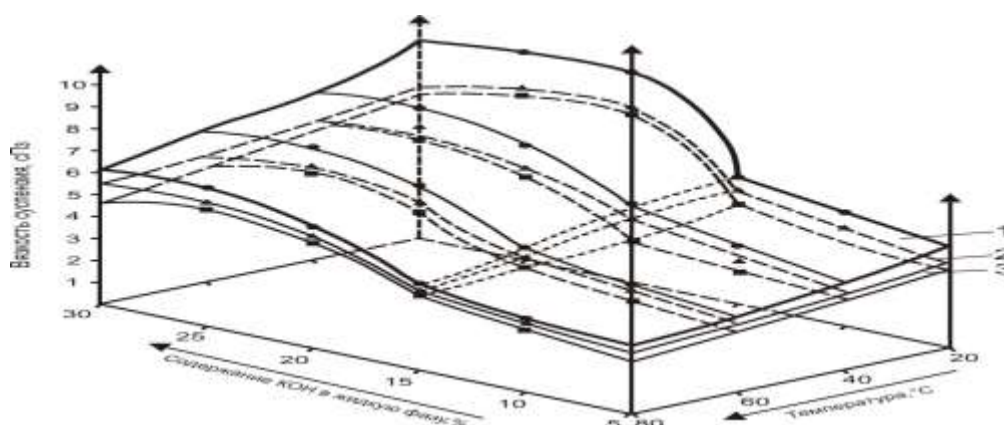
Рис. 2. Номограмма для определения плотности (а) и вязкости (в) суспензии, образующейся в результате конверсии поташа известковым молоком.
