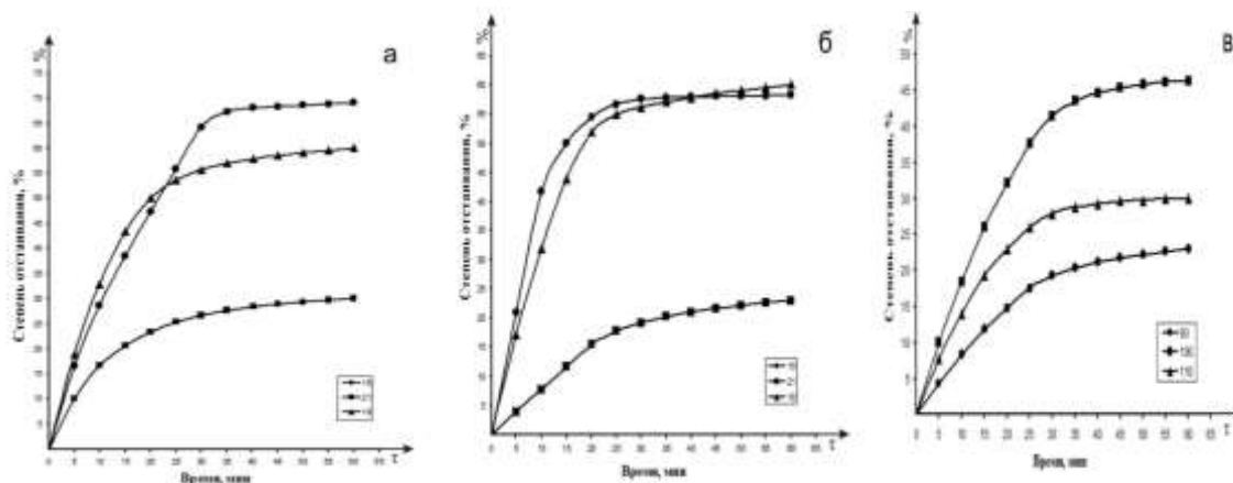
Рис. 1. Кинетика разрушения суспензии, образовавшейся в результате превращения извести в карбонат калия, составляет: а) K_2CO_3 40%, норма 90%; б) K_2CO_3 50%, норма 90%; в) K_2CO_3 - 50%, Ca(OH)_2 - 15%.
